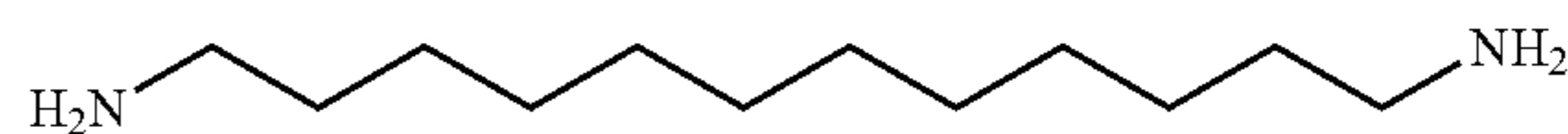
1, 12-dodecanediamine (DAD)
