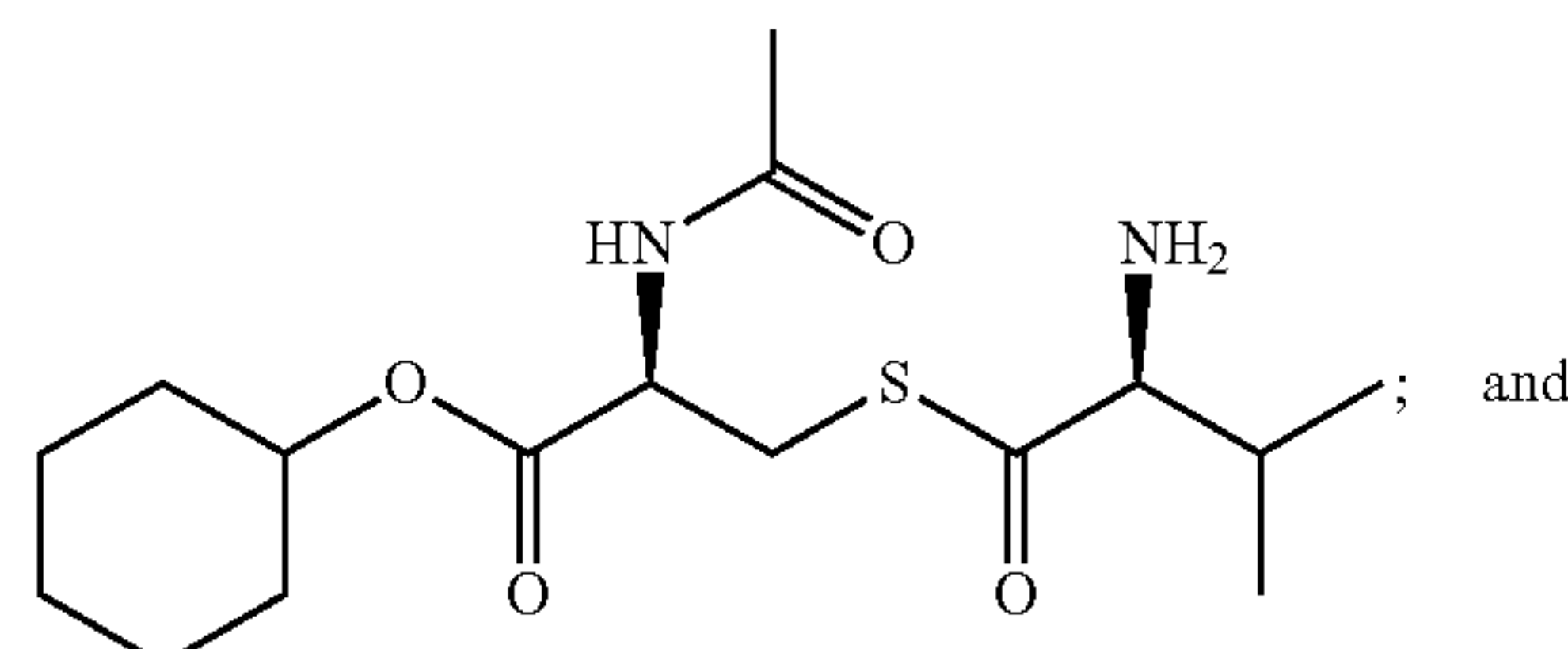
cyclohexyl (2R)-3-([(2S)-2-amino-3-methylbutanoyl]sulfanyl)-2-acetamidopropanoate
