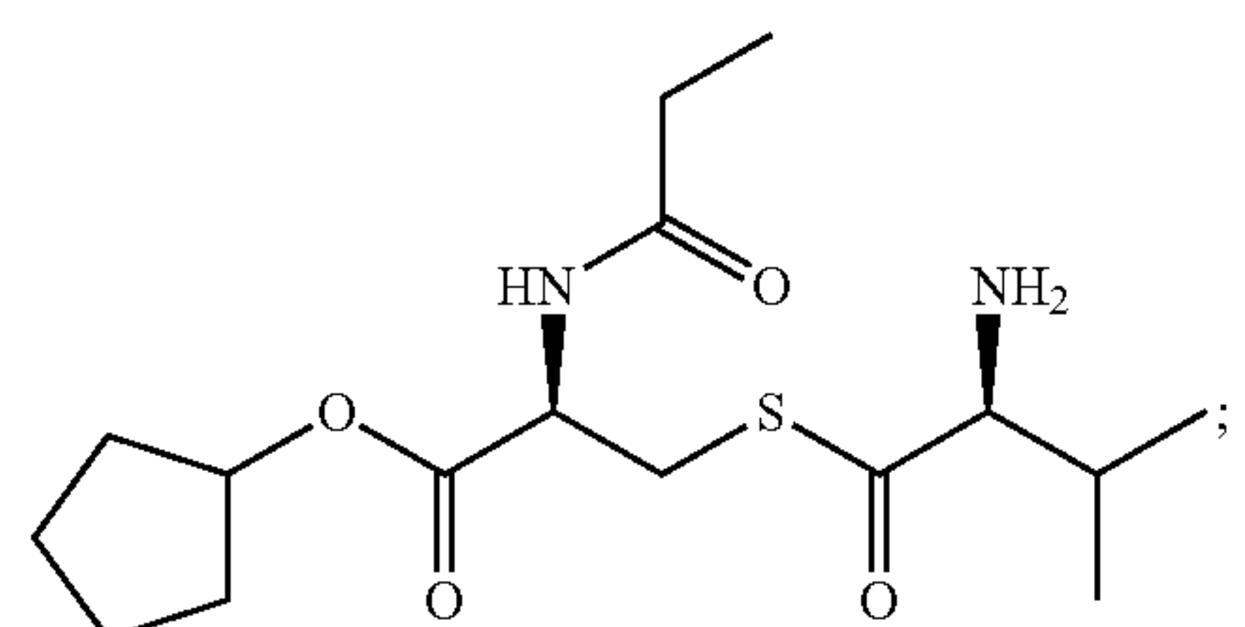
cyclopentyl (2R)-3-([(2S)-2-amino-3-methylbutanoyl]sulfanyl)-2-propanamidopropanoate
