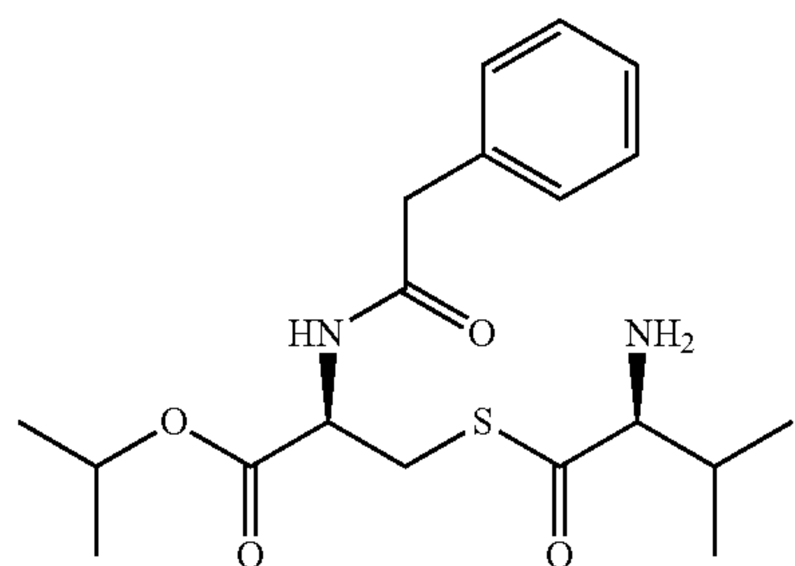
propan-2-yl (2R)-3-([(2S)-2-amino-3-methylbutanoyl]sulfanyl)-2-(phenylacetamido)propanoate
