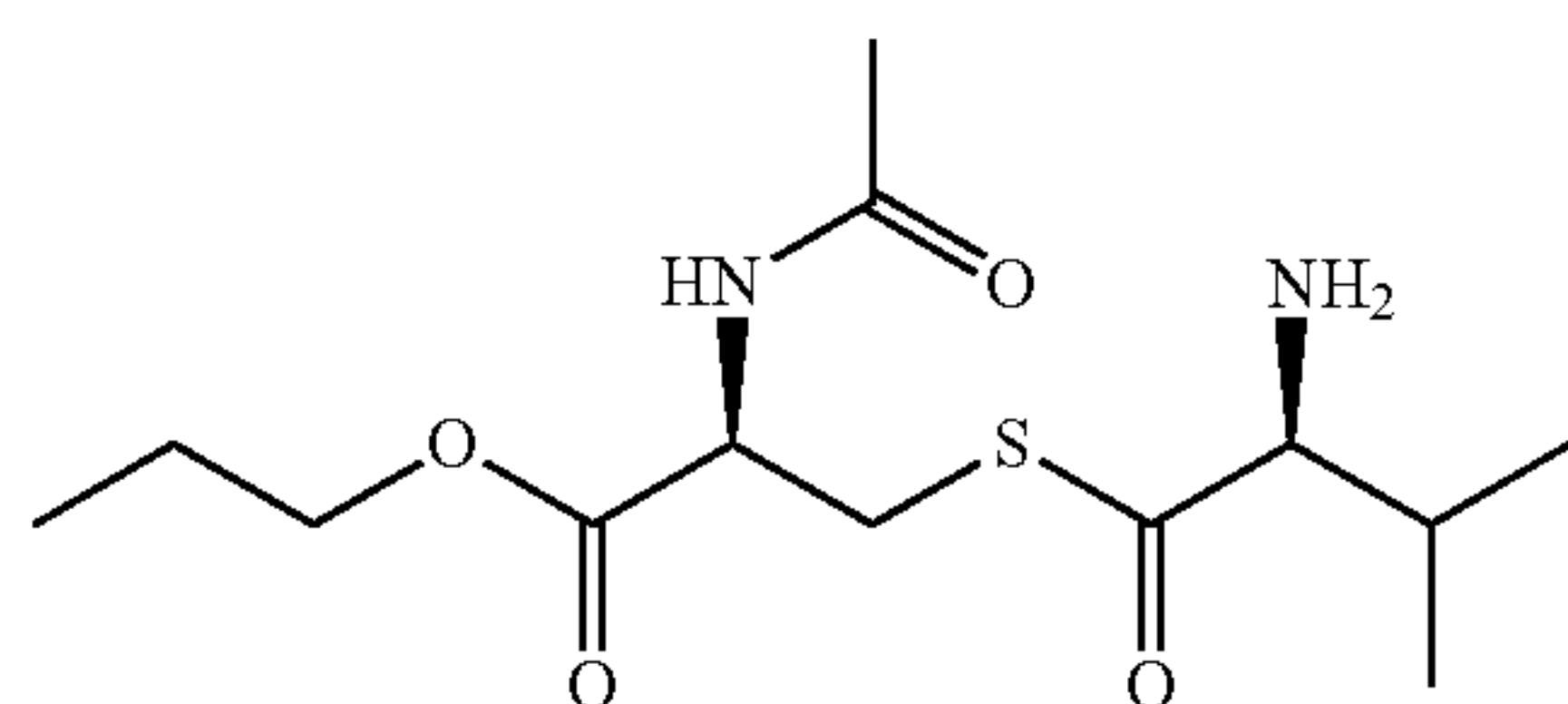
propyl (2R)-3-([(2S)-2-amino-3-methylbutanoyl]sulfanyl)-2-acetamidopropanoate
