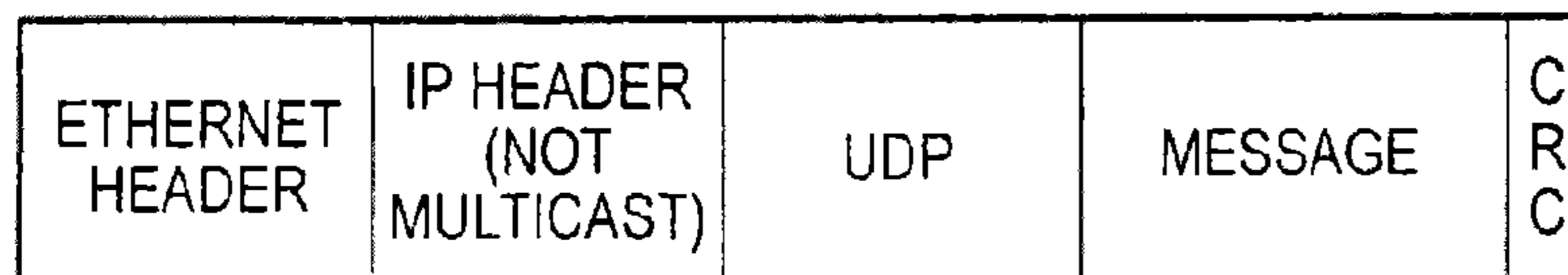
FIG. 3C
