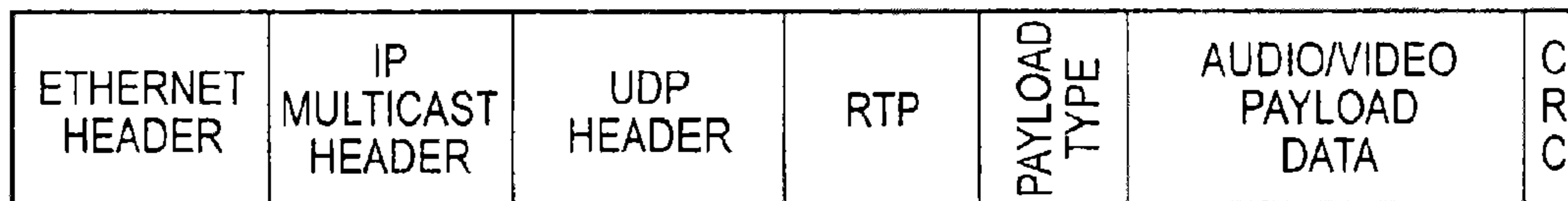
FIG. 3A
