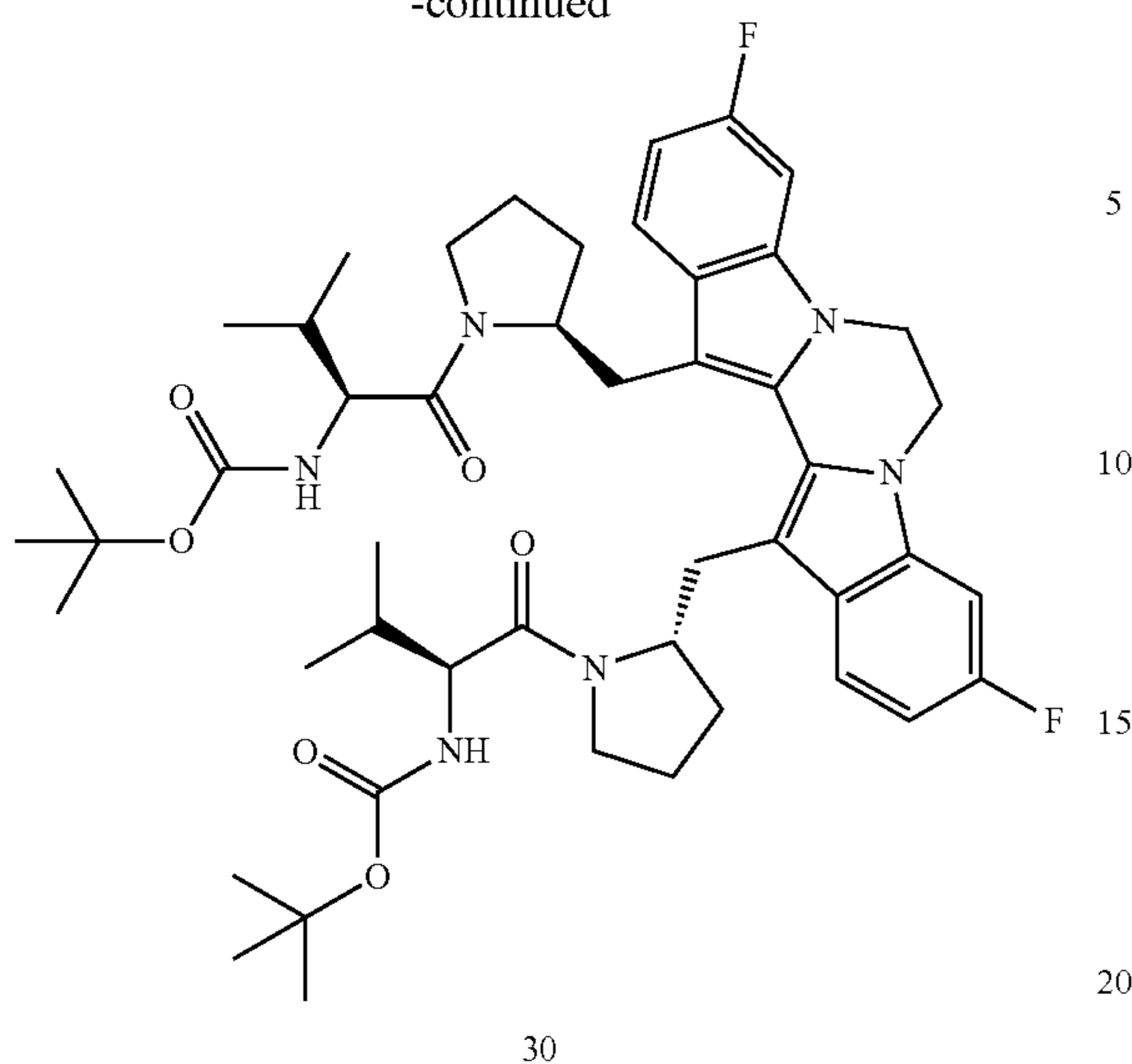
3,10-Difluoro-13,14-bis-pyrrolidin-2-ylmethyl-6,7-dihydro-pyrazino[1,2-a;4,3-a']diindole (29)
