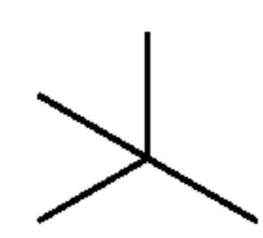
tert-butyl
