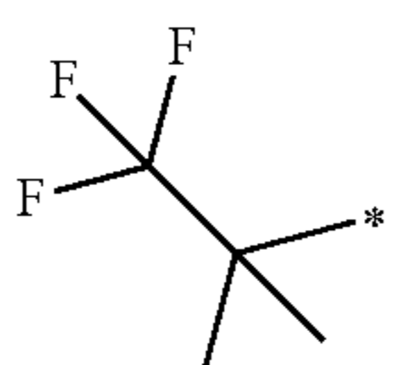
1,1,1-trifluoro-2-methylpropane-2-yl
