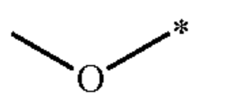
methoxy
