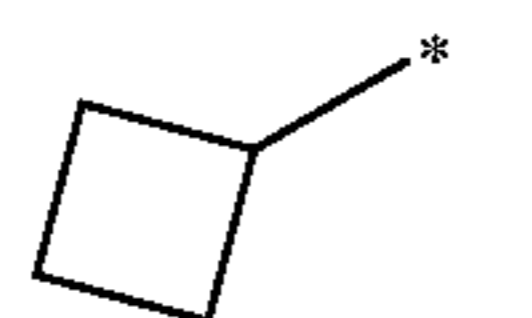
cyclobutyl
