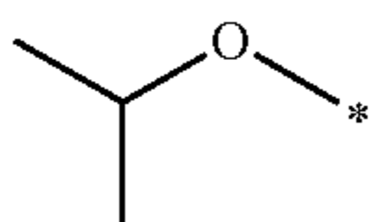
isopropoxy
