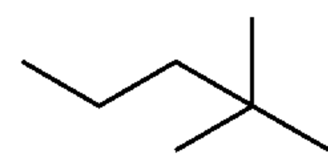
2-methylpentan-2-yl
