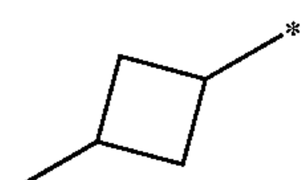
3-methylcyclobutyl
