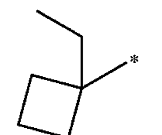
1-ethylcyclobutyl
