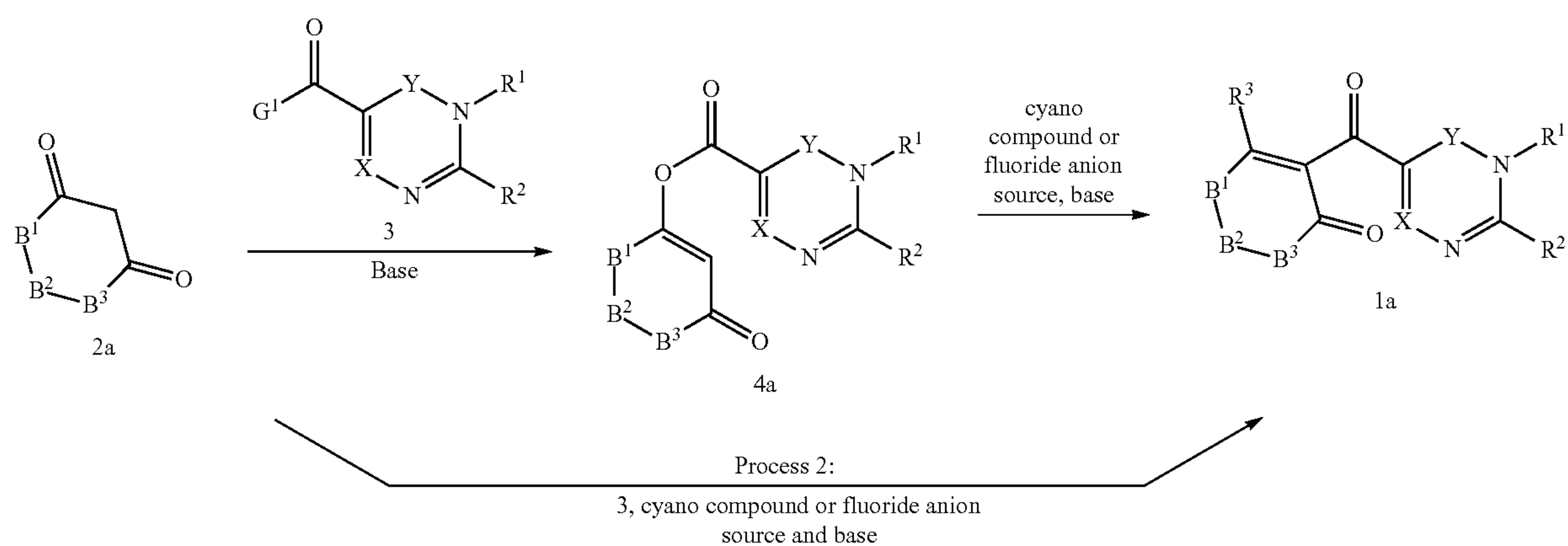
Scheme 1a
