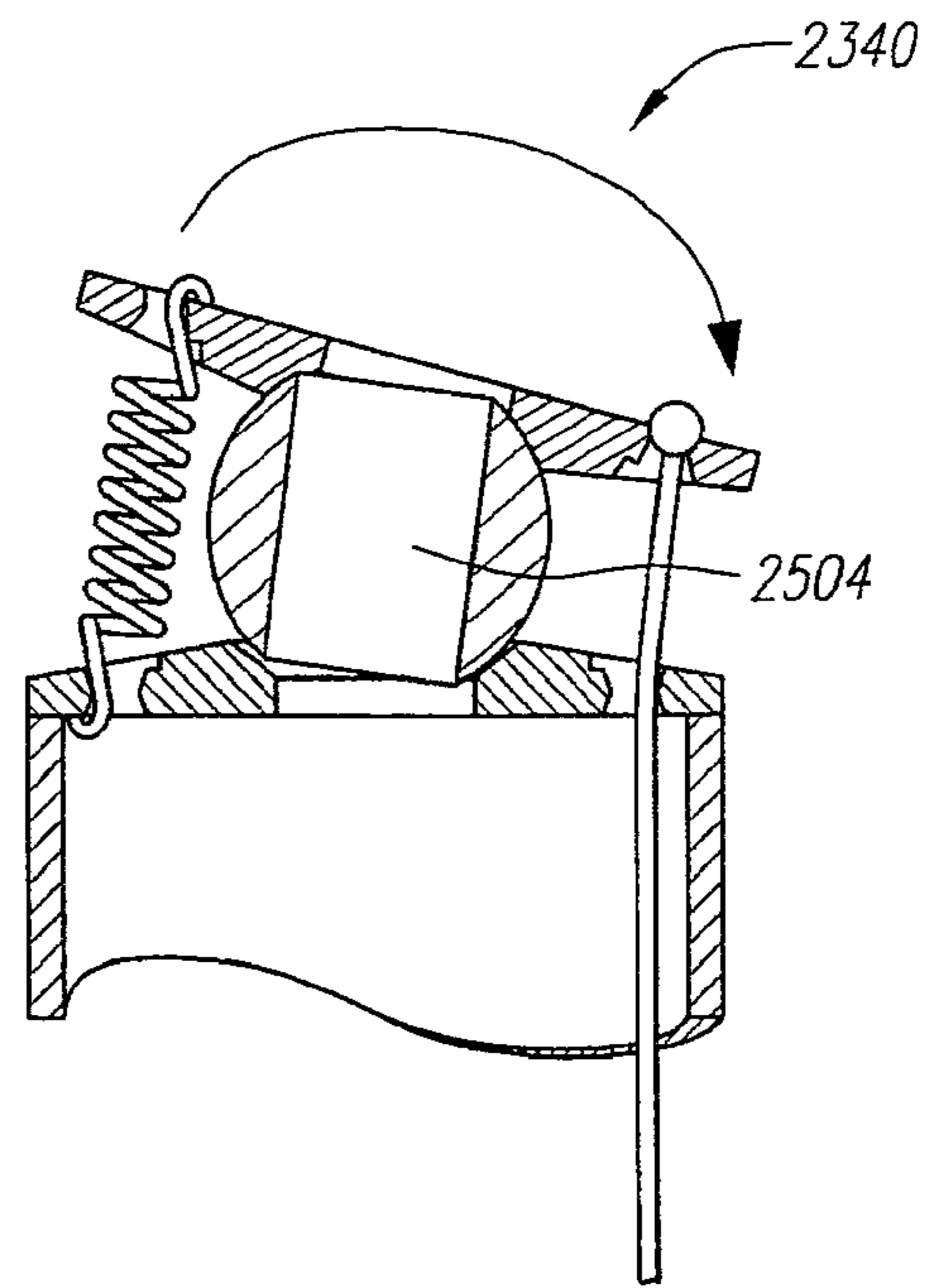
Fig 25F
