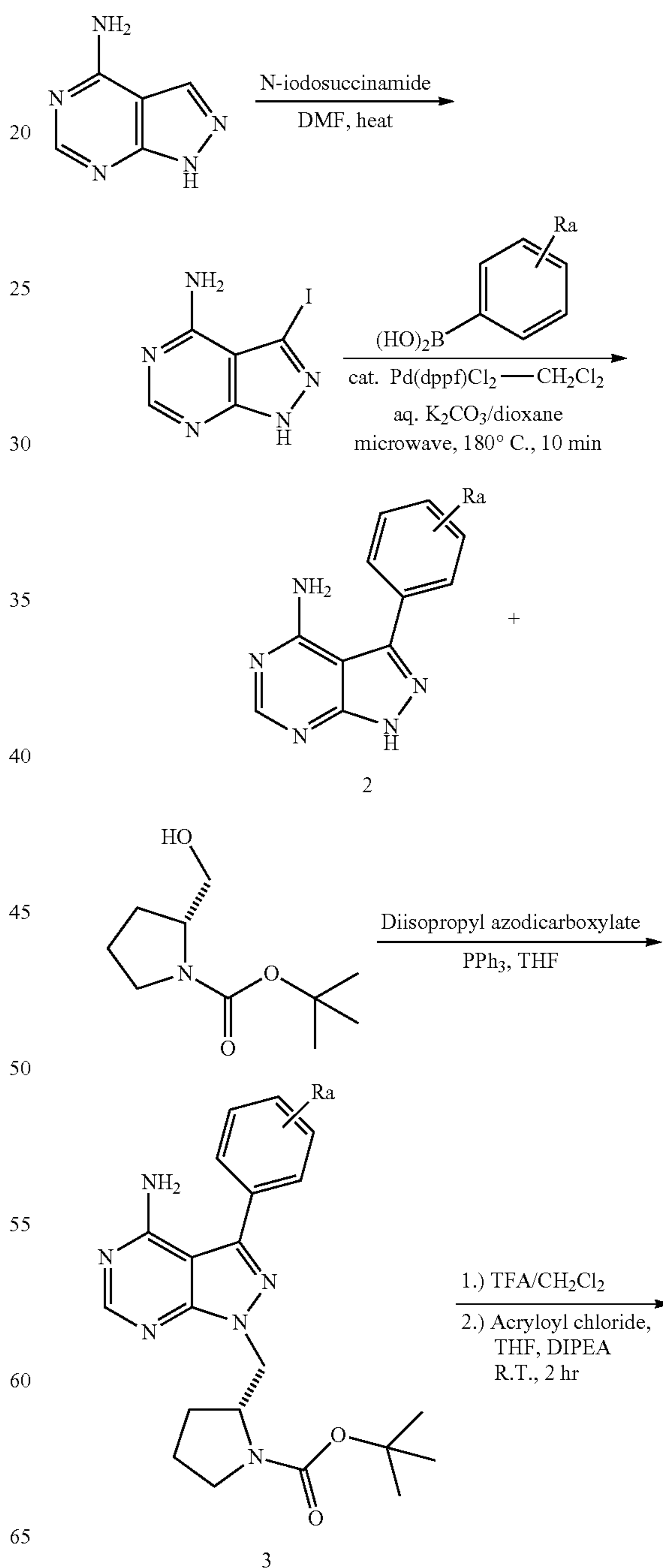
Scheme I.
