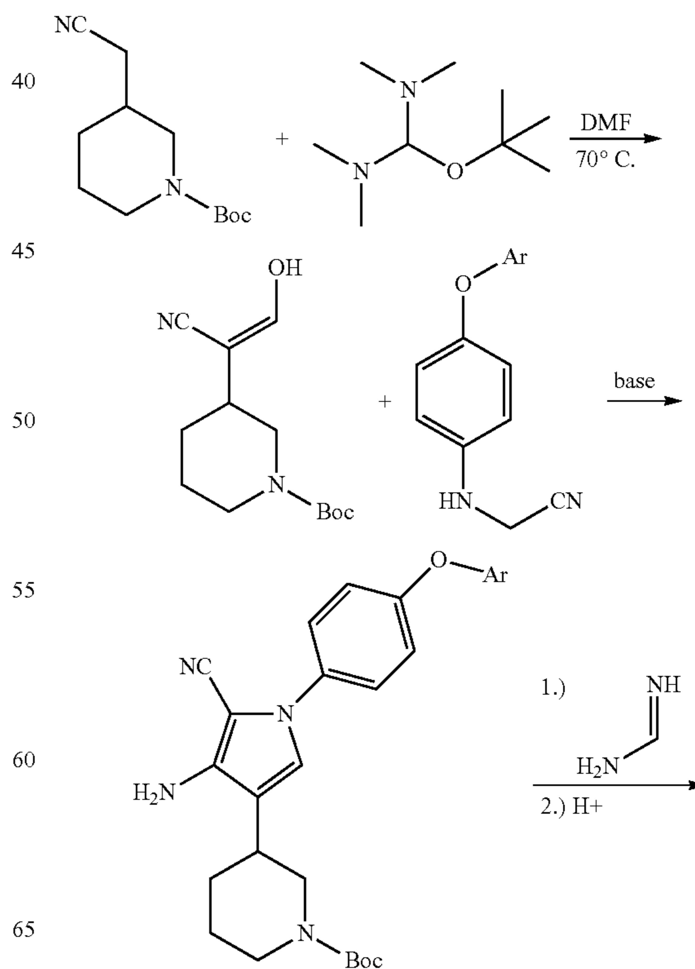
Scheme VI.
