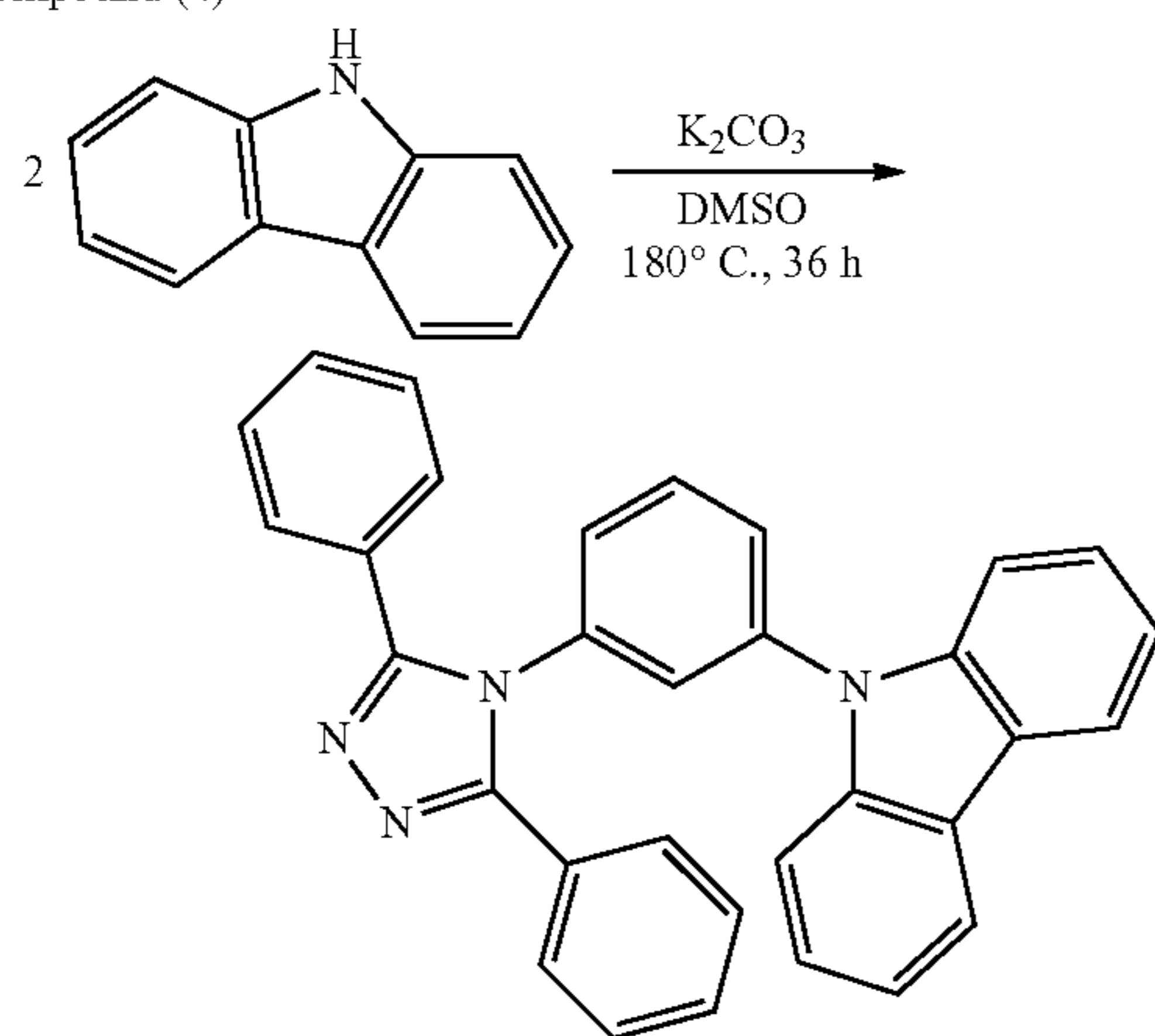
m-TAZCz
