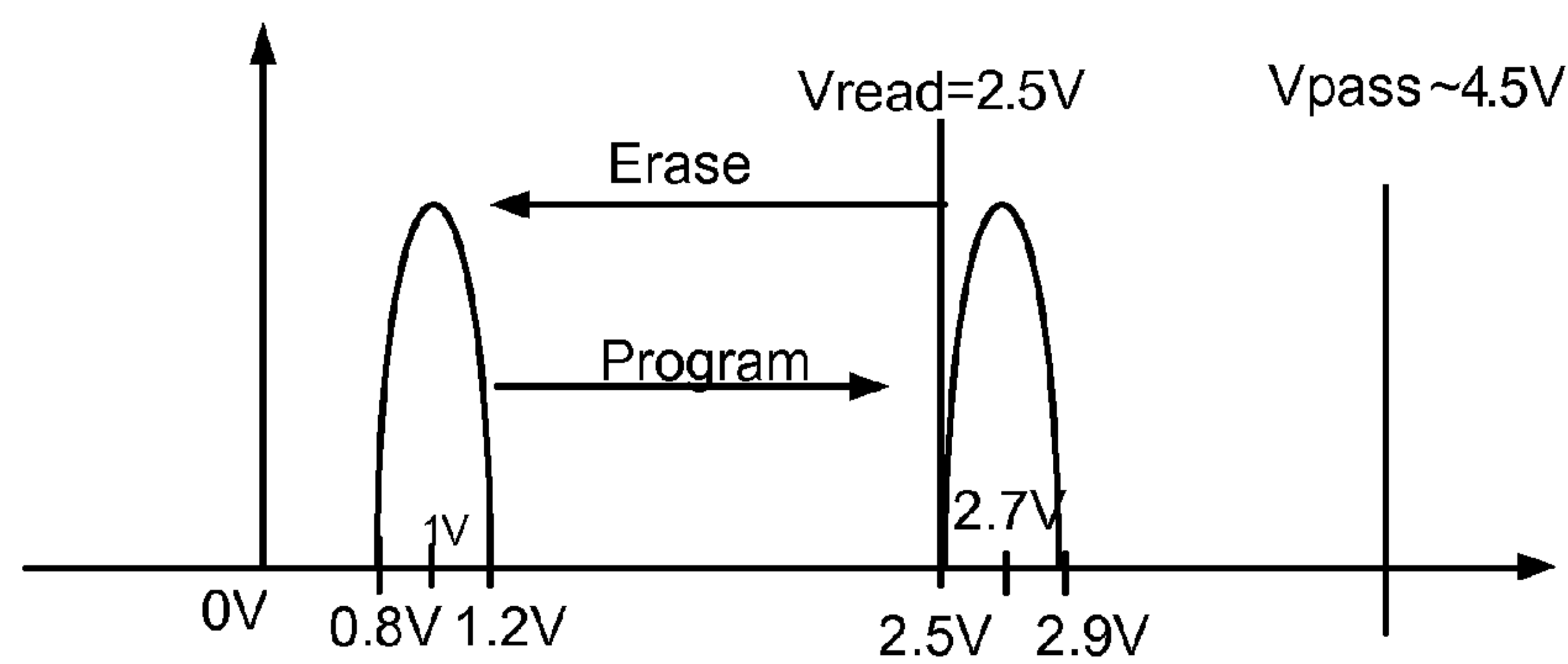
Fig. 12A
