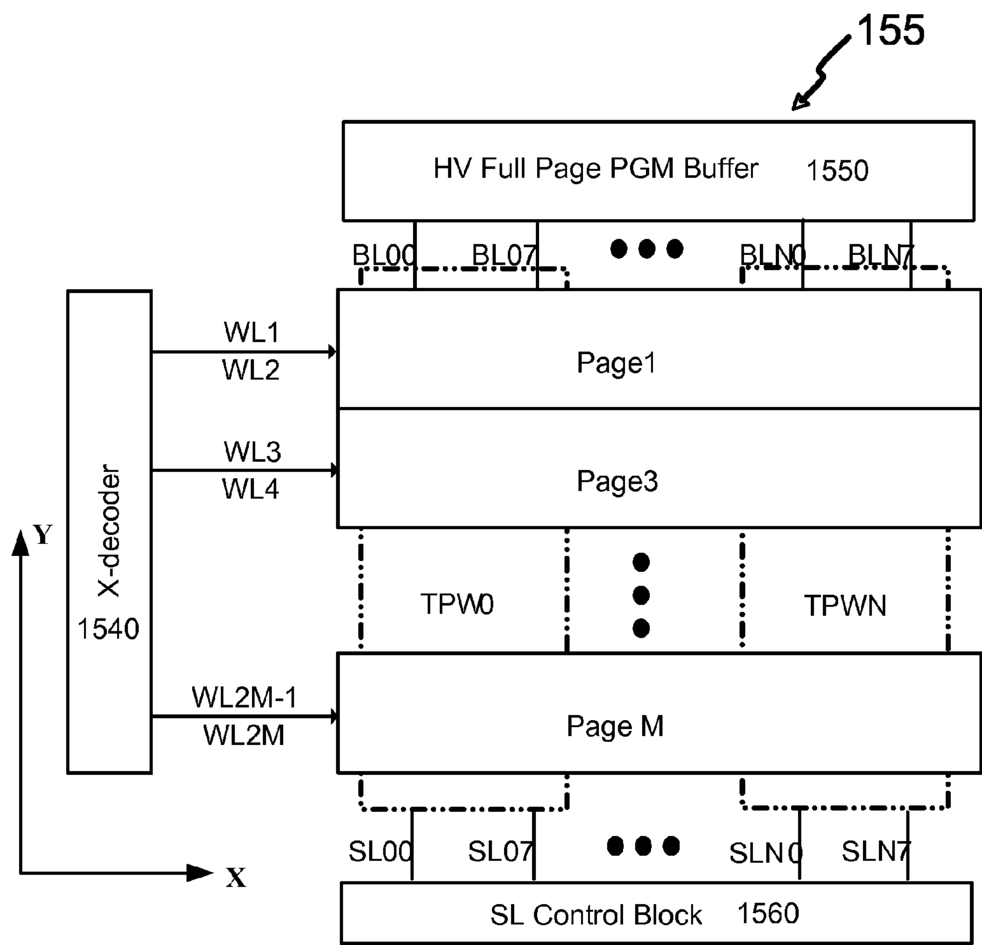
Fig. 11B
