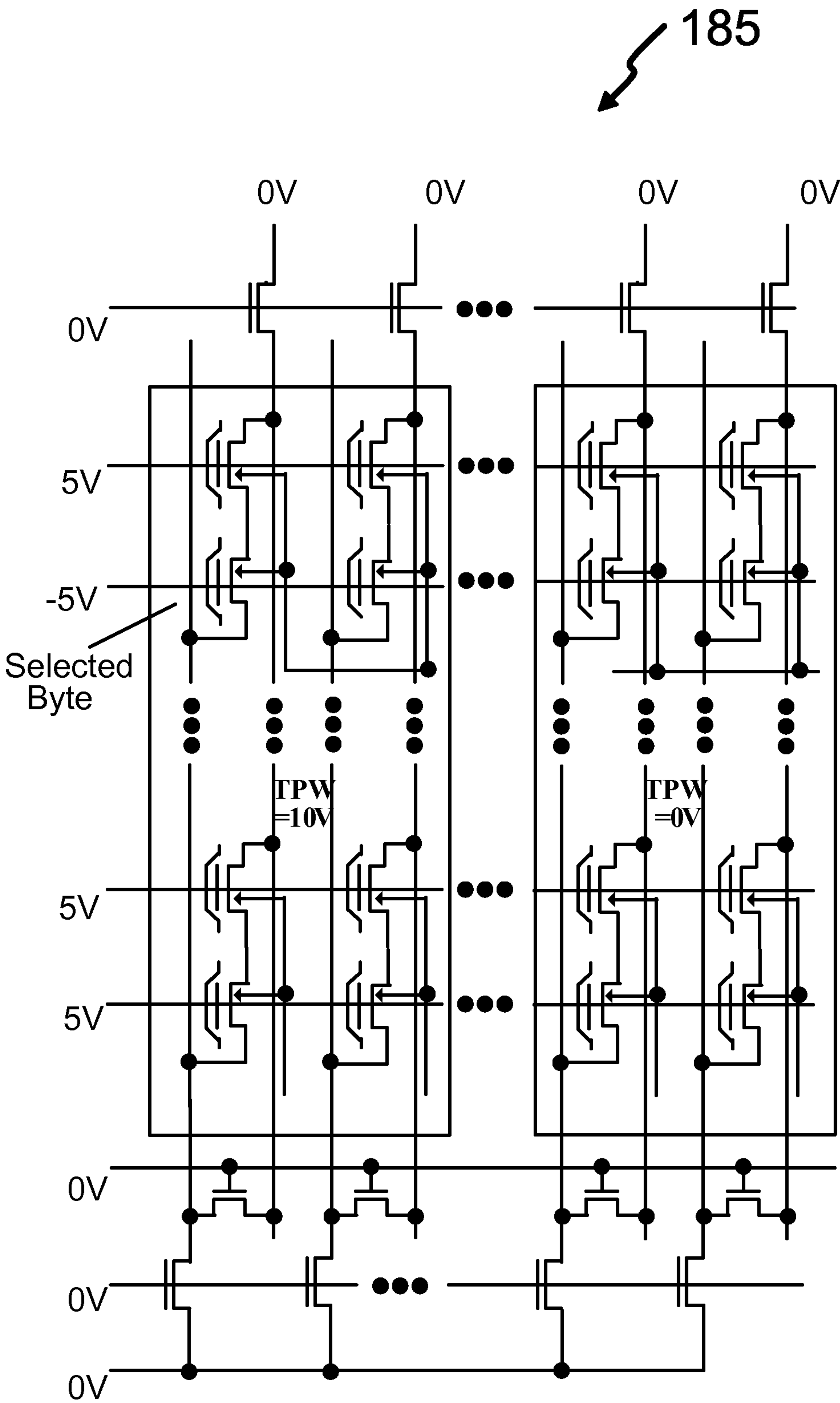
Fig. 14B
