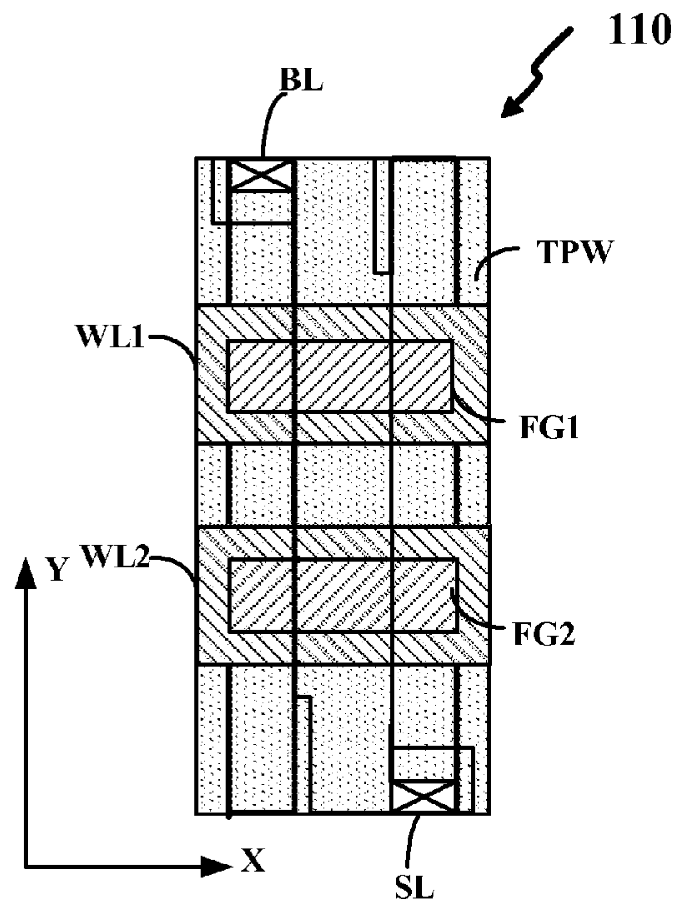
Fig. 9A
