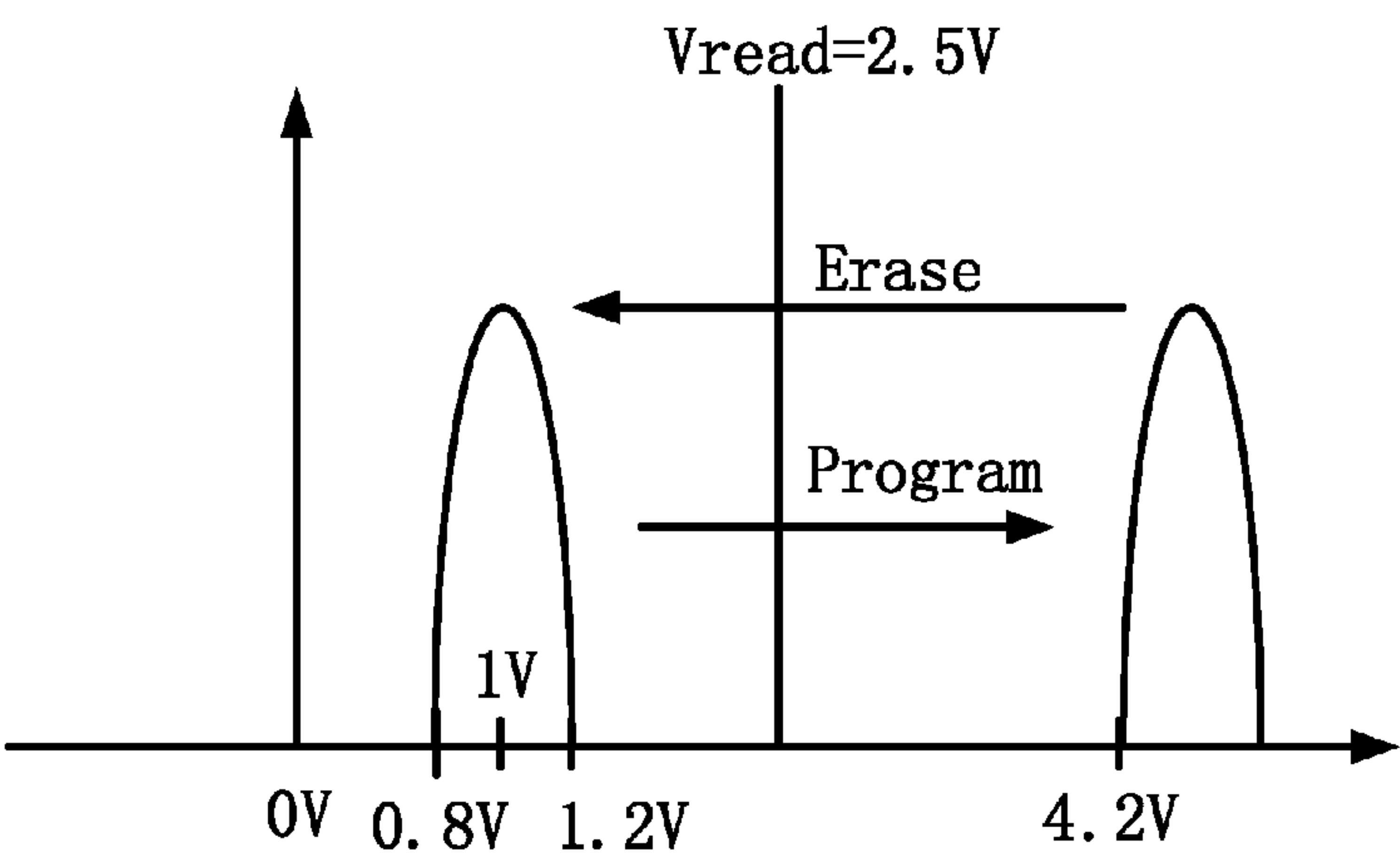
Fig. 6A
