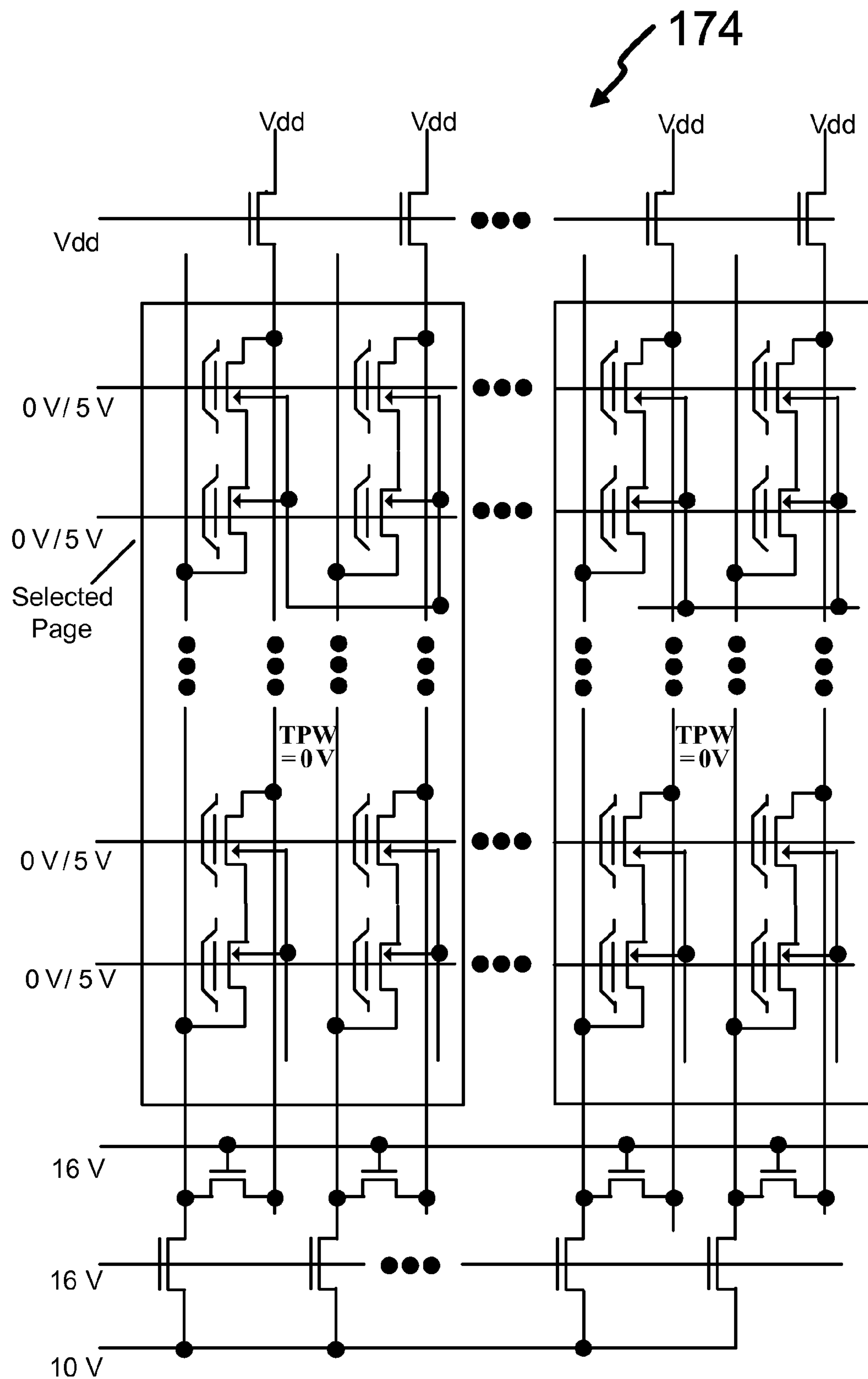
Fig. 13C
