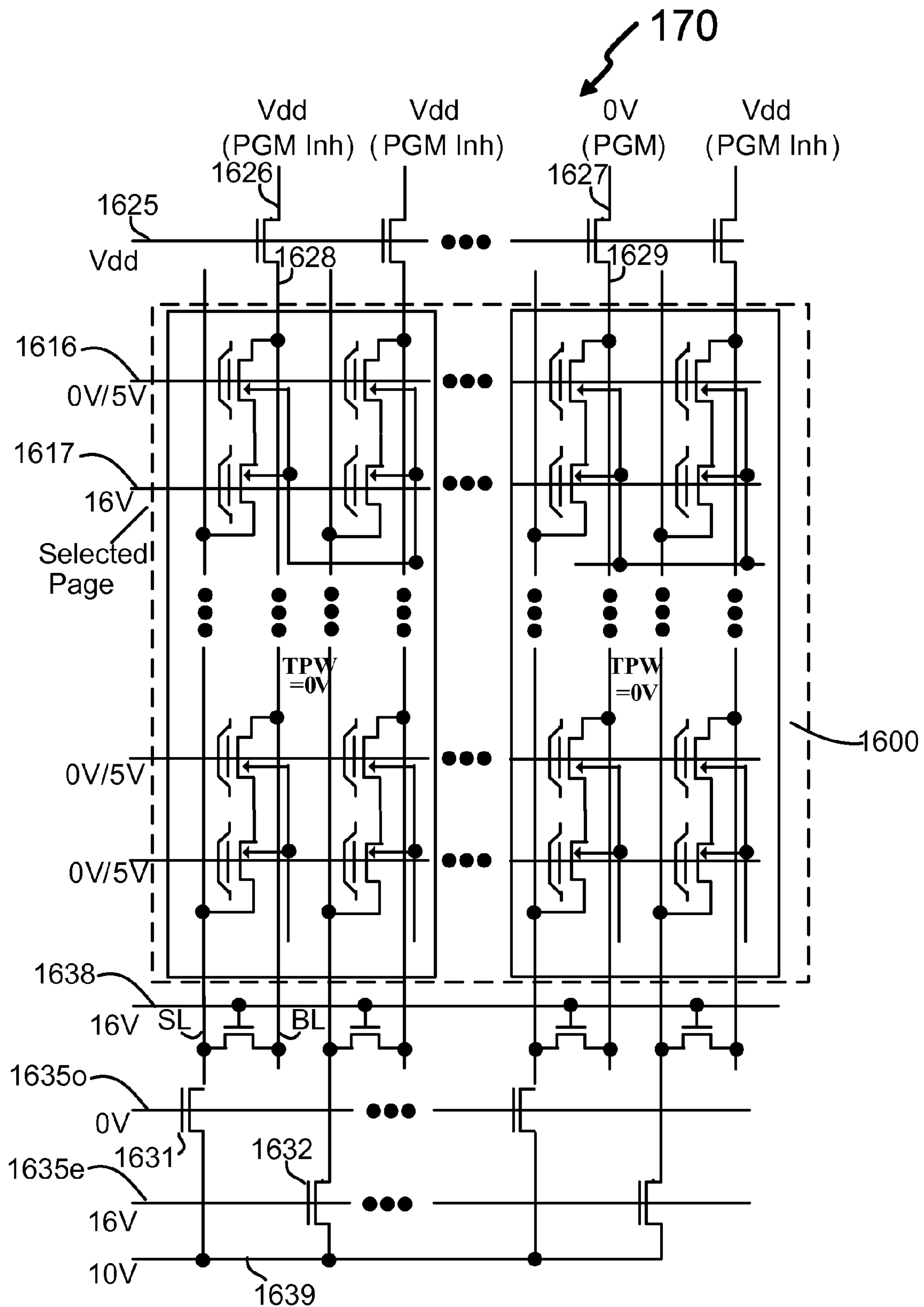
Fig. 13B
