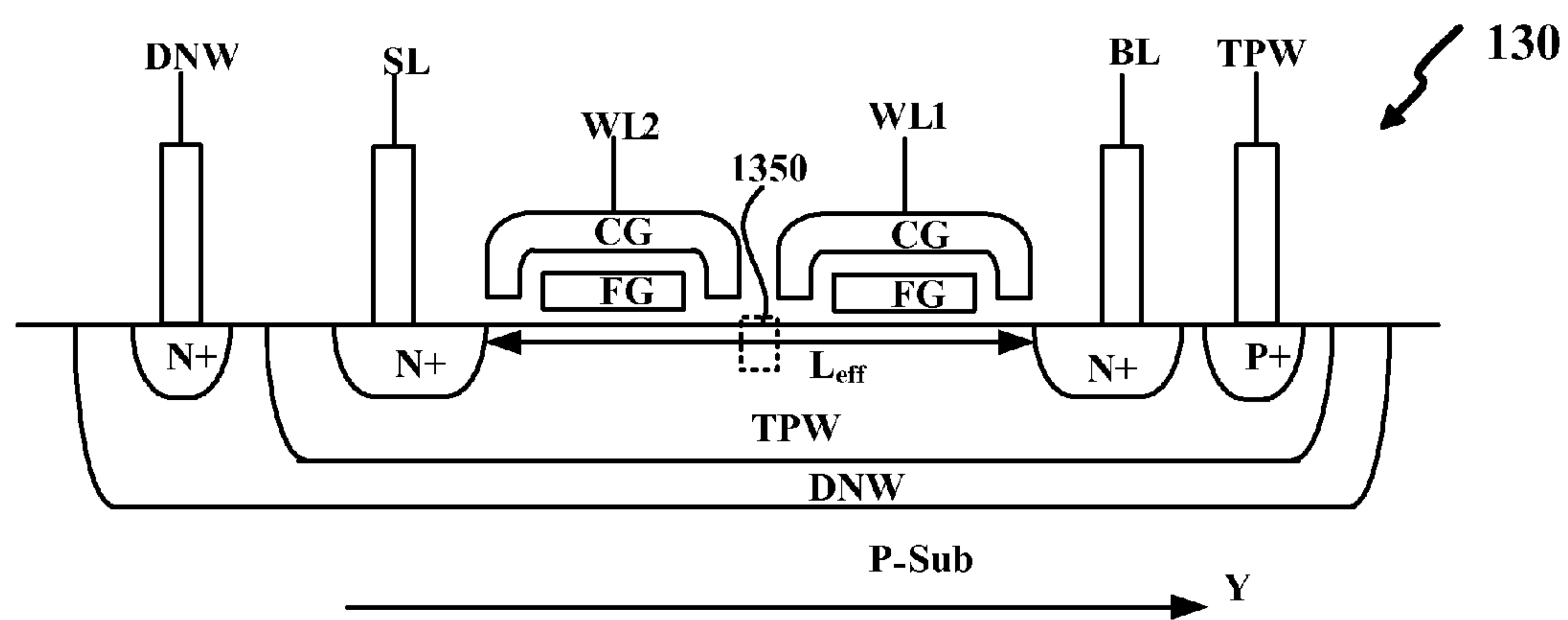
Fig. 9C
