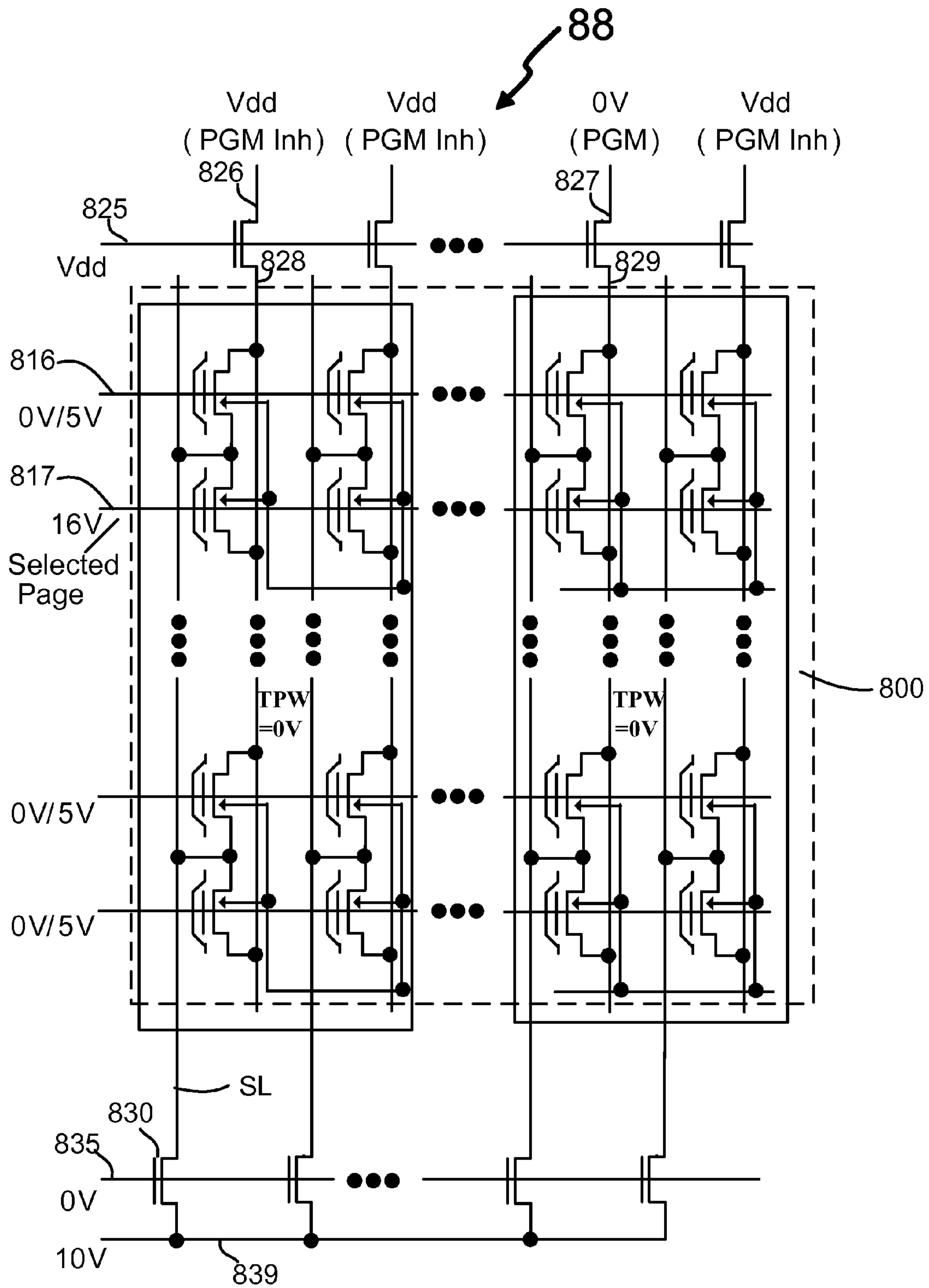
Fig. 7D
