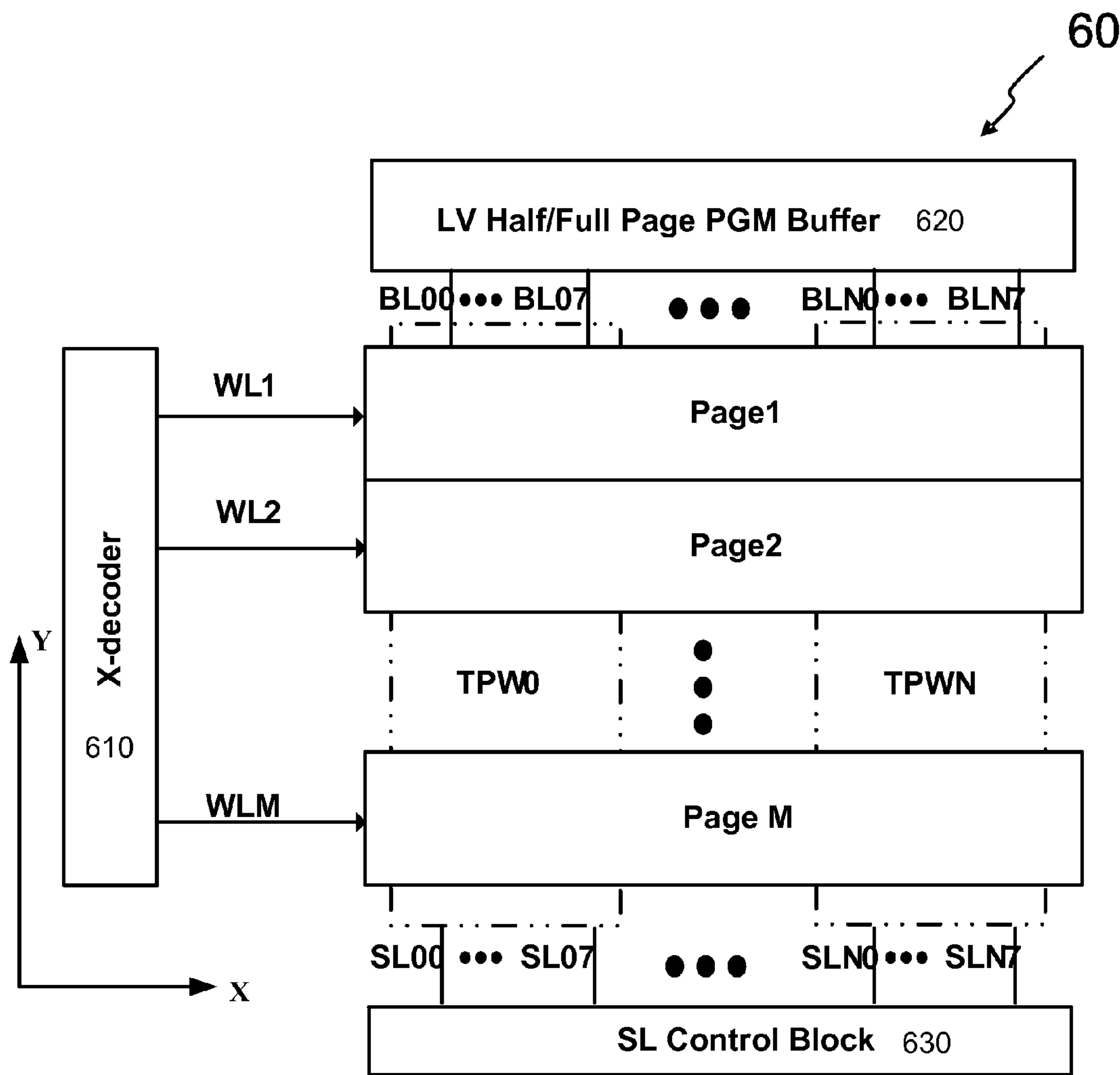
Fig. 5A
