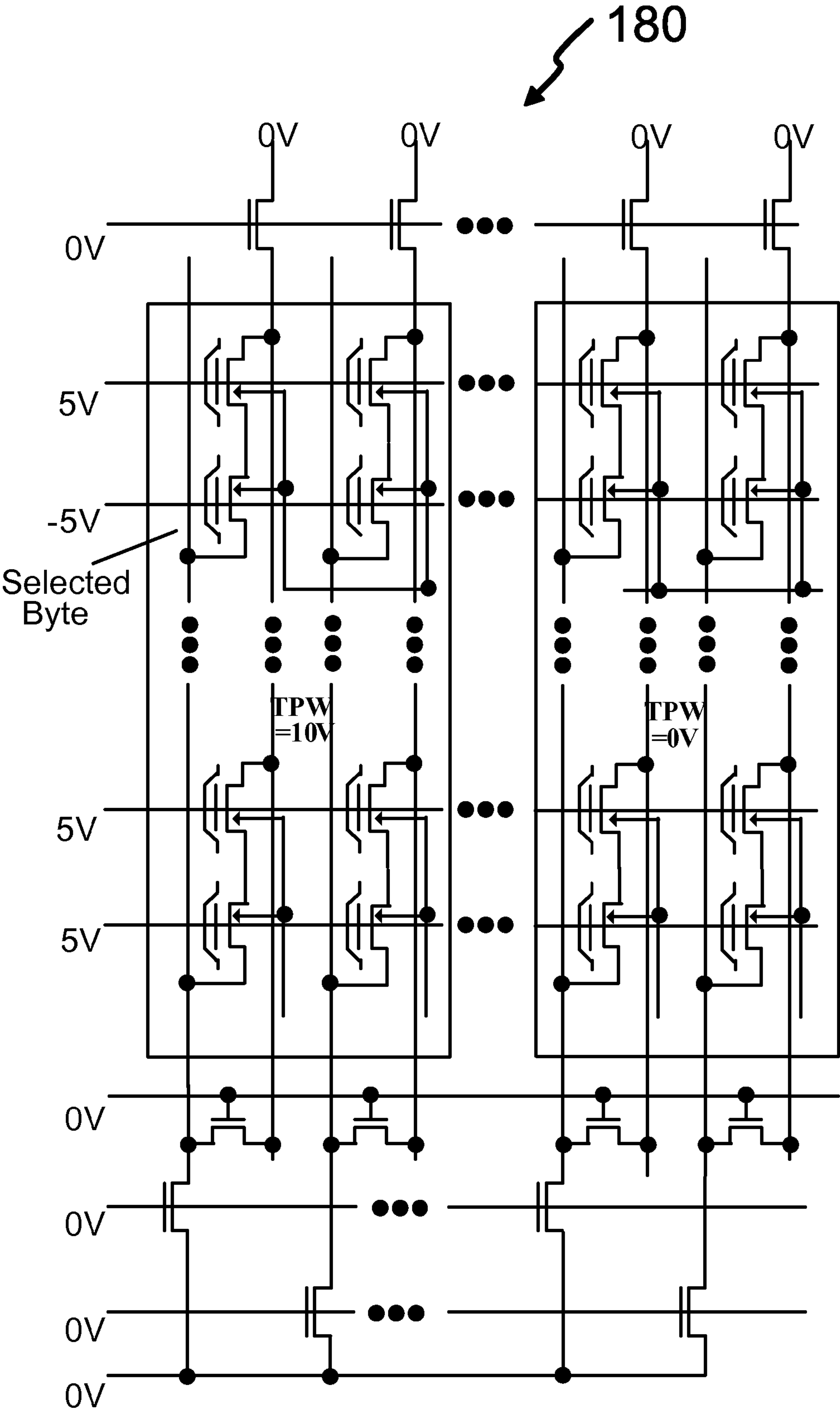
Fig. 14A
