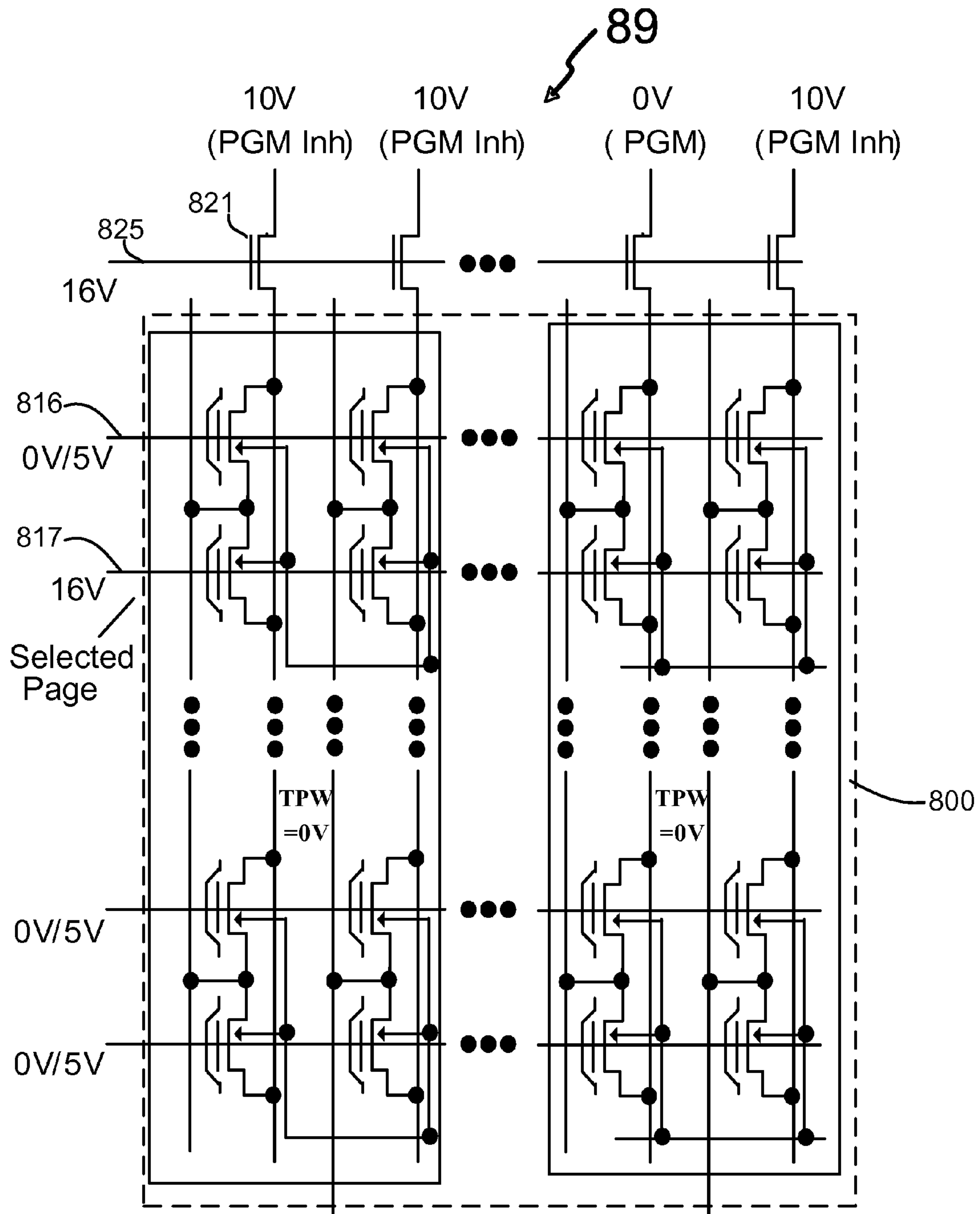
Fig. 7E
