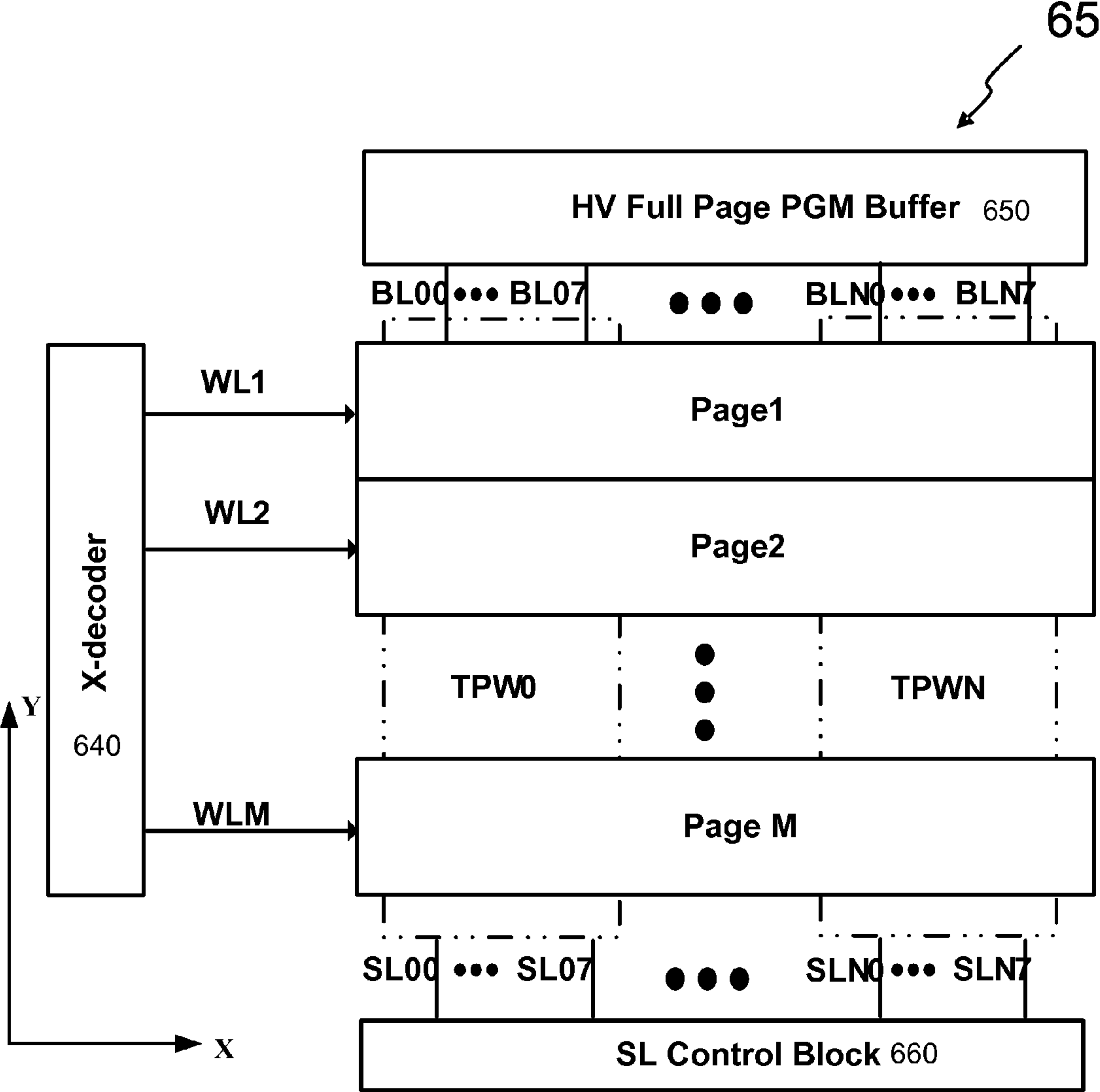
Fig. 5B
