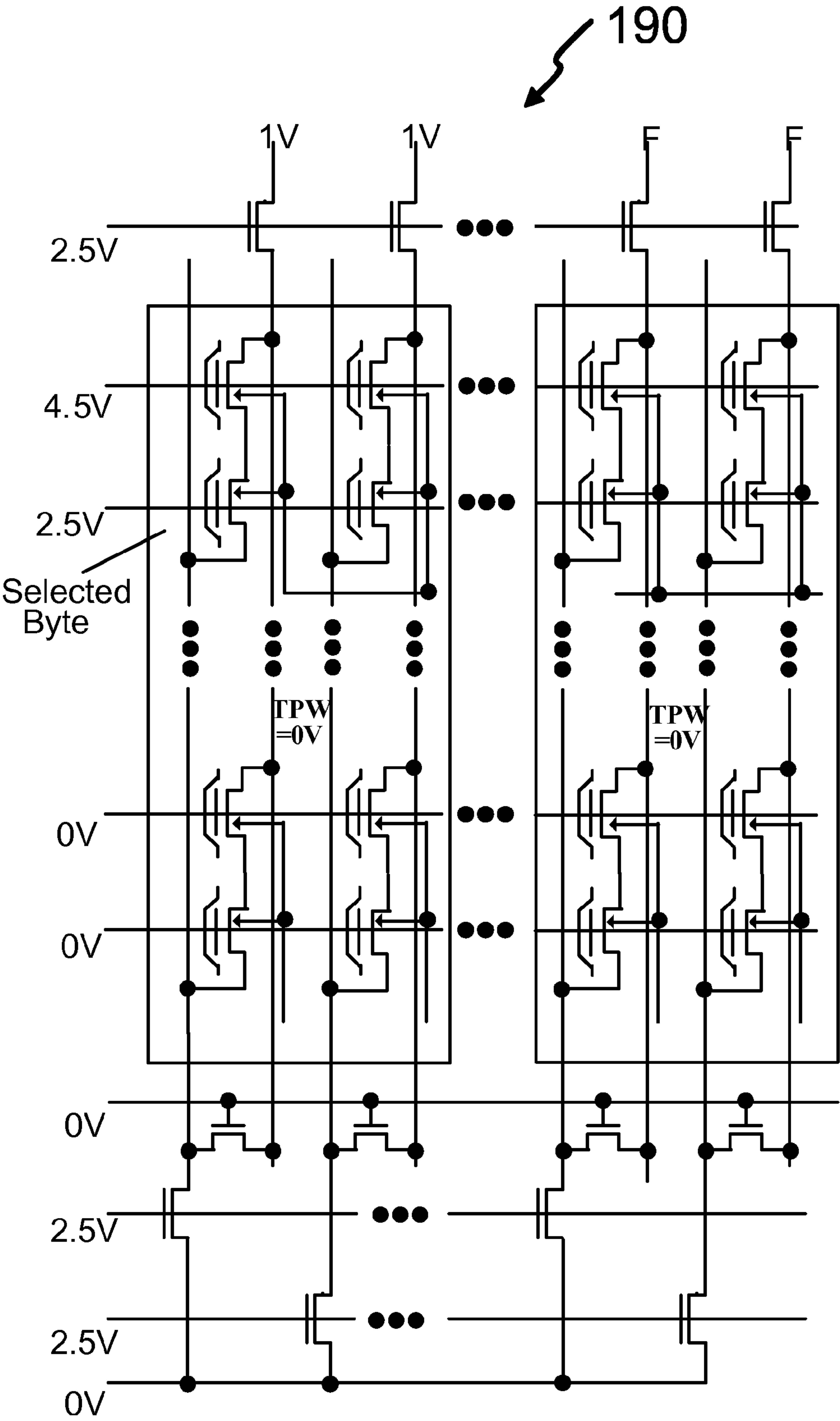
Fig. 15A
