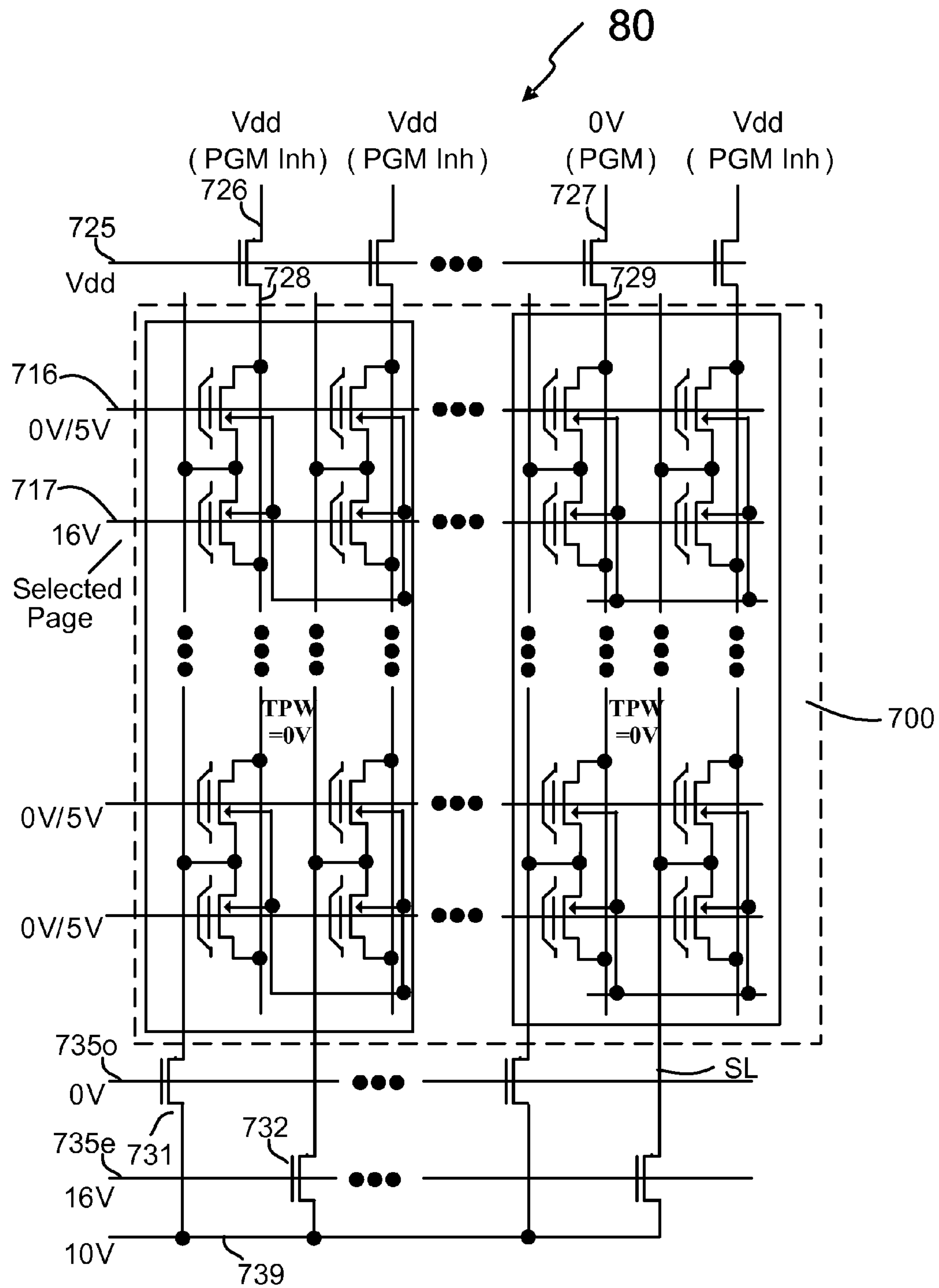
Fig. 7B
