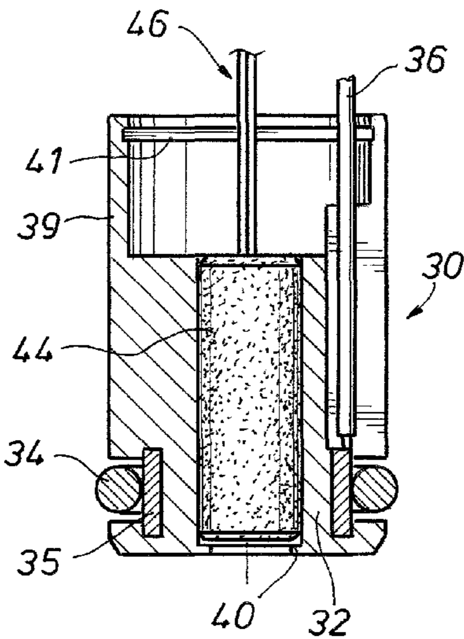
FIG. 4A
