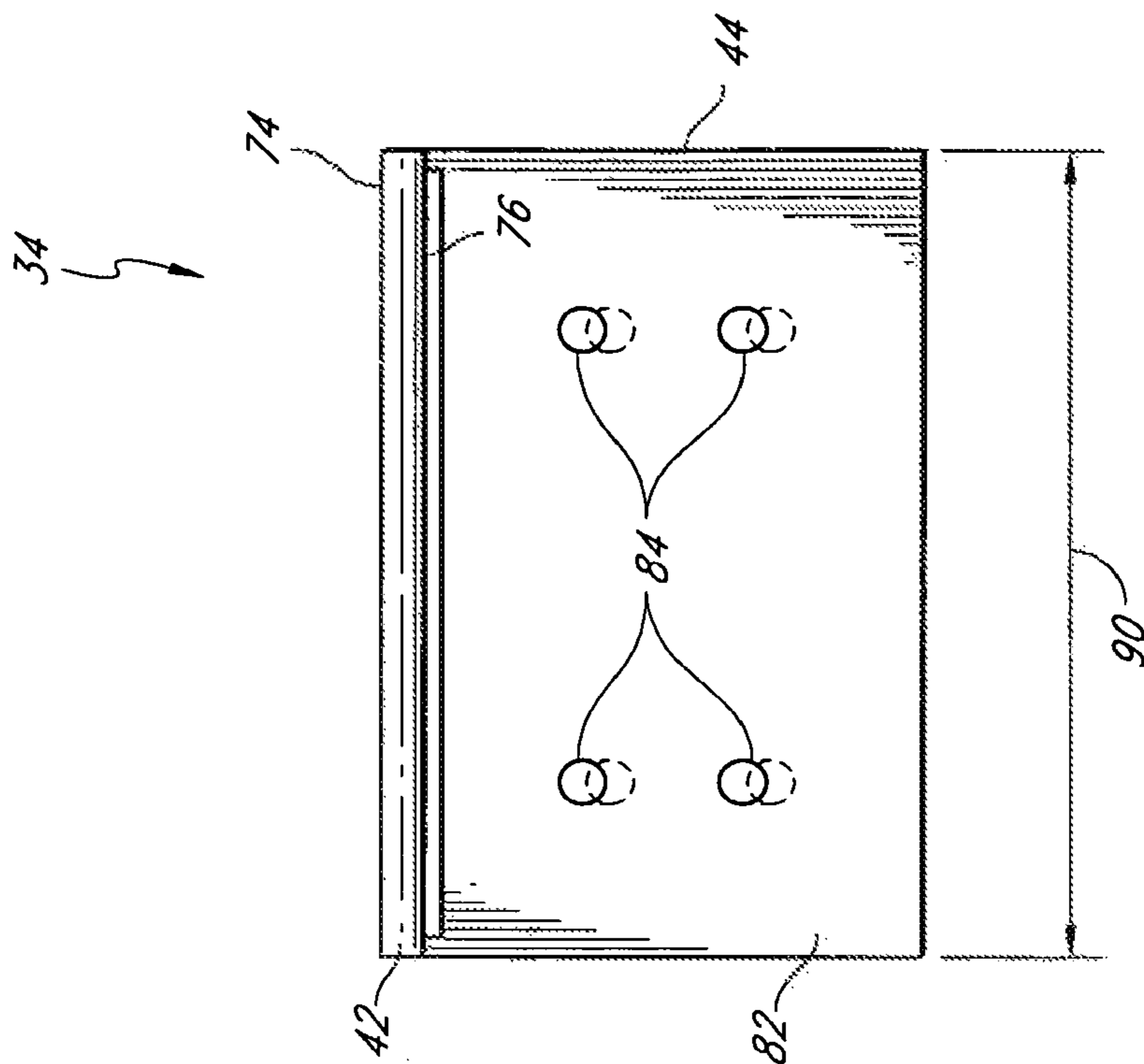
FIG. 3B
