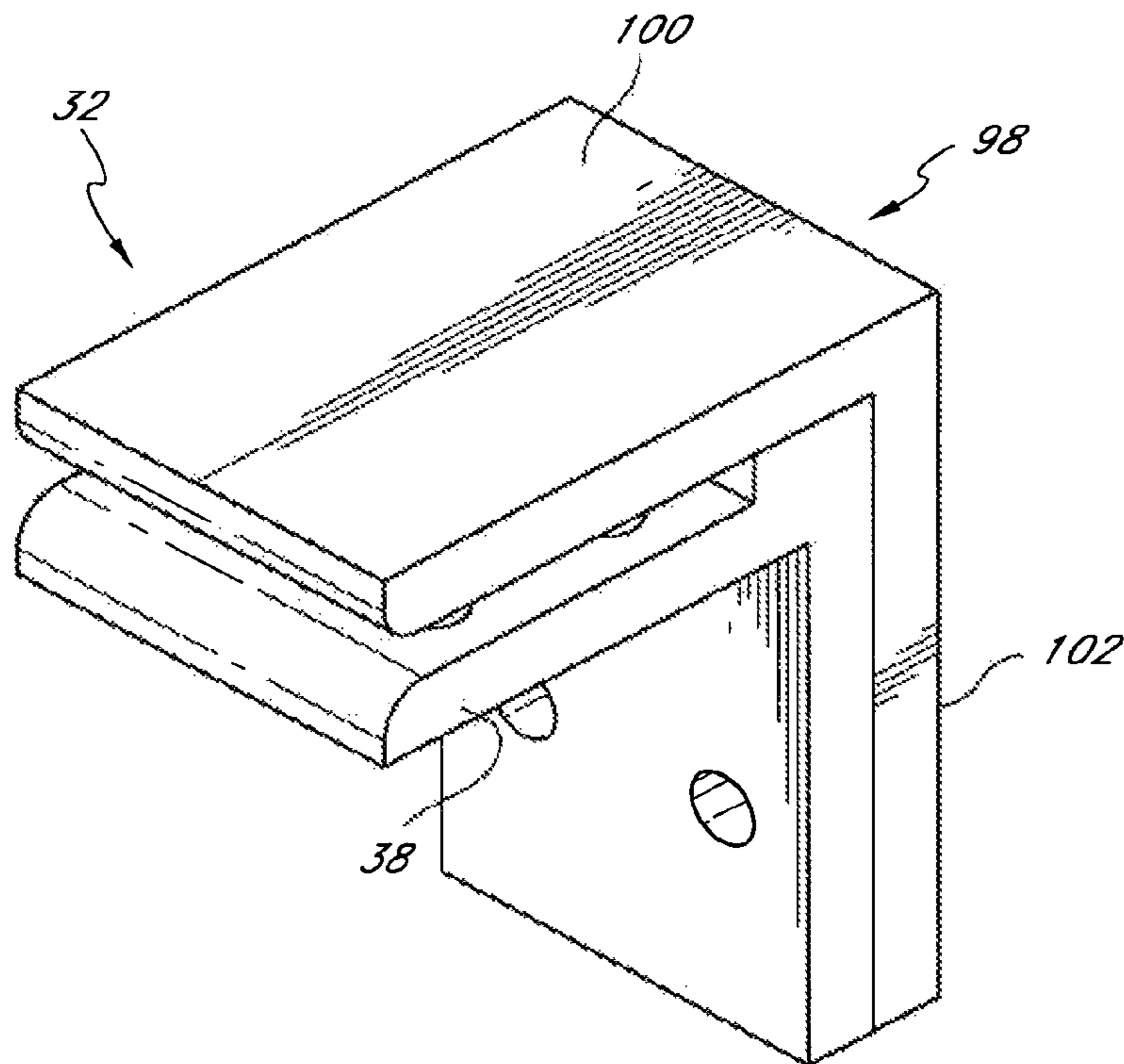
FIG. 7A
