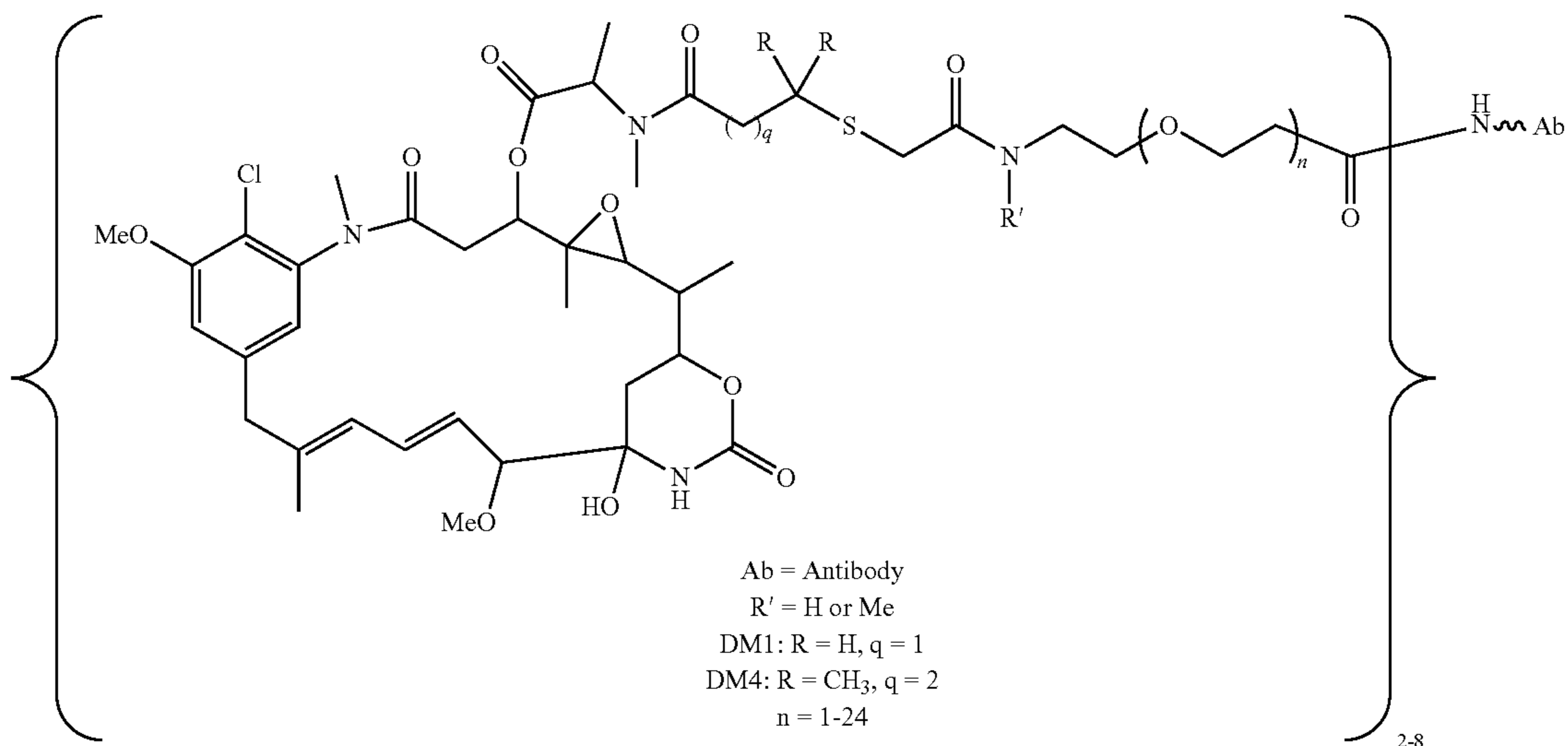
Ab-PEG-SIA-DM1/DM4
