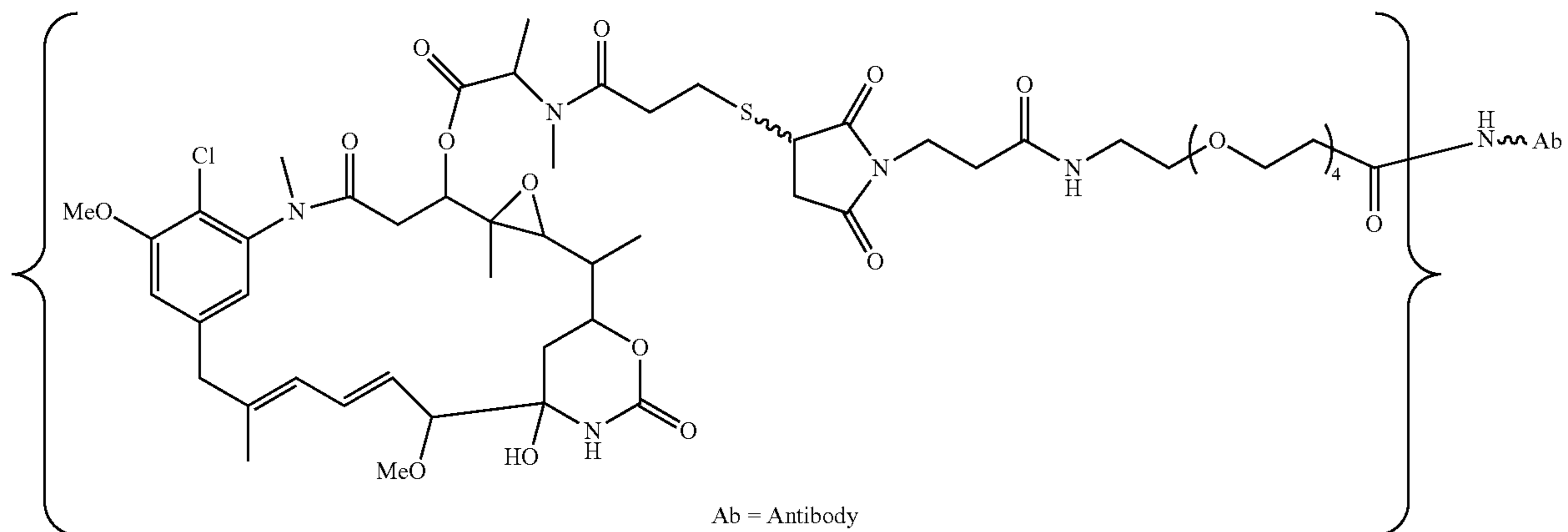
Ab-PEG4-Mal-DM1
