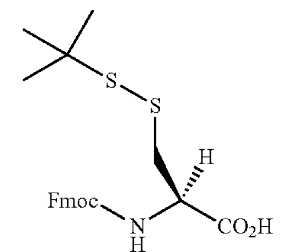
N- \alpha -Fmoc-S-S-t-Bu-L-cysteine
