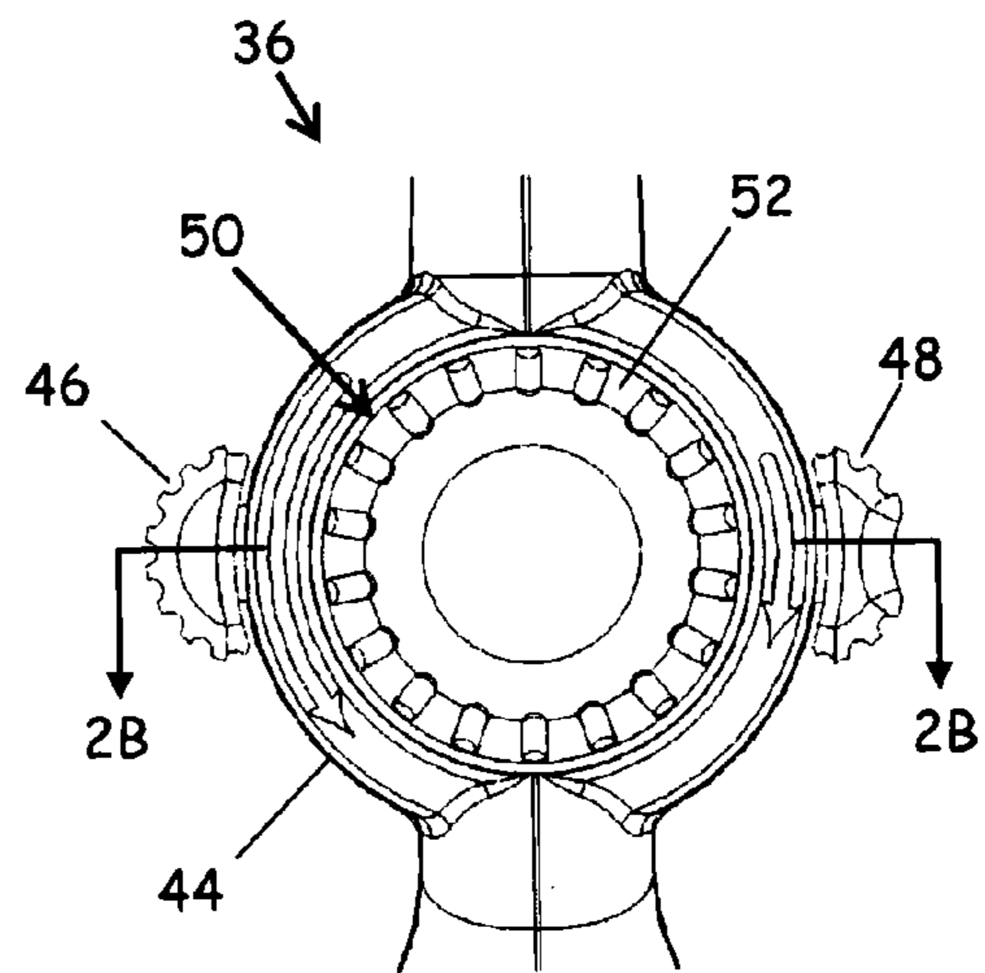
FIG. 2A
