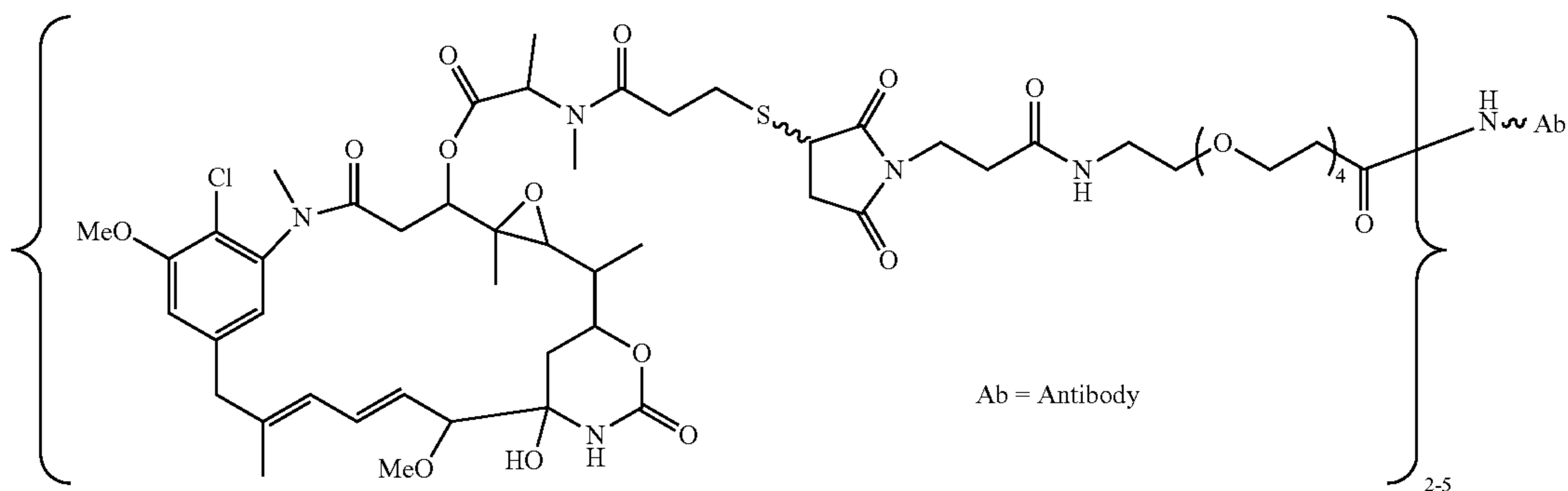
Ab-PEG4-Mal-DM1
