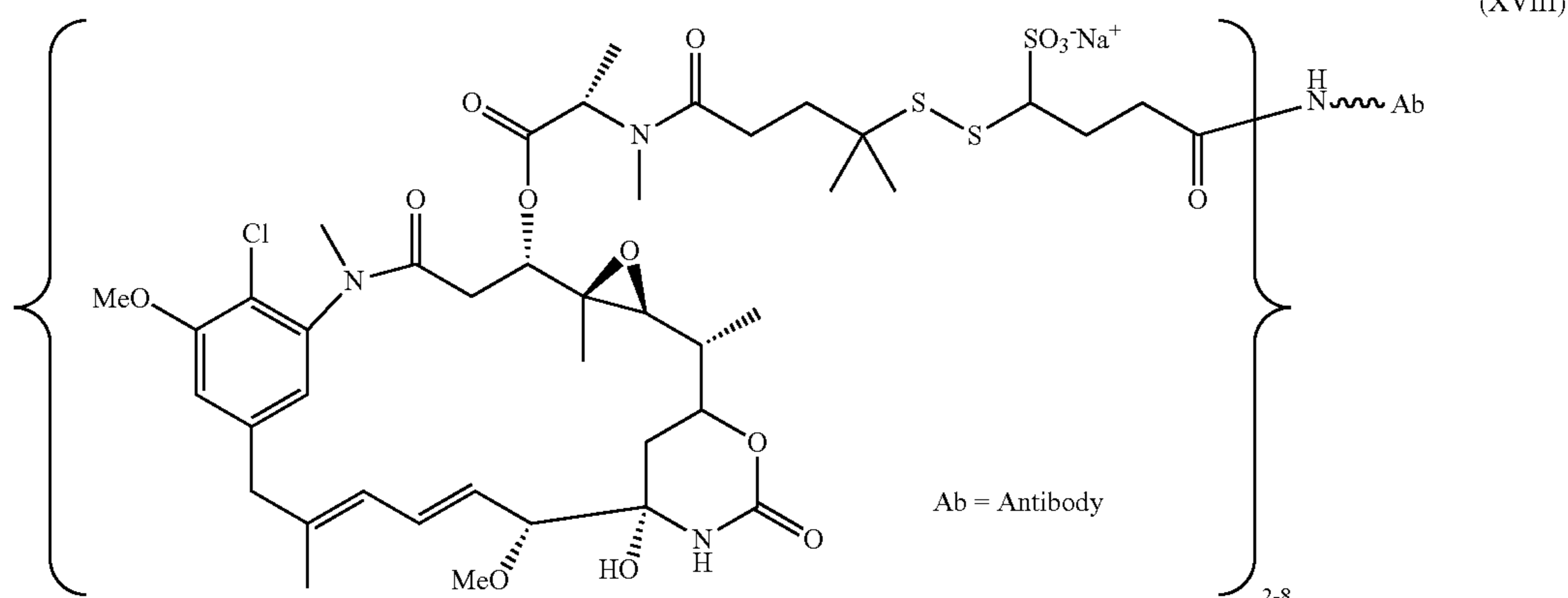
Ab-sulfo-SPDB-DM4
