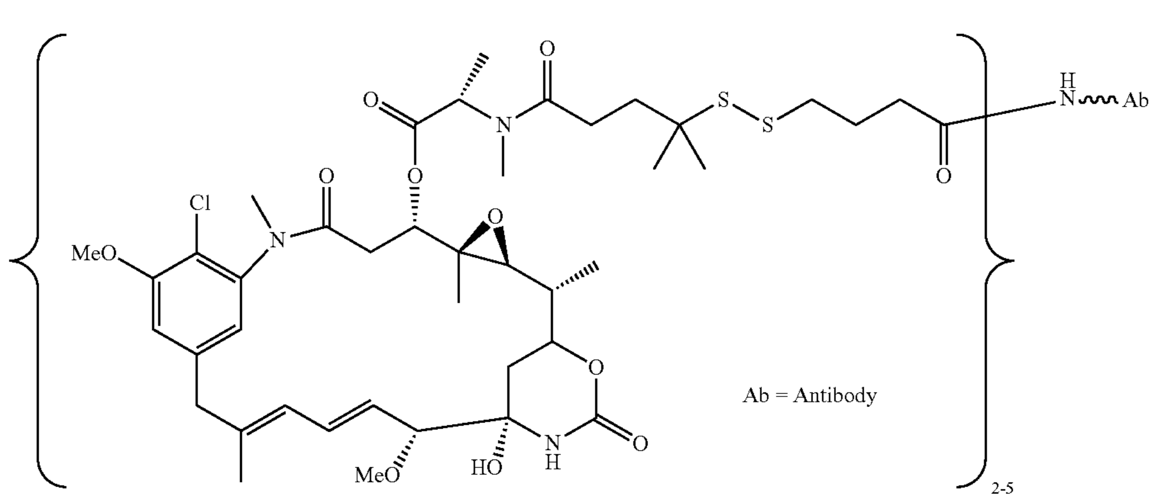
Ab-SPDB-DM4
