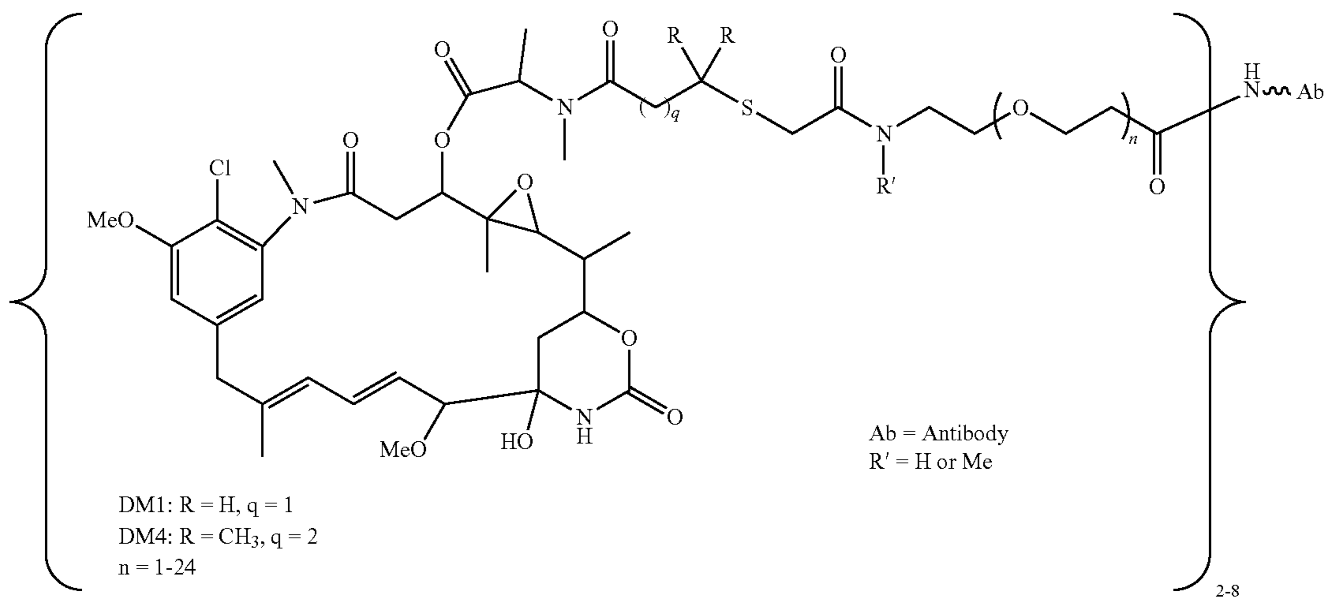
Ab-PEG-SIA-DM1/DM4
