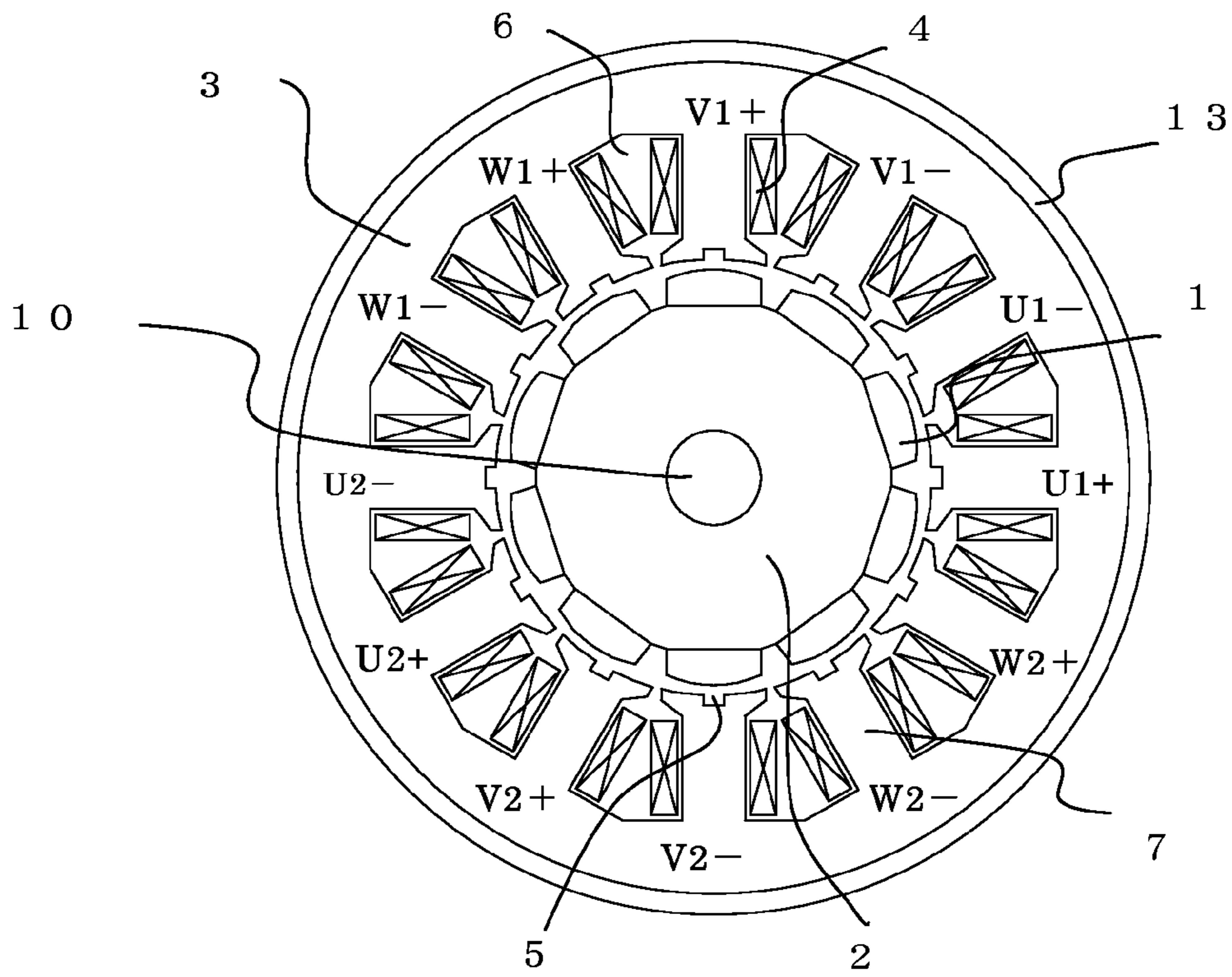
D1—D2 cross-section
