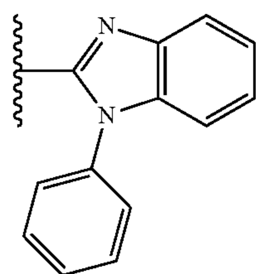
1-phenyl-1H-benzo[d]imidazol-2-yl
