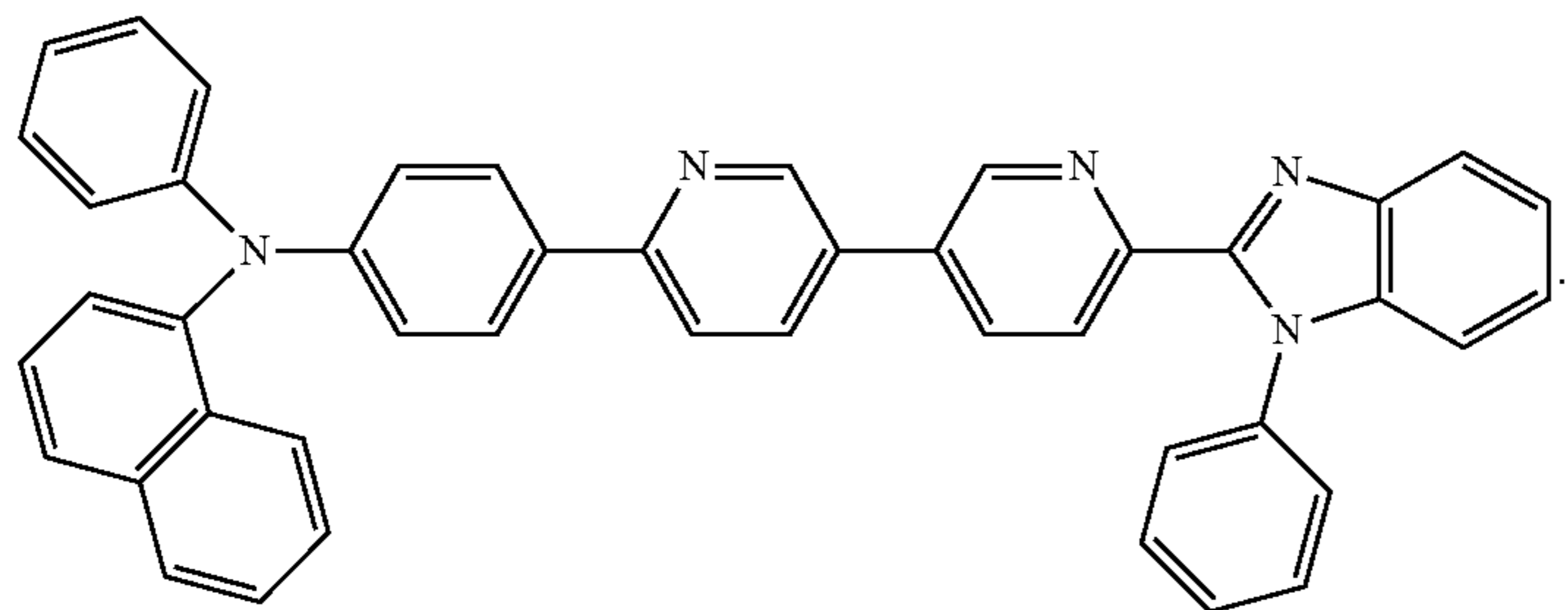
N-phenyl-N-(4-(6'-(1-phenyl-1H-benzo[d]imidazol-2-yl)-[3,3'-bipyridin]-6-yl)phenyl)naphthalen-1-amine, or
