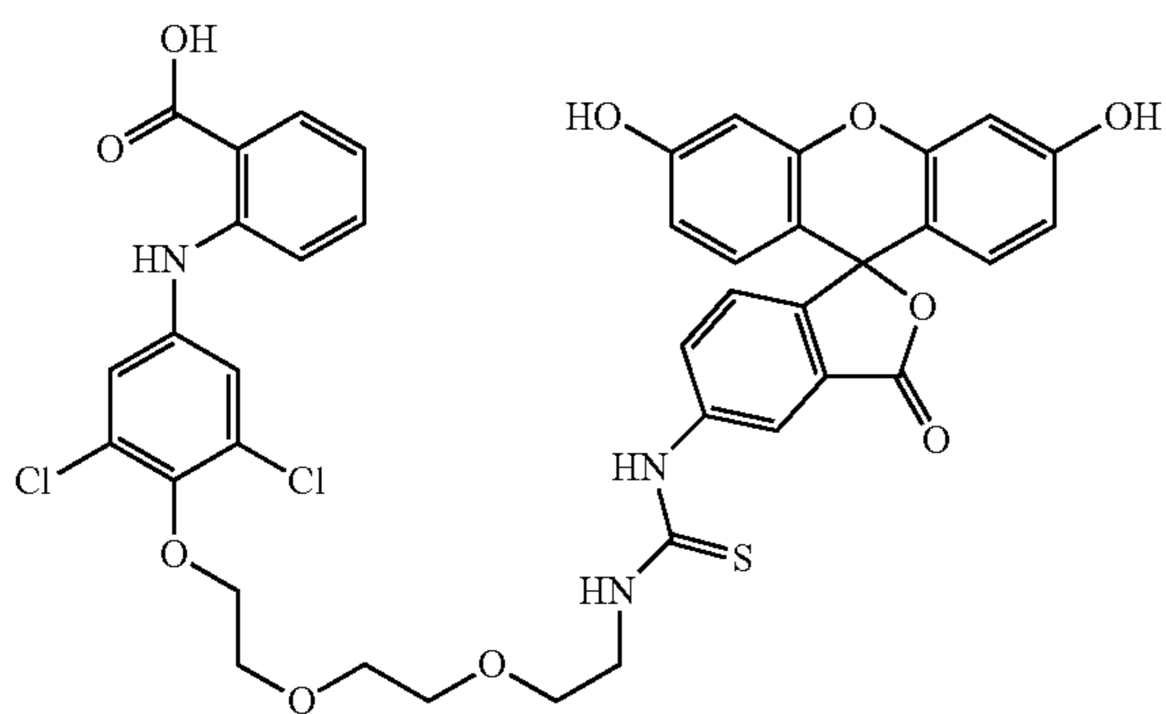
FP-probe 5
