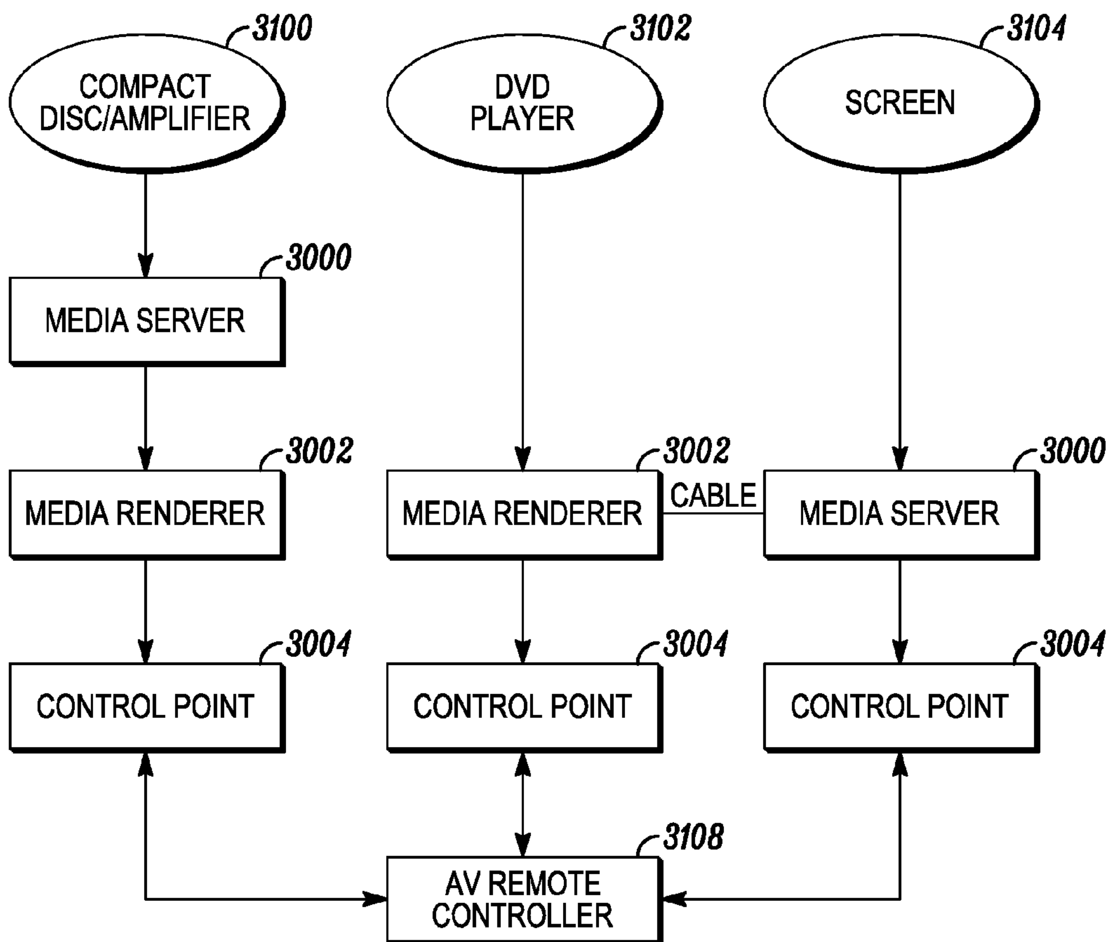
FIG. 31
