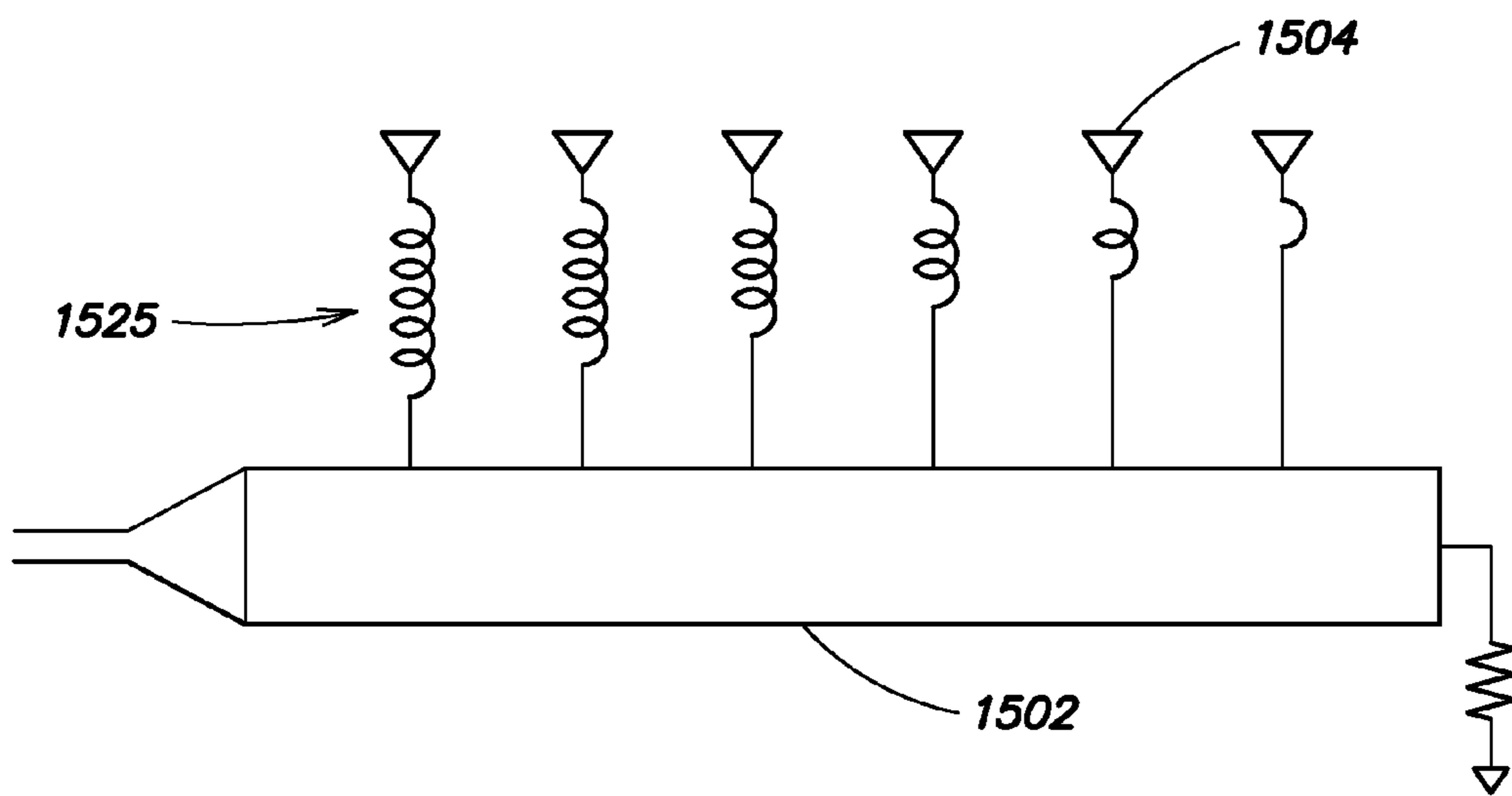
FIG. 15B
