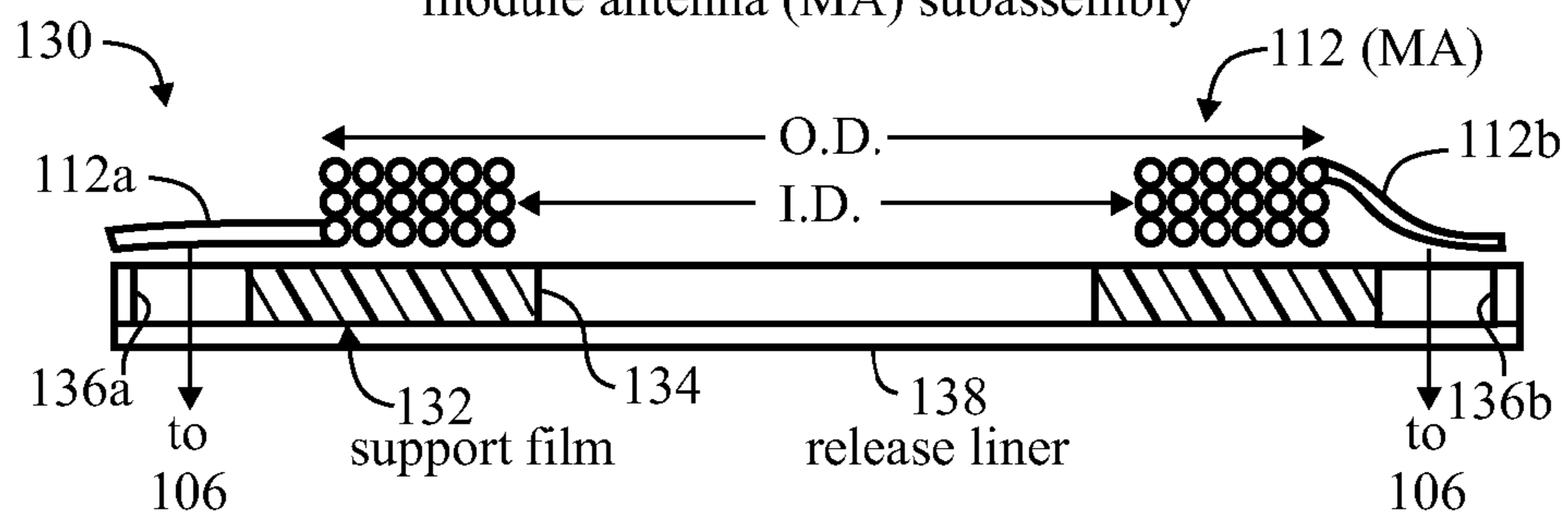
module antenna (MA) subassembly
