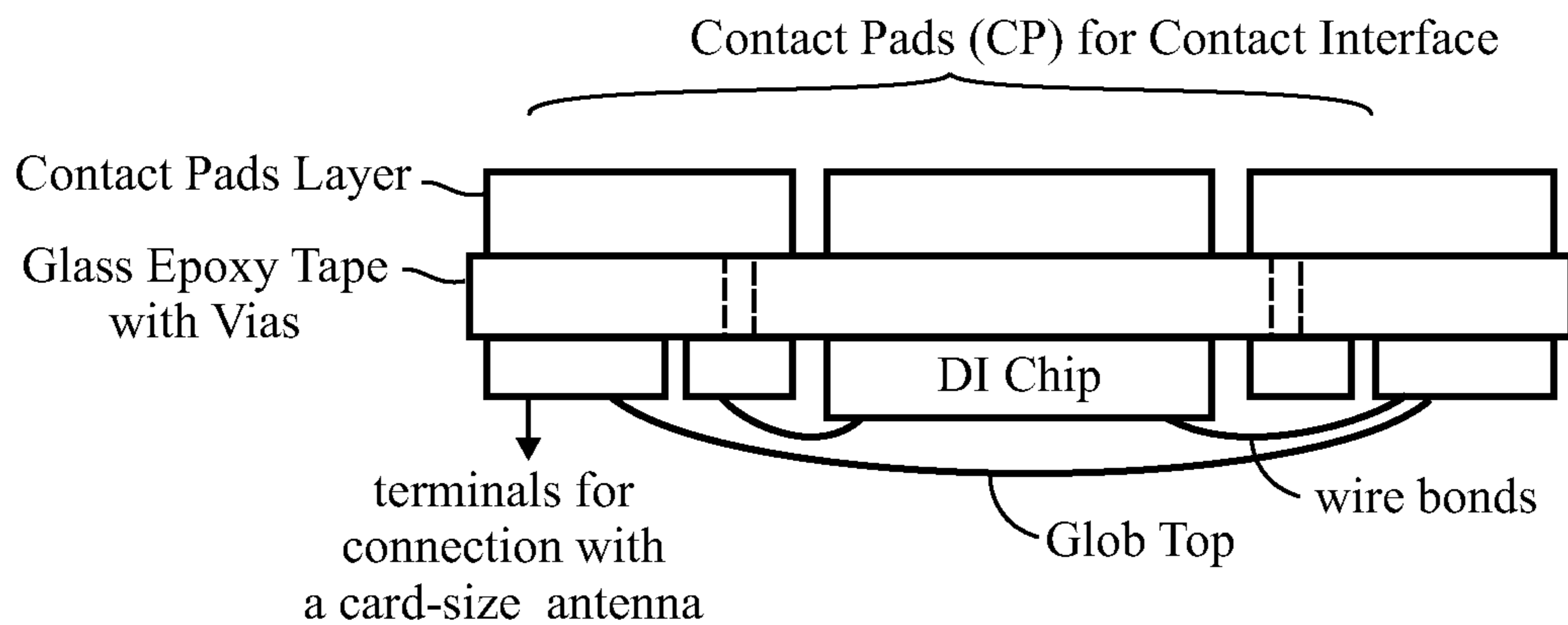
FIG. 1E DI Chip Module
