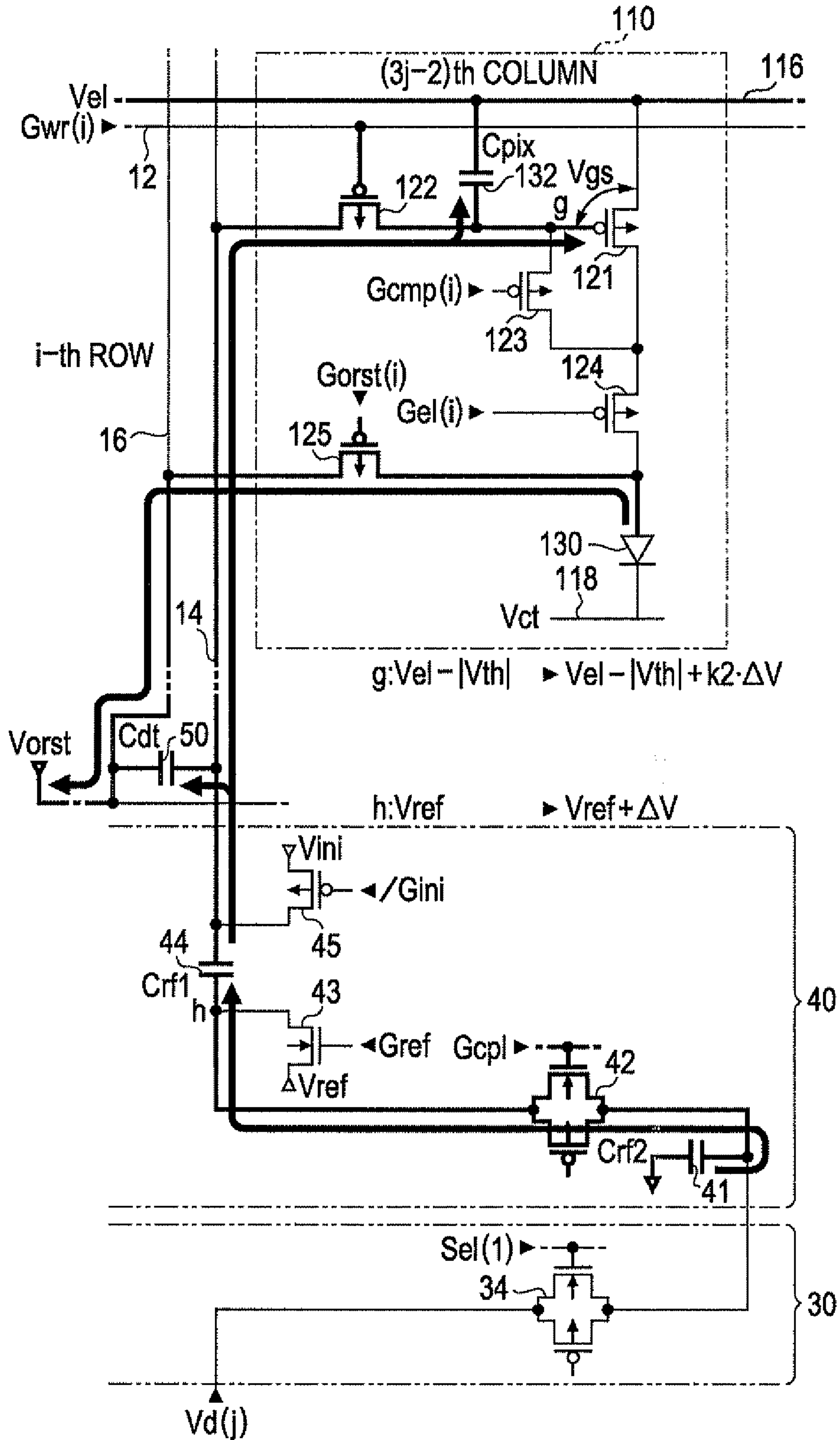
FIG. 8 <(d) WRITING PERIOD>
