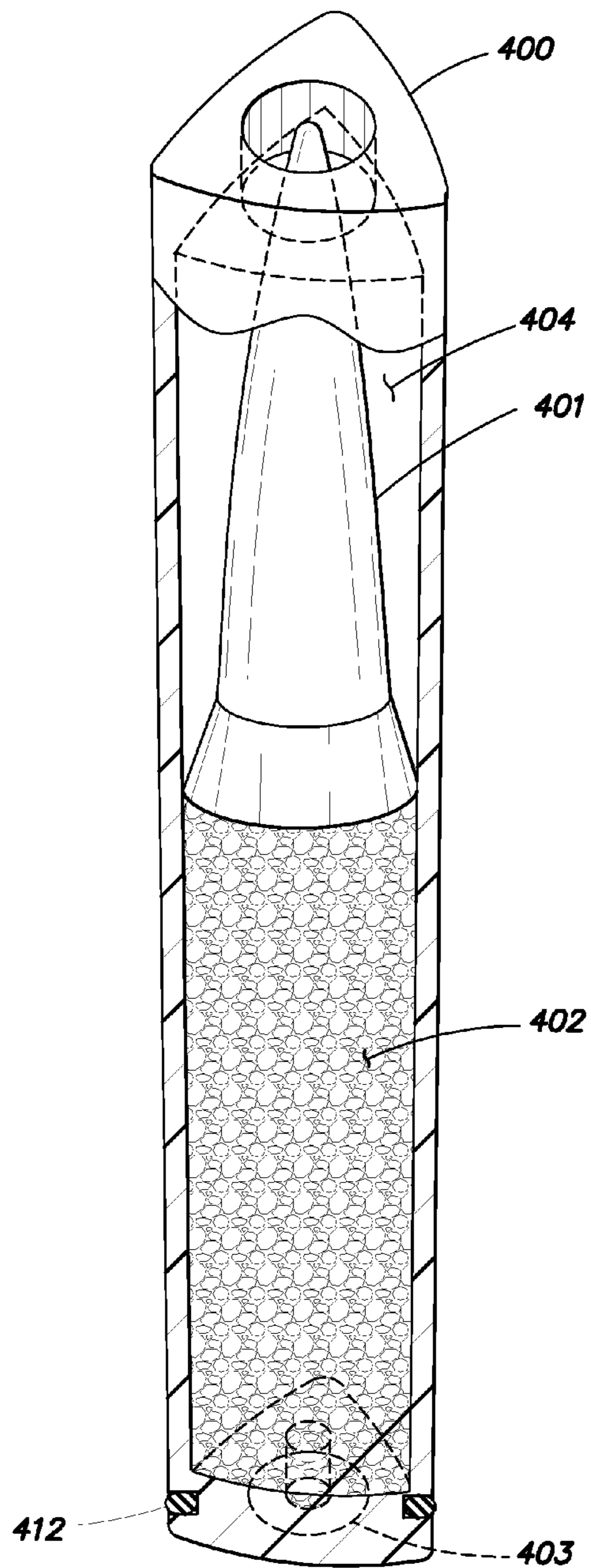
FIG. 4A
