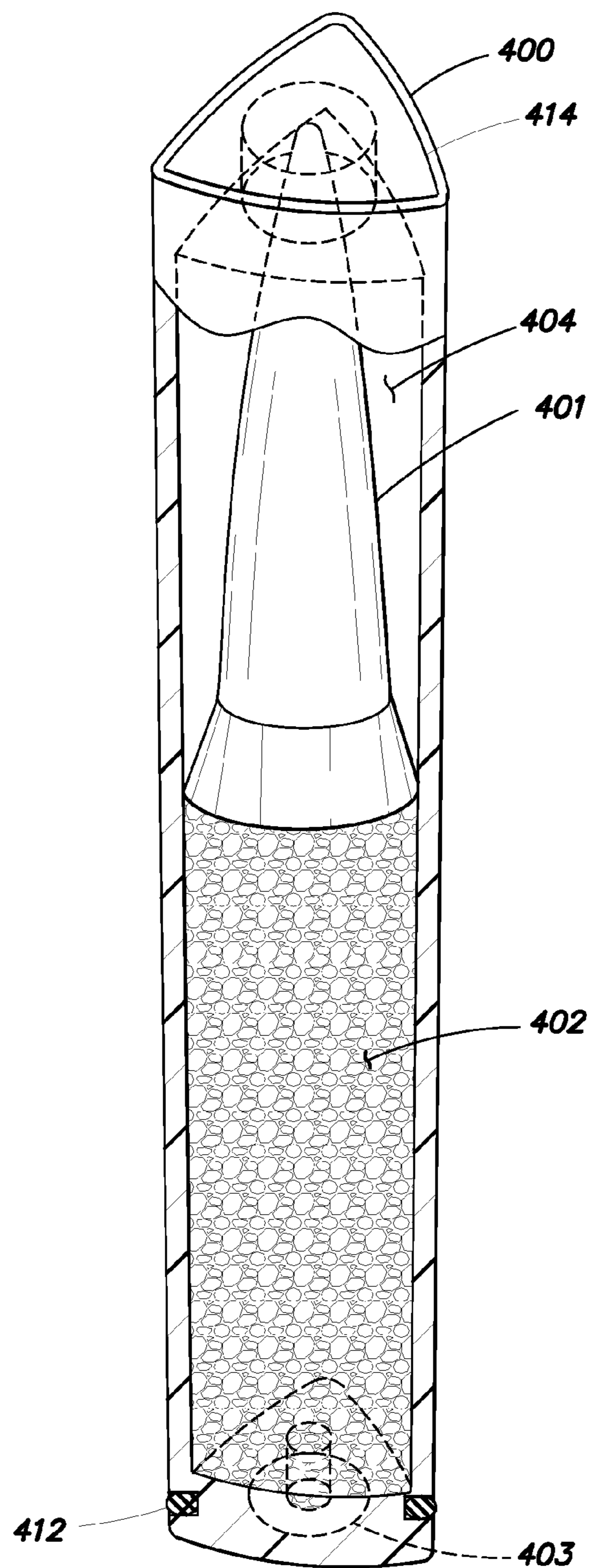
FIG. 4C
