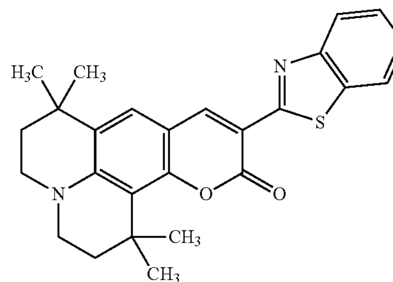
C545T
