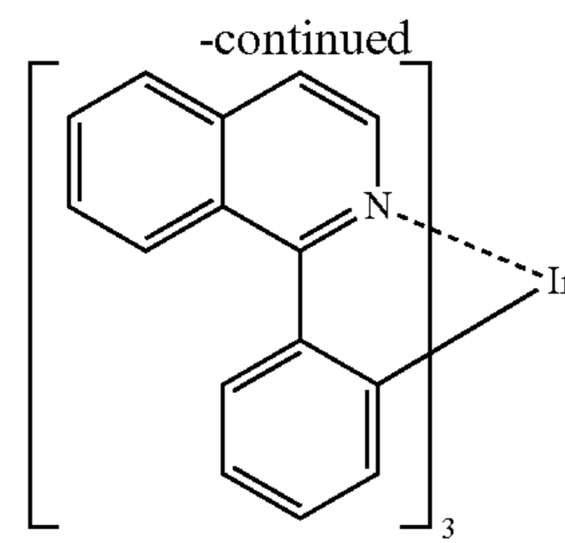
Ir(piq) 3
