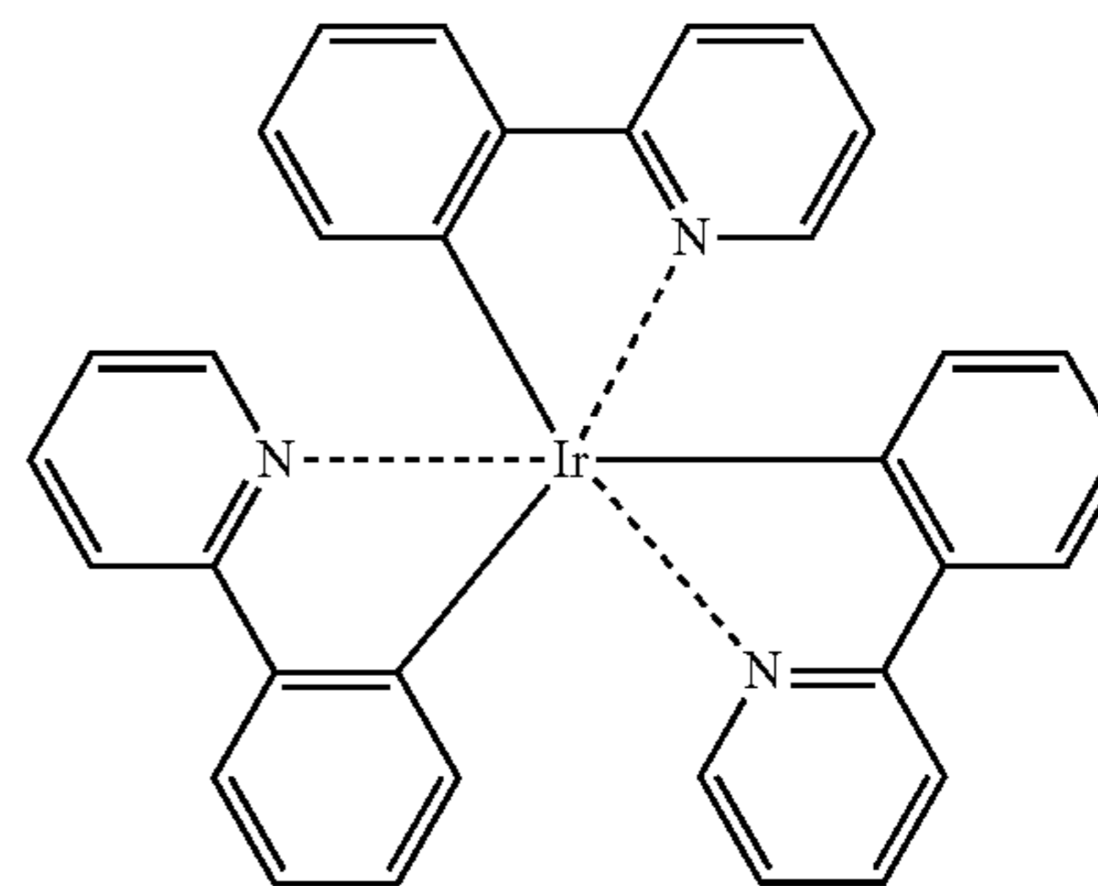
Ir(ppy) 3
