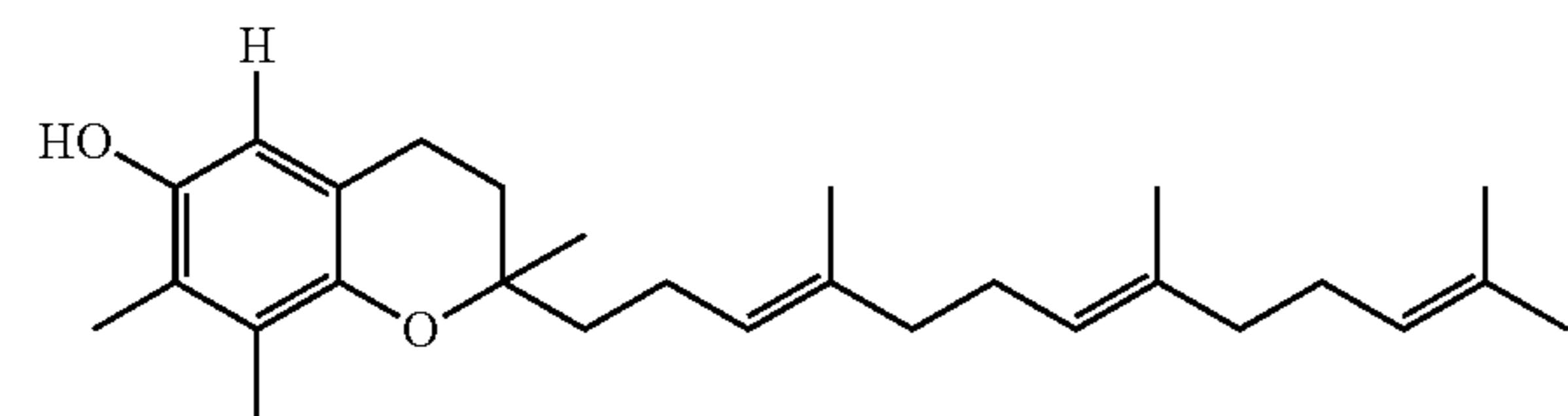
Gamma-tocotrienol
