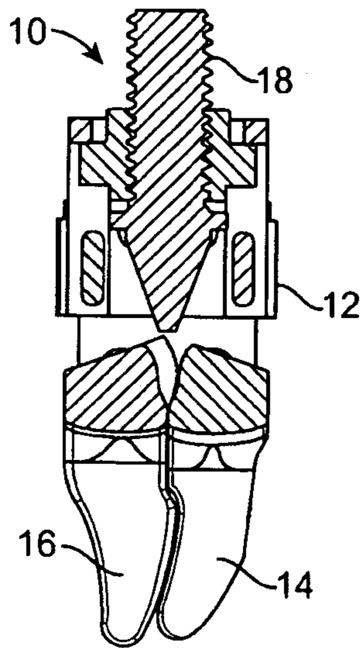
SECTION A-A
