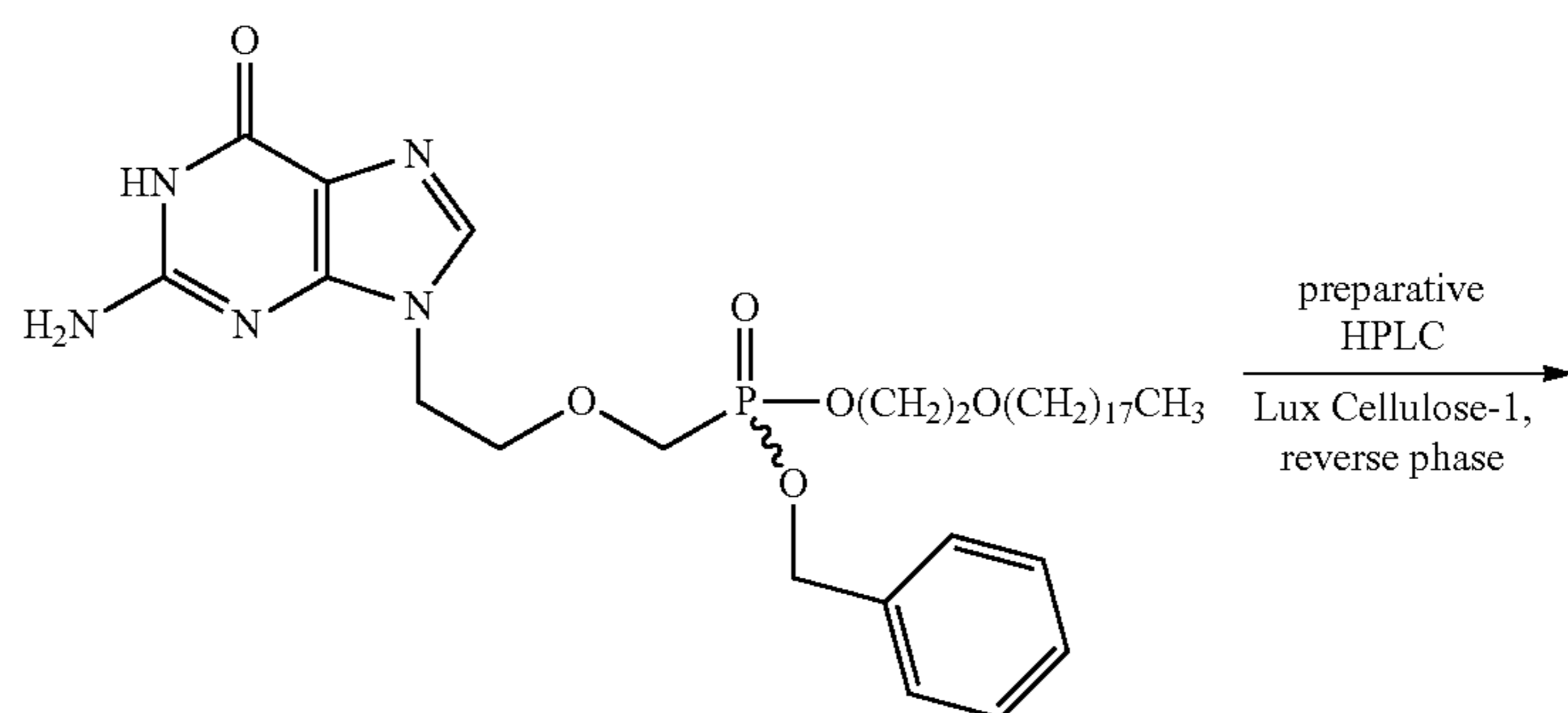
Bn-ODE-PMEG
