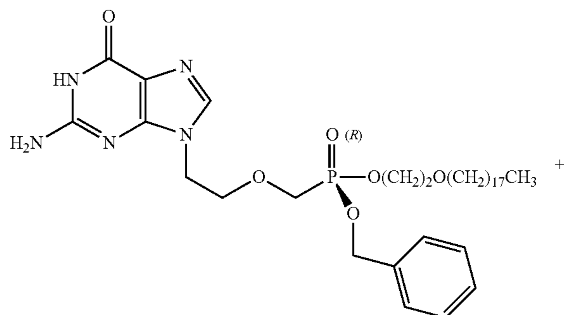
Bn-ODE-PMEG
