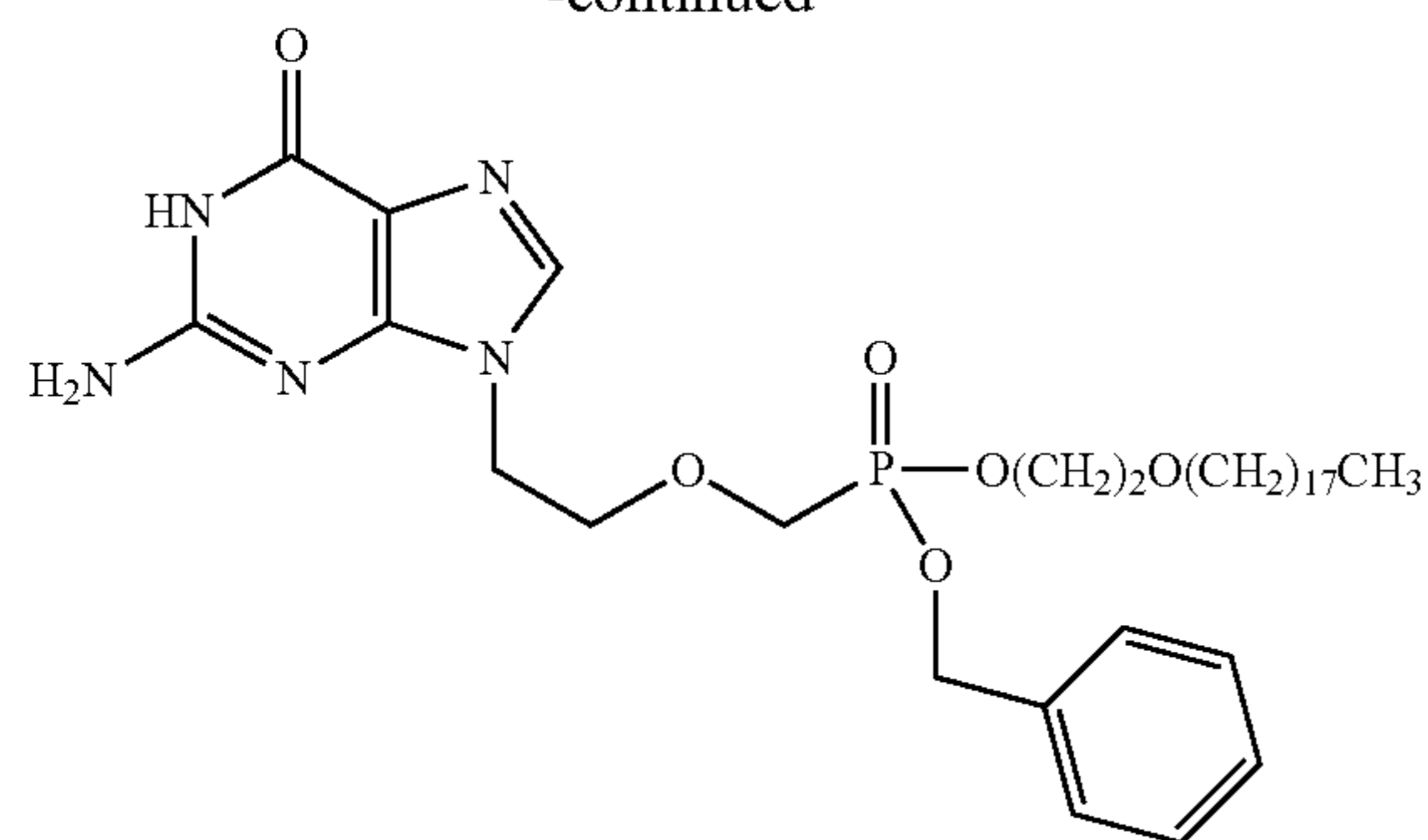
Bn-ODE-PMEG
