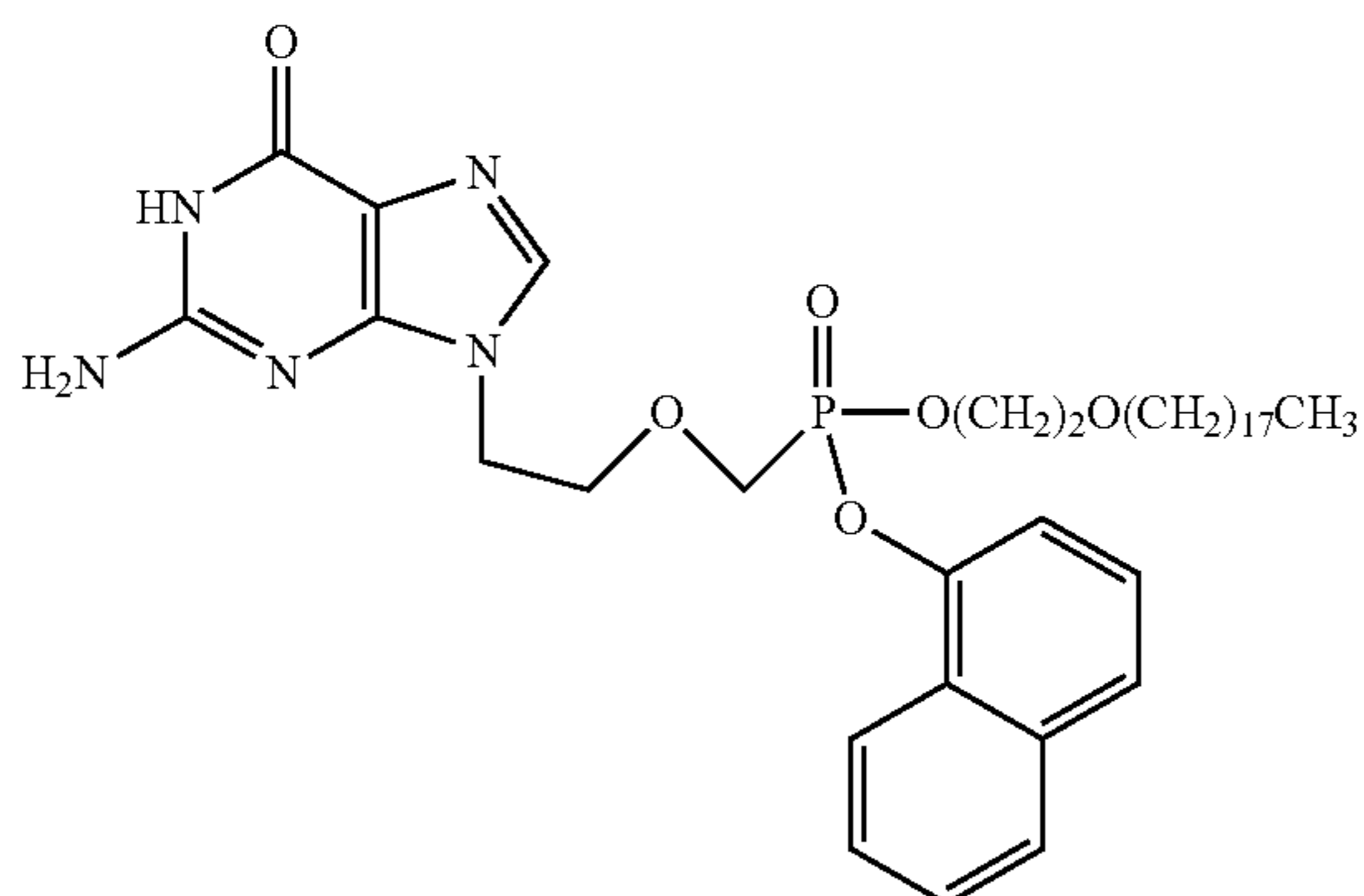
ODE-PMEG
