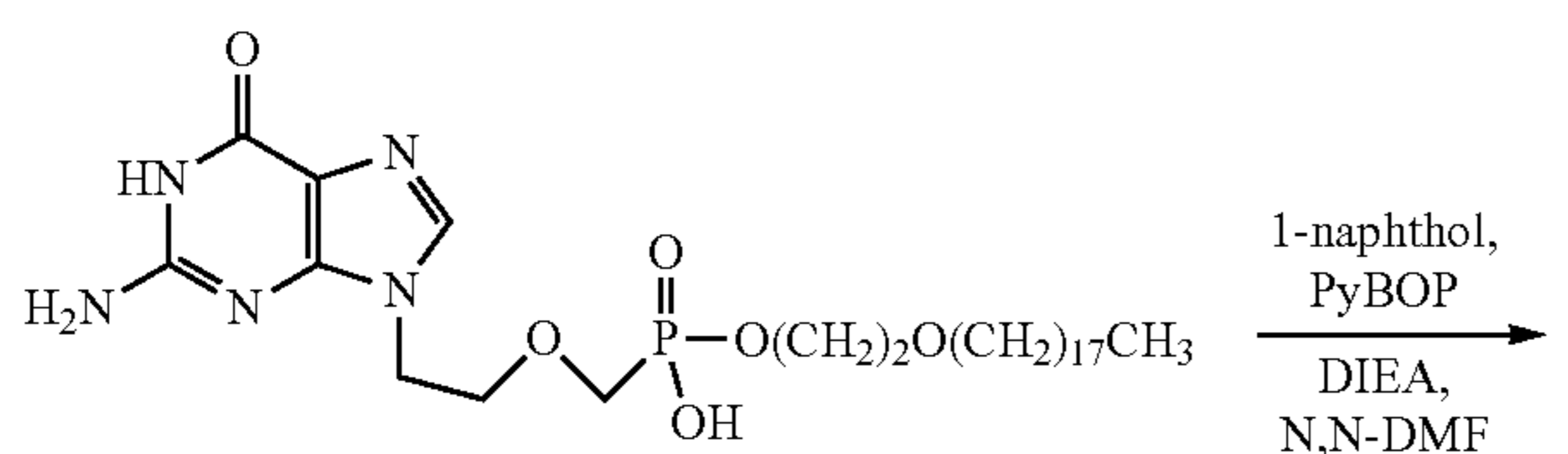
ODE-PMEG
