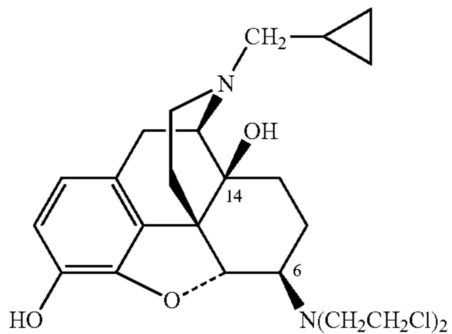
\beta -CNA
