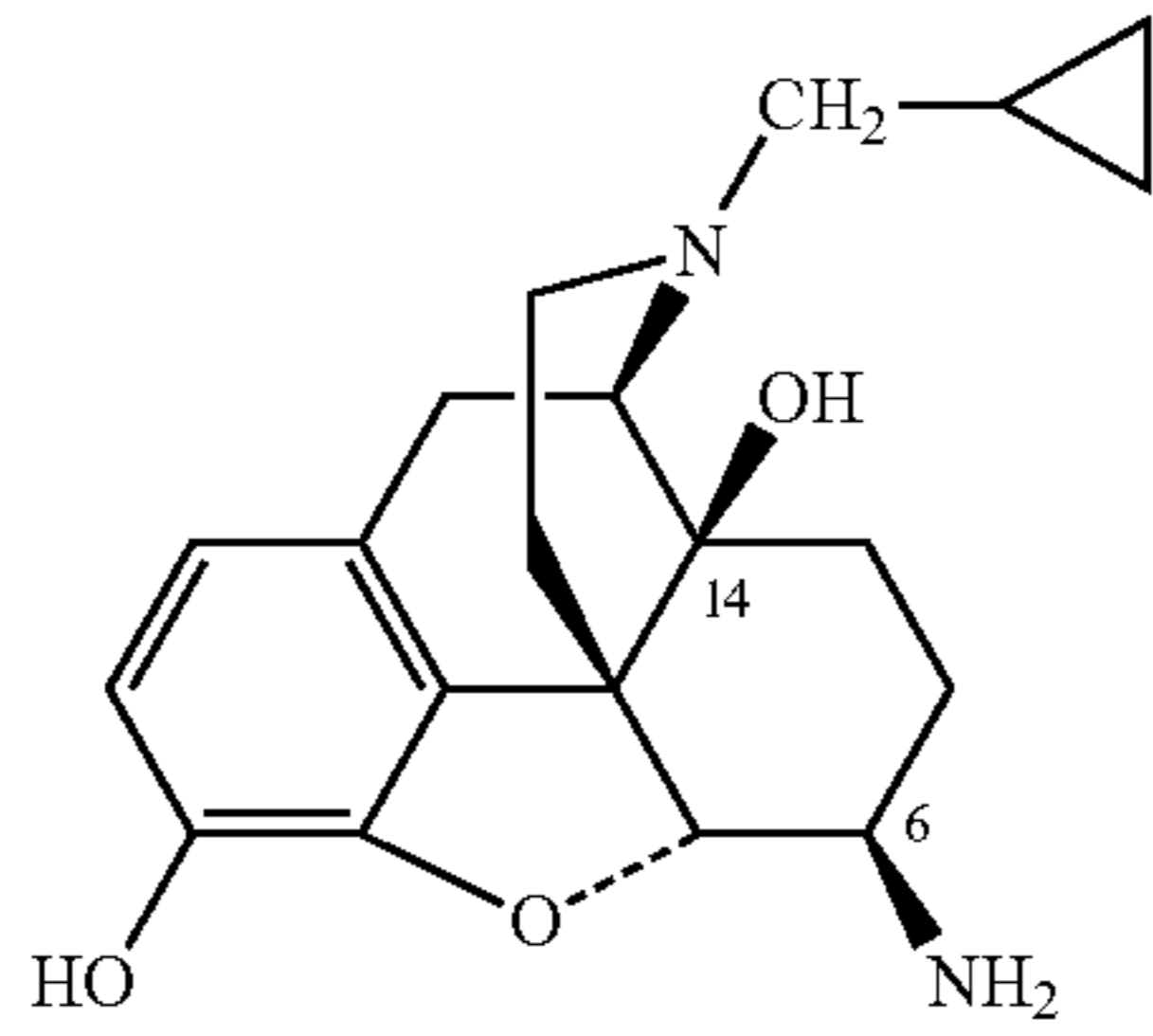
\beta -Naltrexamine
