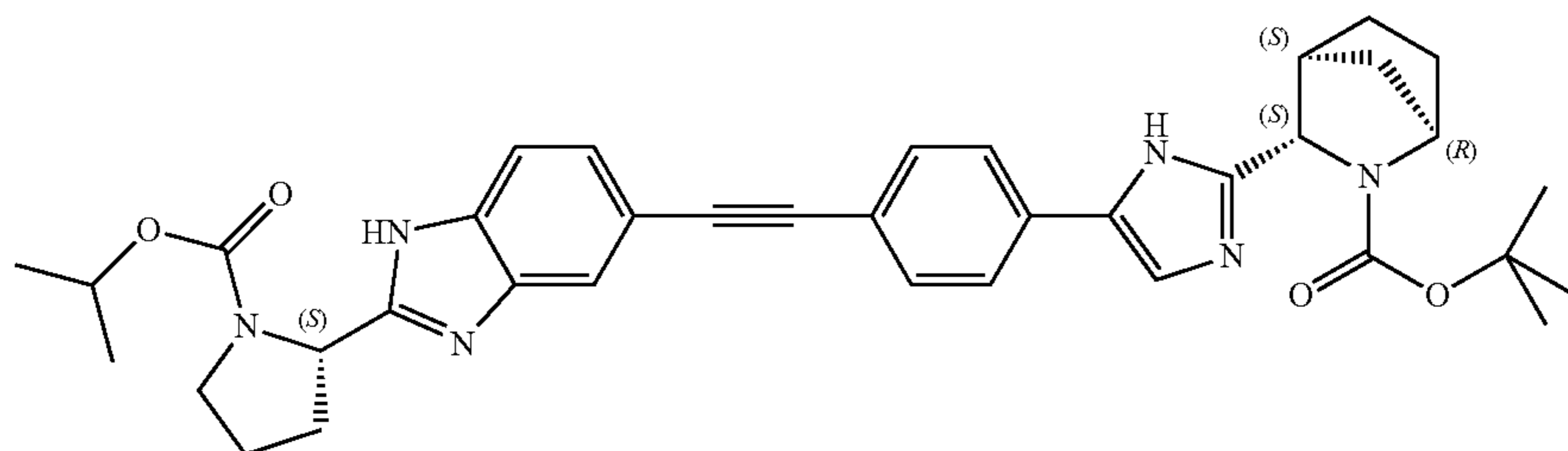
Example 336
