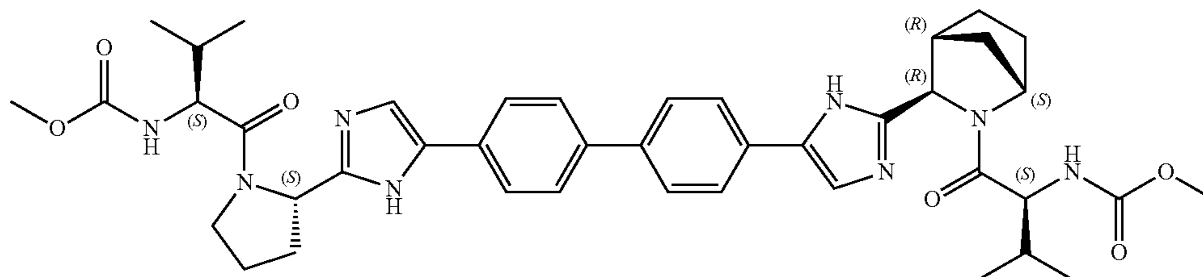
Example 246
