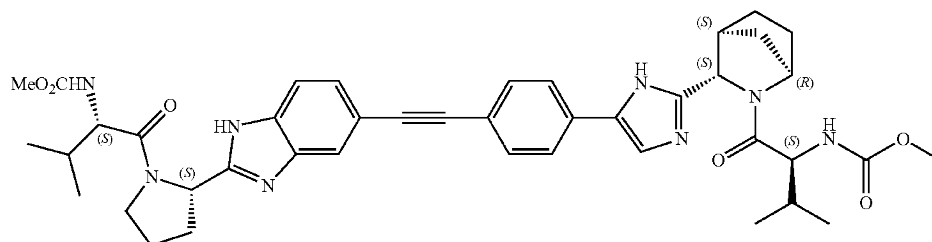
Example 319
