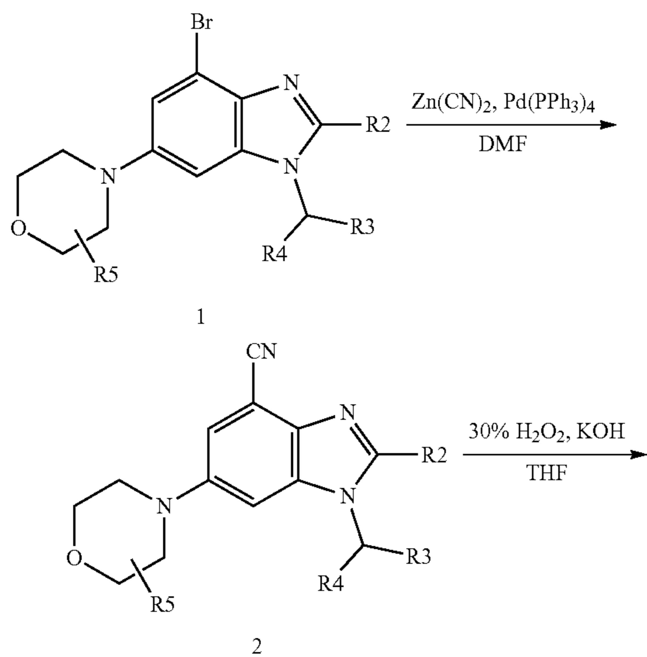
Scheme VI
