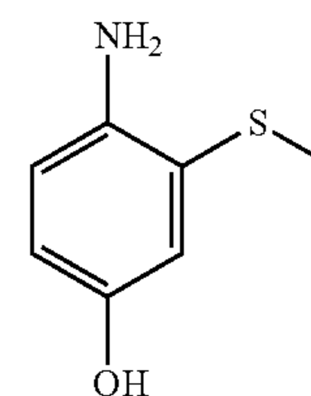
4-amino-3-(methylthio)phenol
