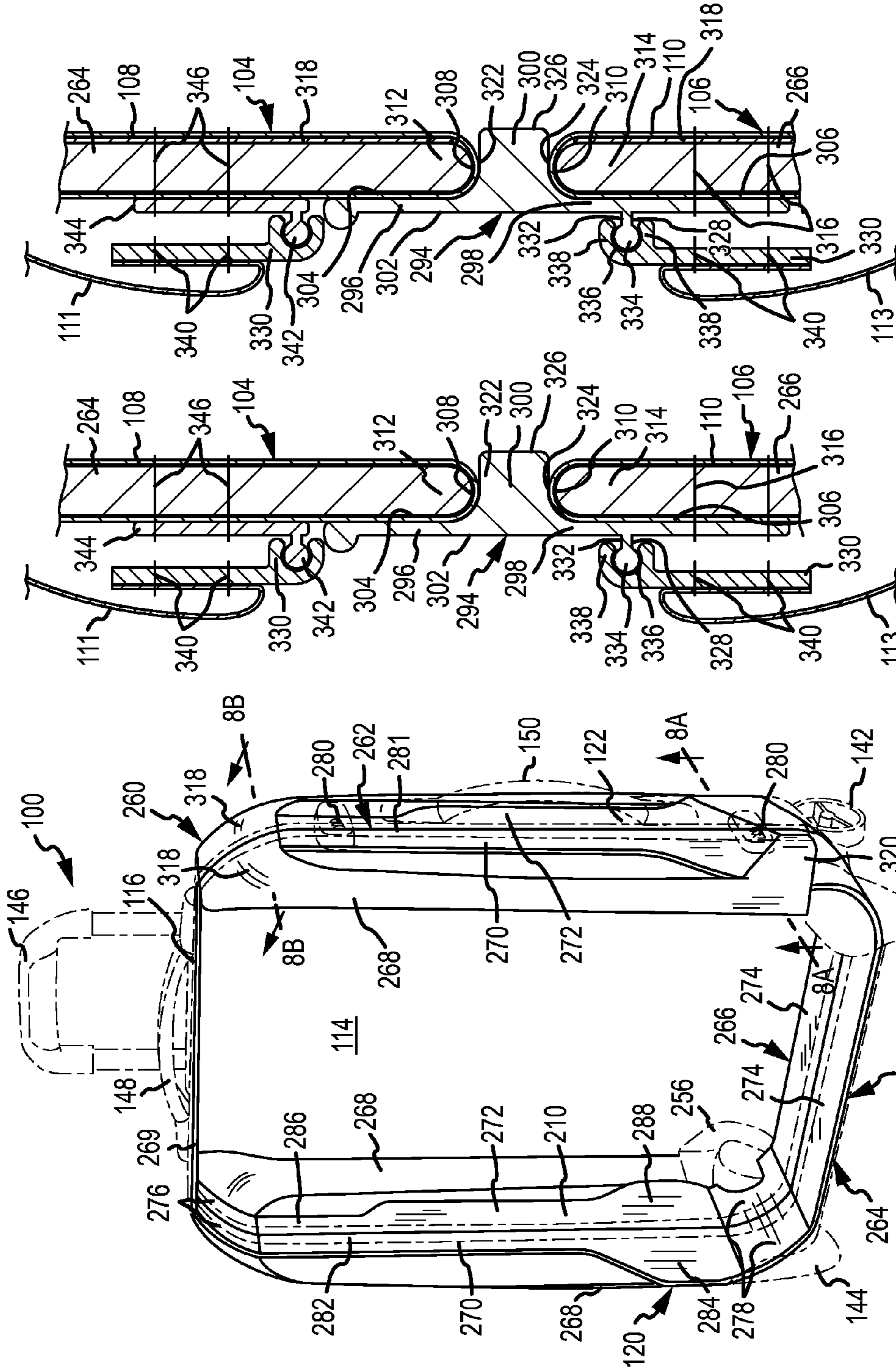
FIG. 8A
