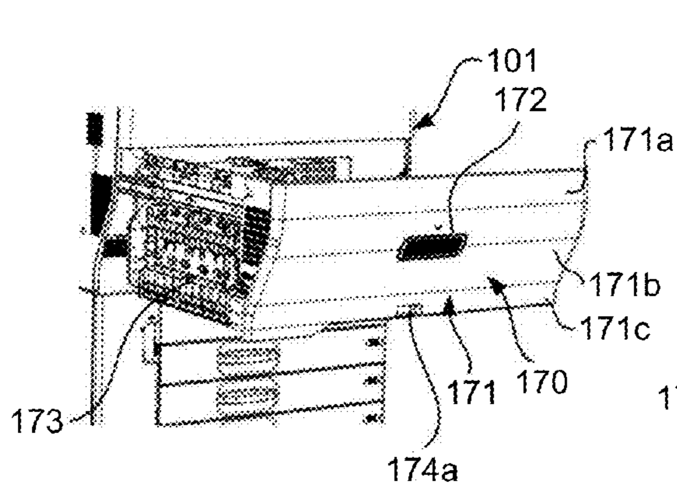
FIG.5B
