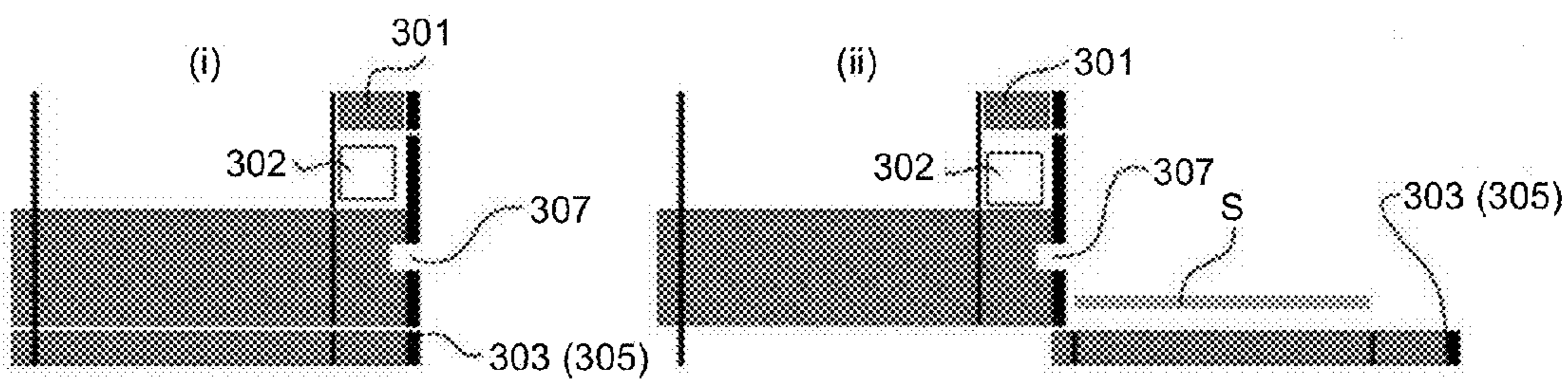
FIG.9D
