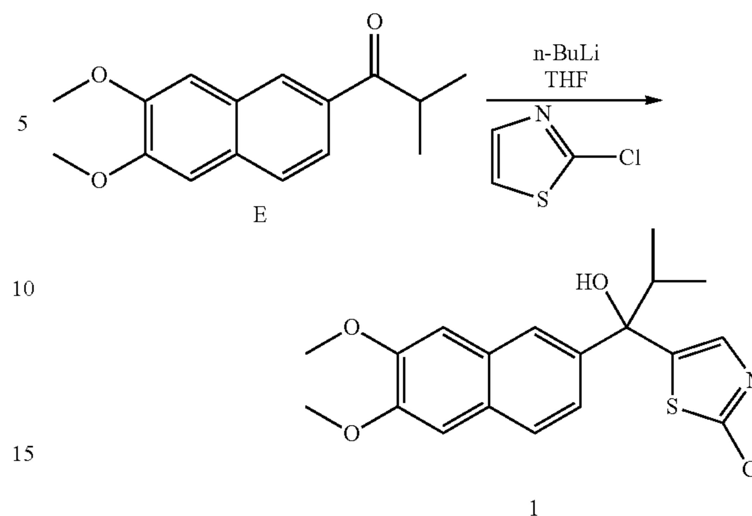
1-(2-Chloro-thiazol-5-yl)-1-(6,7-dimethoxynaphthalen-2-yl)-2-methylpropan-1-ol (1)
