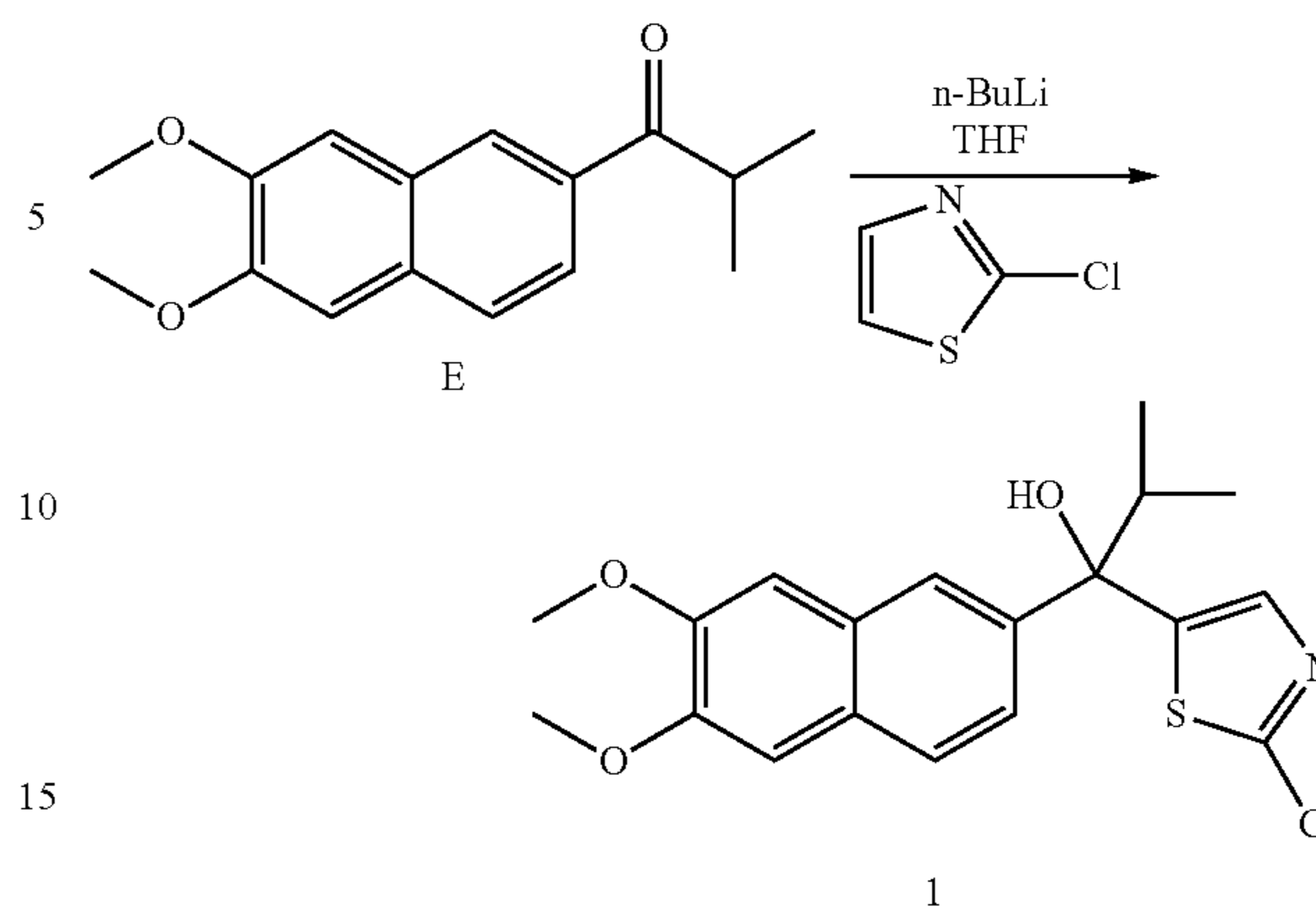
1-(2-Chloro-thiazol-5-yl)-1-(6,7-dimethoxynaphthalen-2-yl)-2-methylpropan-1-ol (1)
