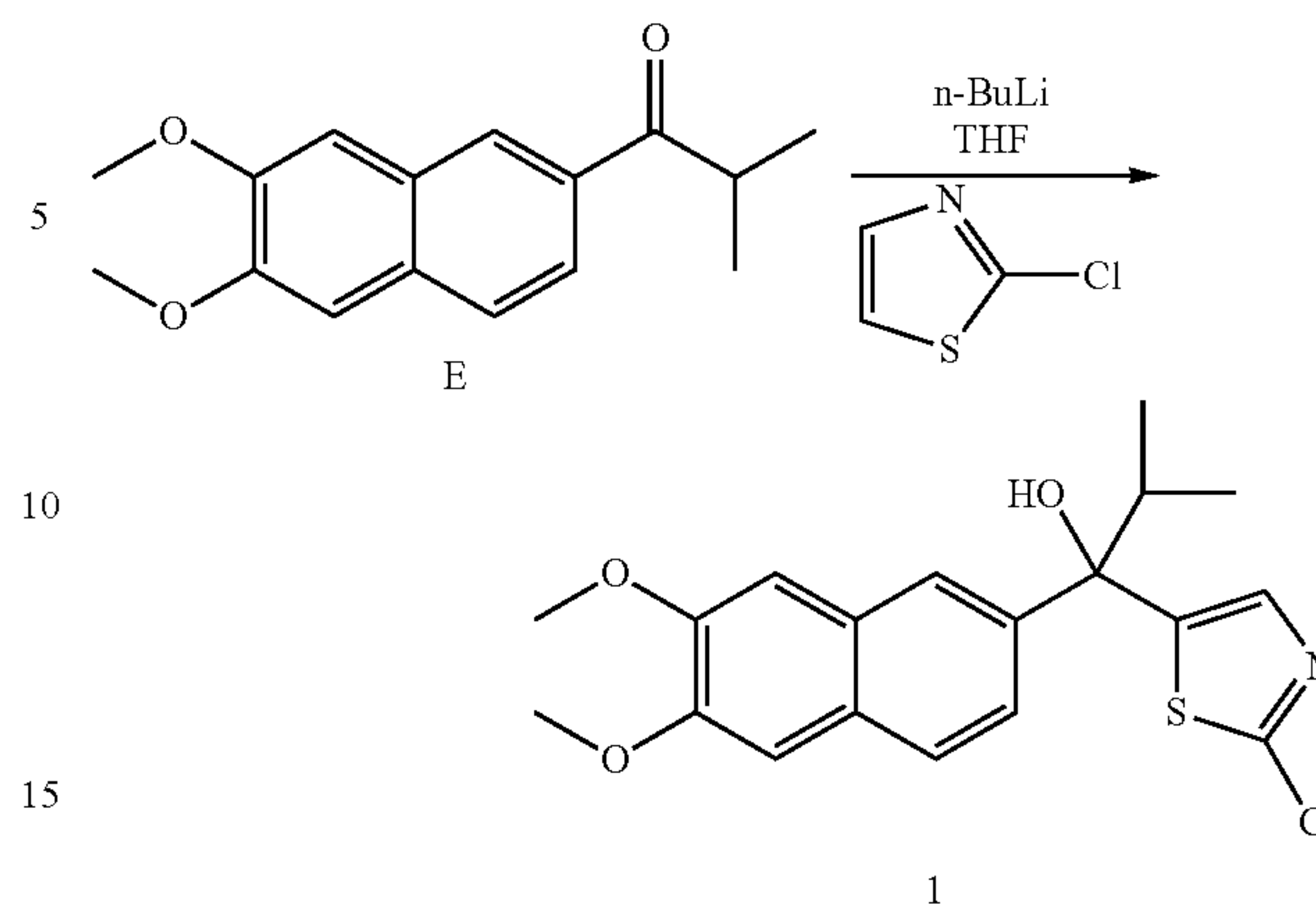
1-(2-Chloro-thiazol-5-yl)-1-(6,7-dimethoxynaphthalen-2-yl)-2-methylpropan-1-ol (1)
