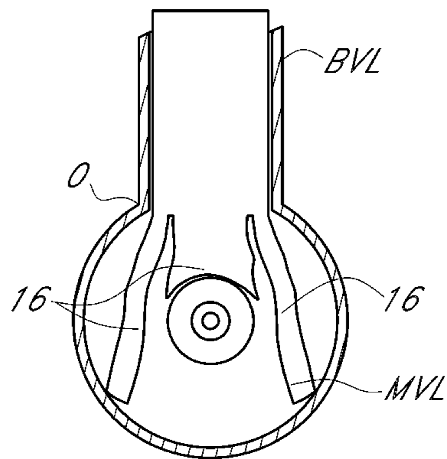
FIG. 11B
