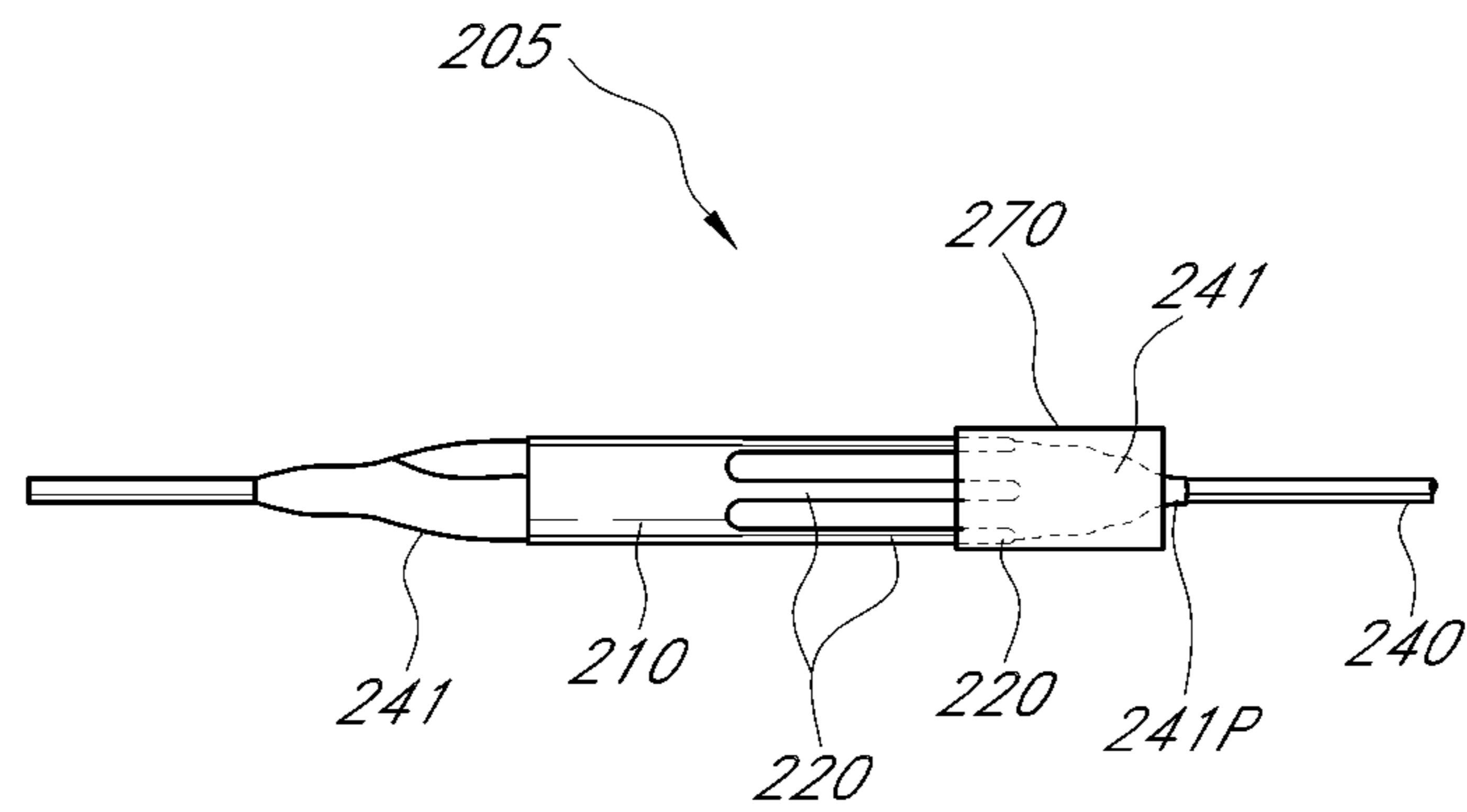
FIG. 8A
