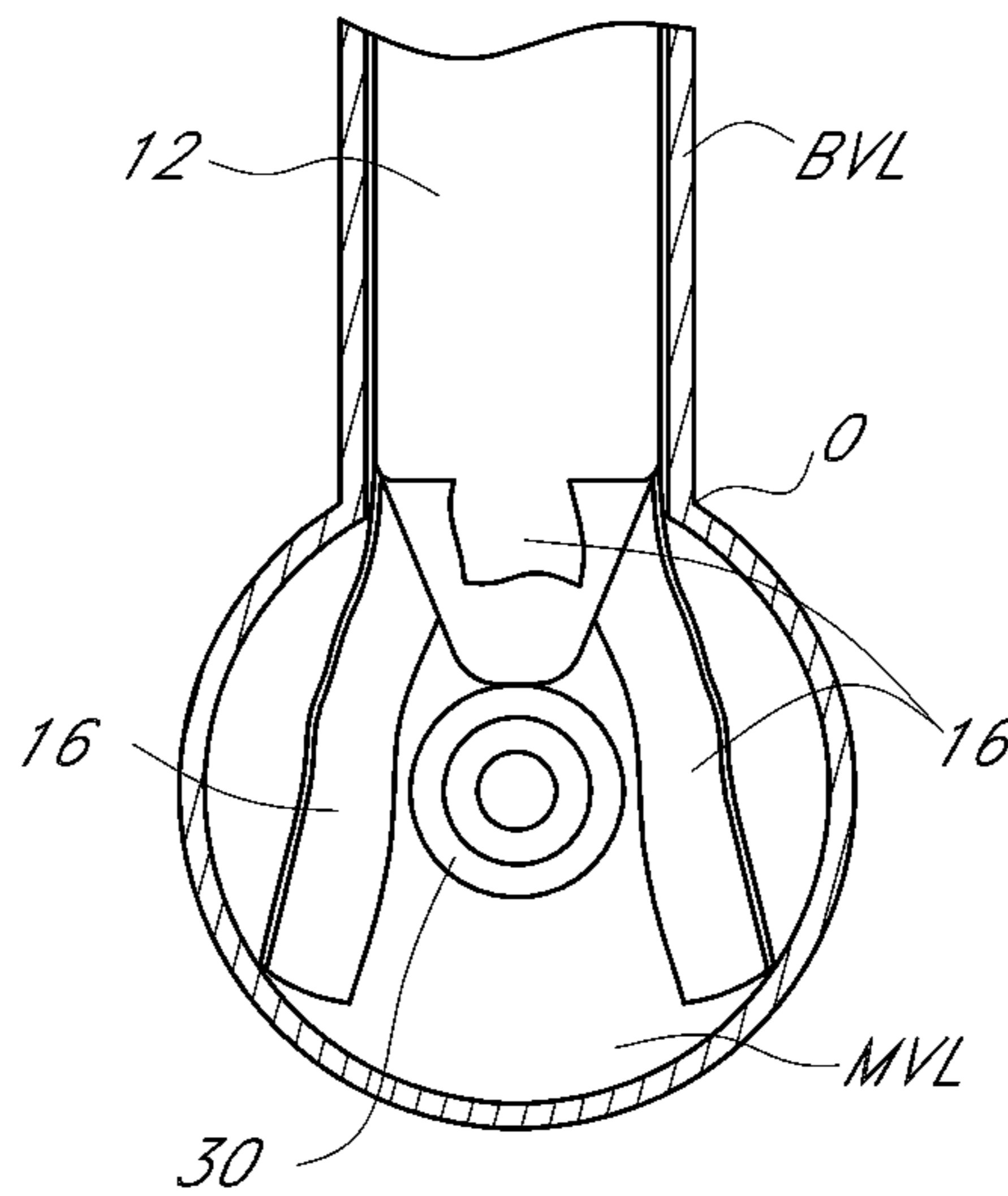
FIG. 10B
