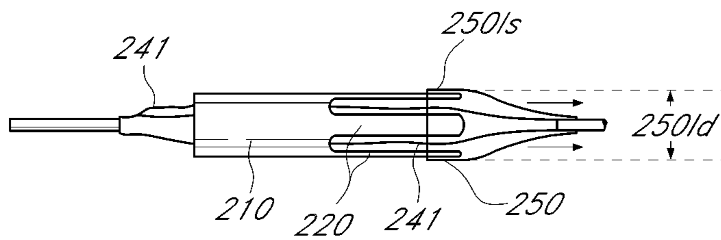
FIG. 5C
