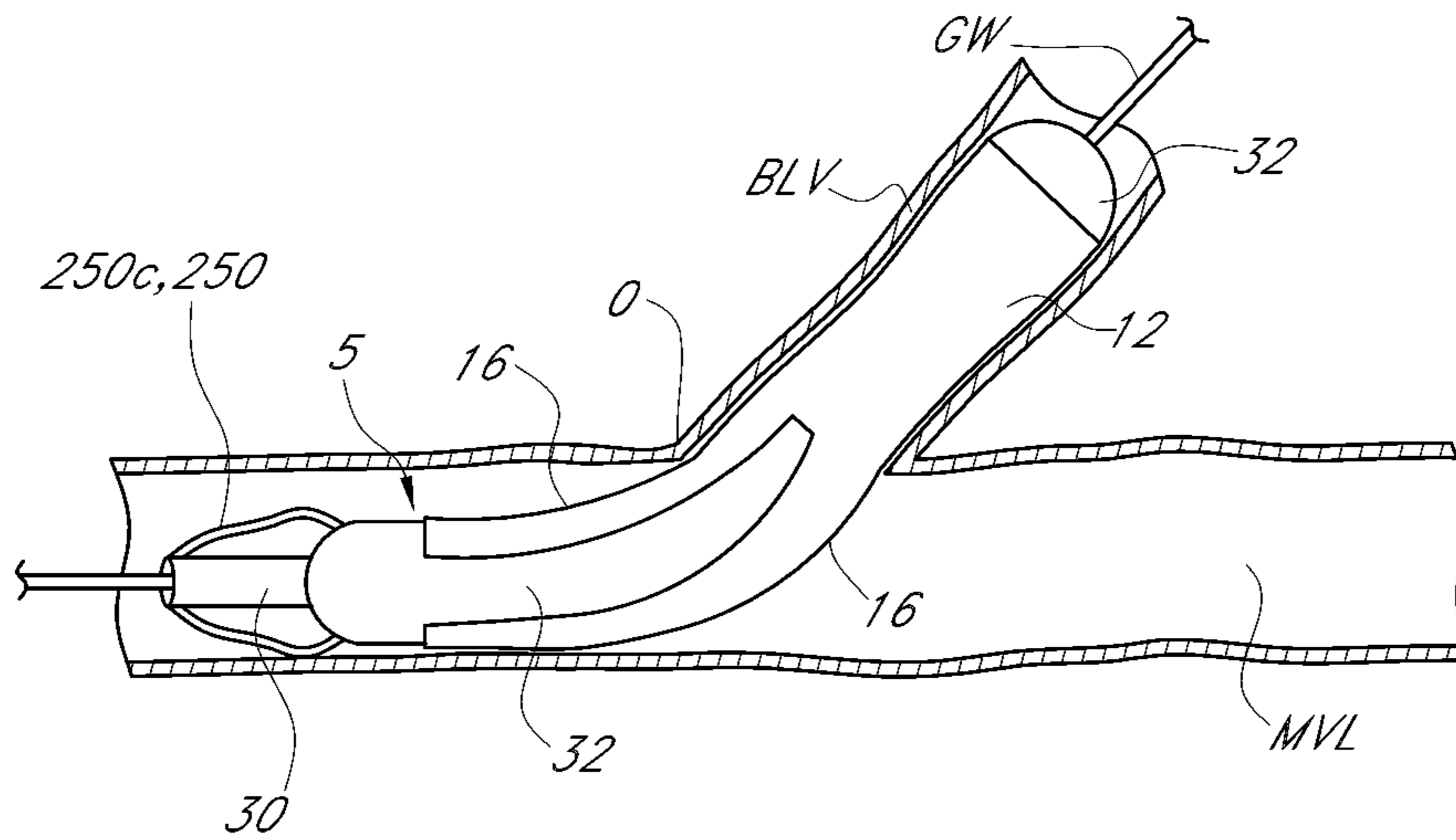
FIG. 10A
