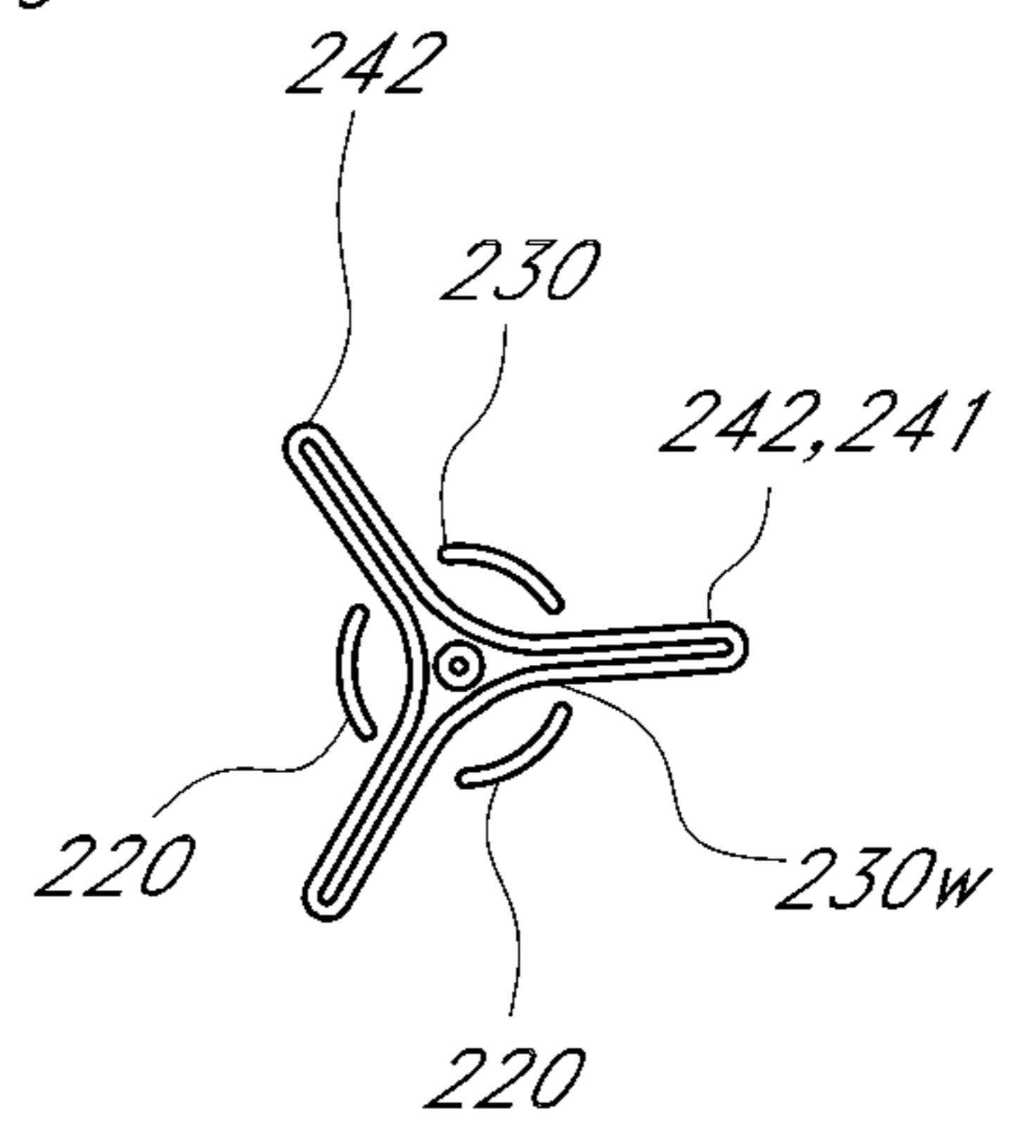
FIG. 3B
