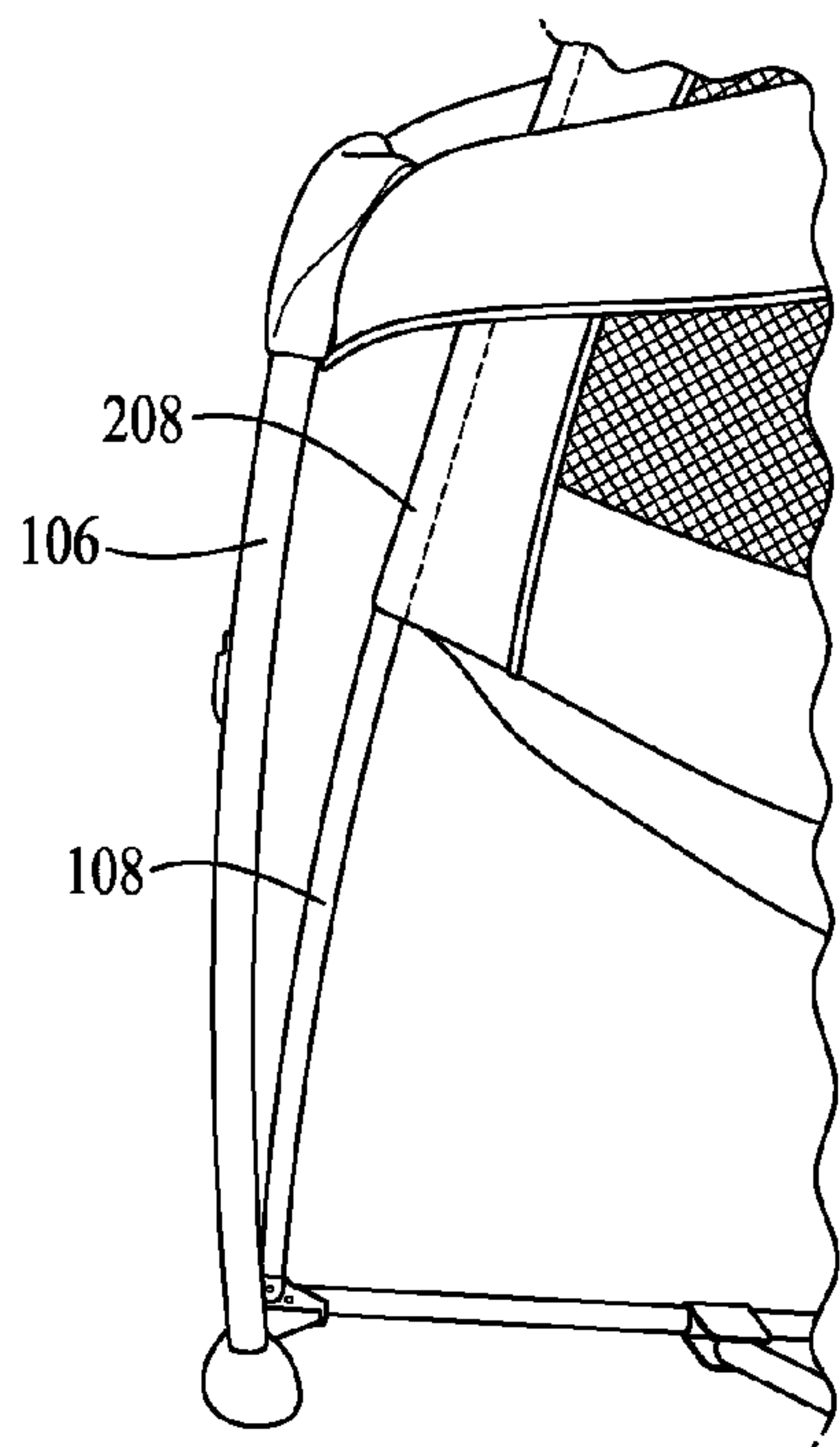
FIG. 13
