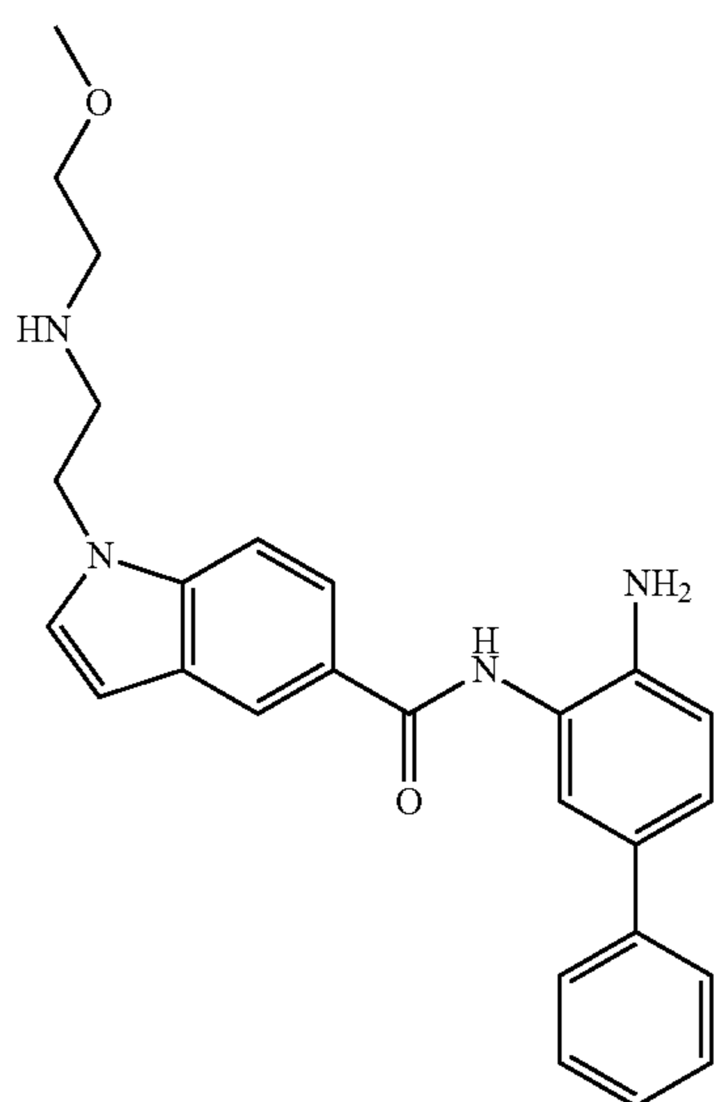
N-(4-amino-[1,1'-biphenyl]-3-yl)-1-(2-((2-methoxyethyl)amino)ethyl)-1H-indole-5-carboxamide
