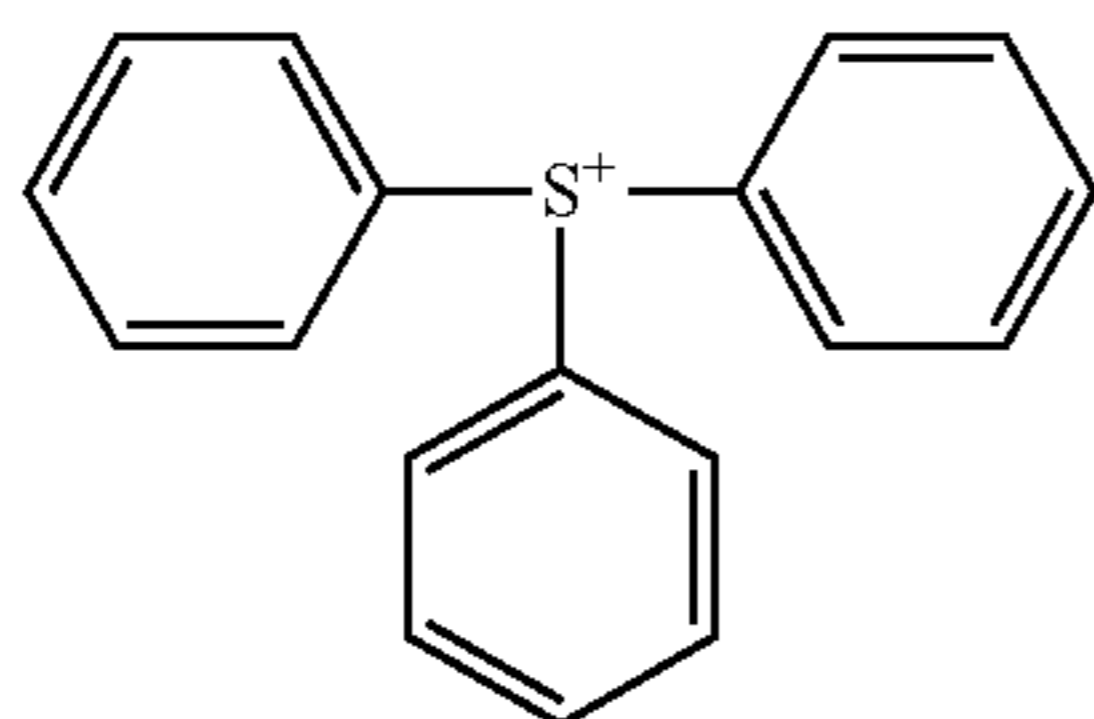
PAG Monomer 2
