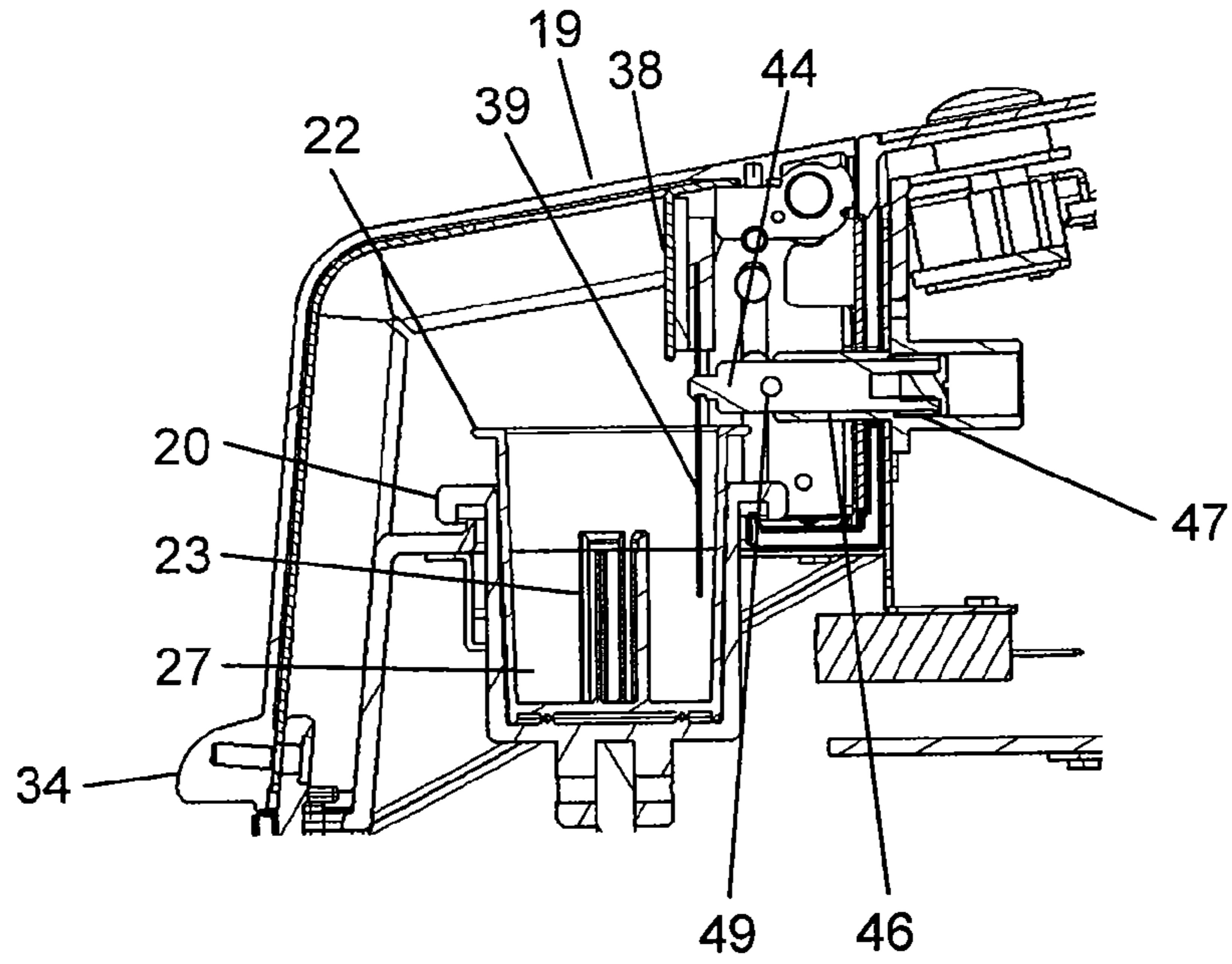
FIG. 33A
