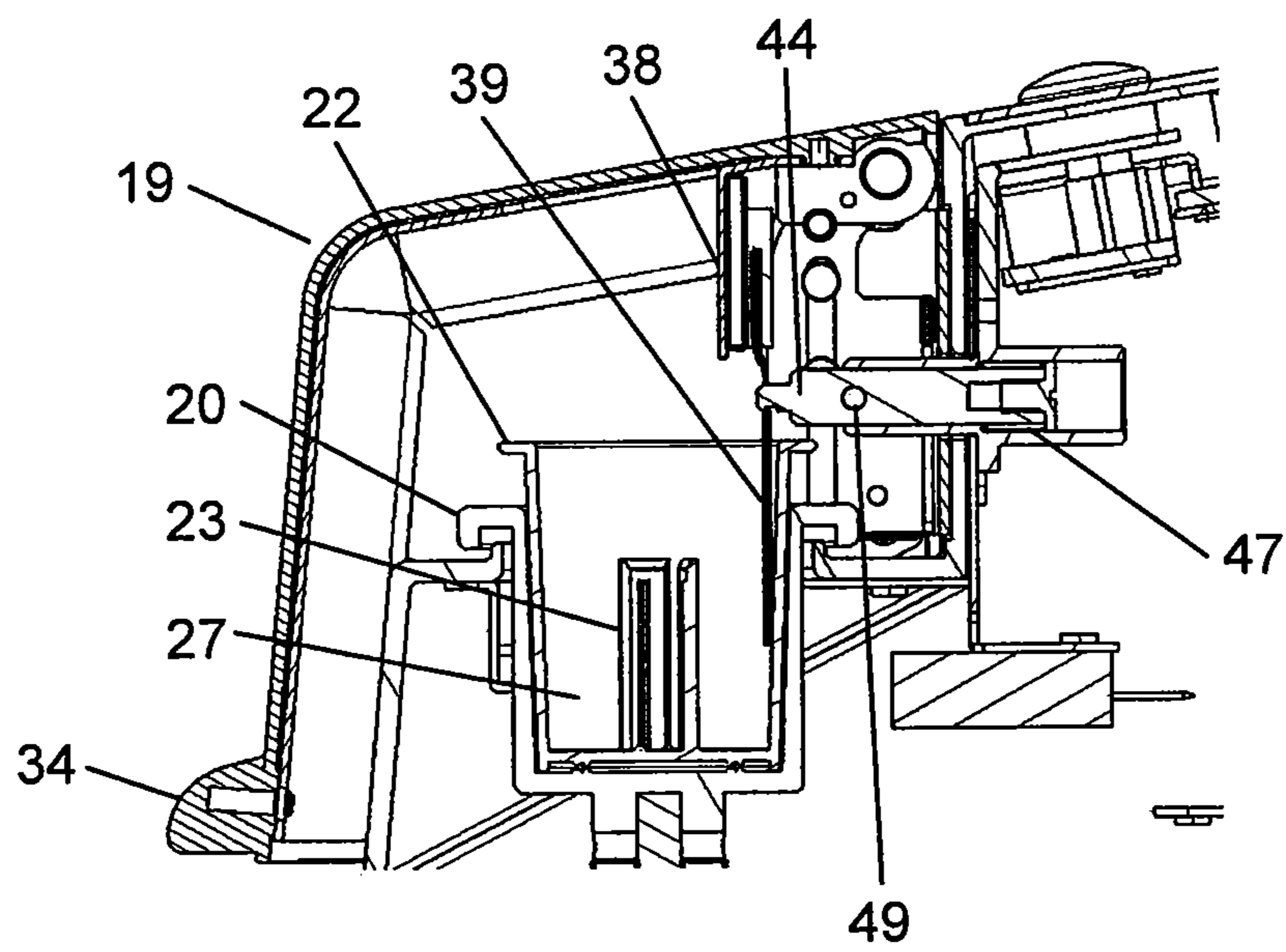
FIG. 36B
