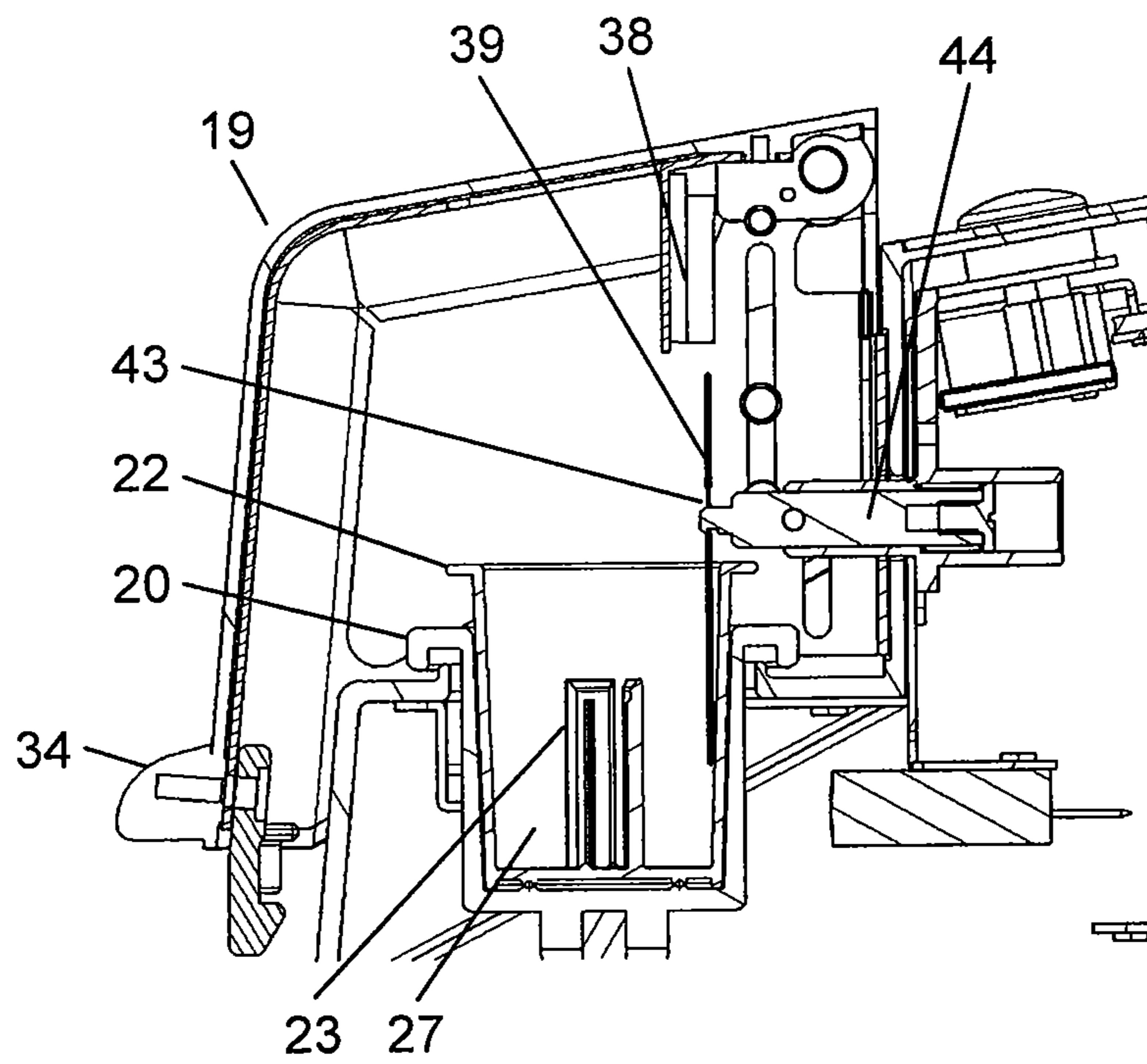
FIG. 37
