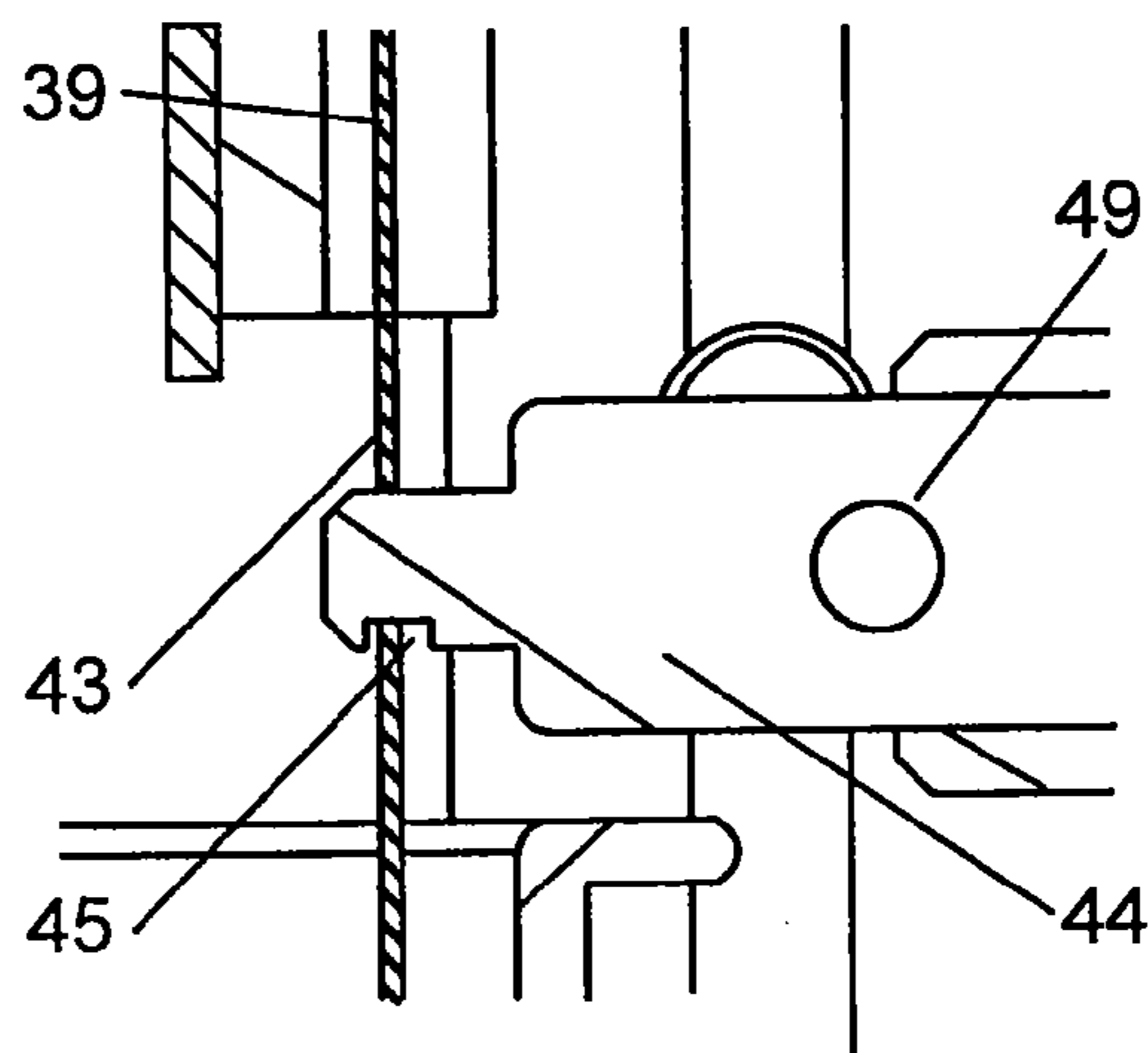
FIG. 33C
