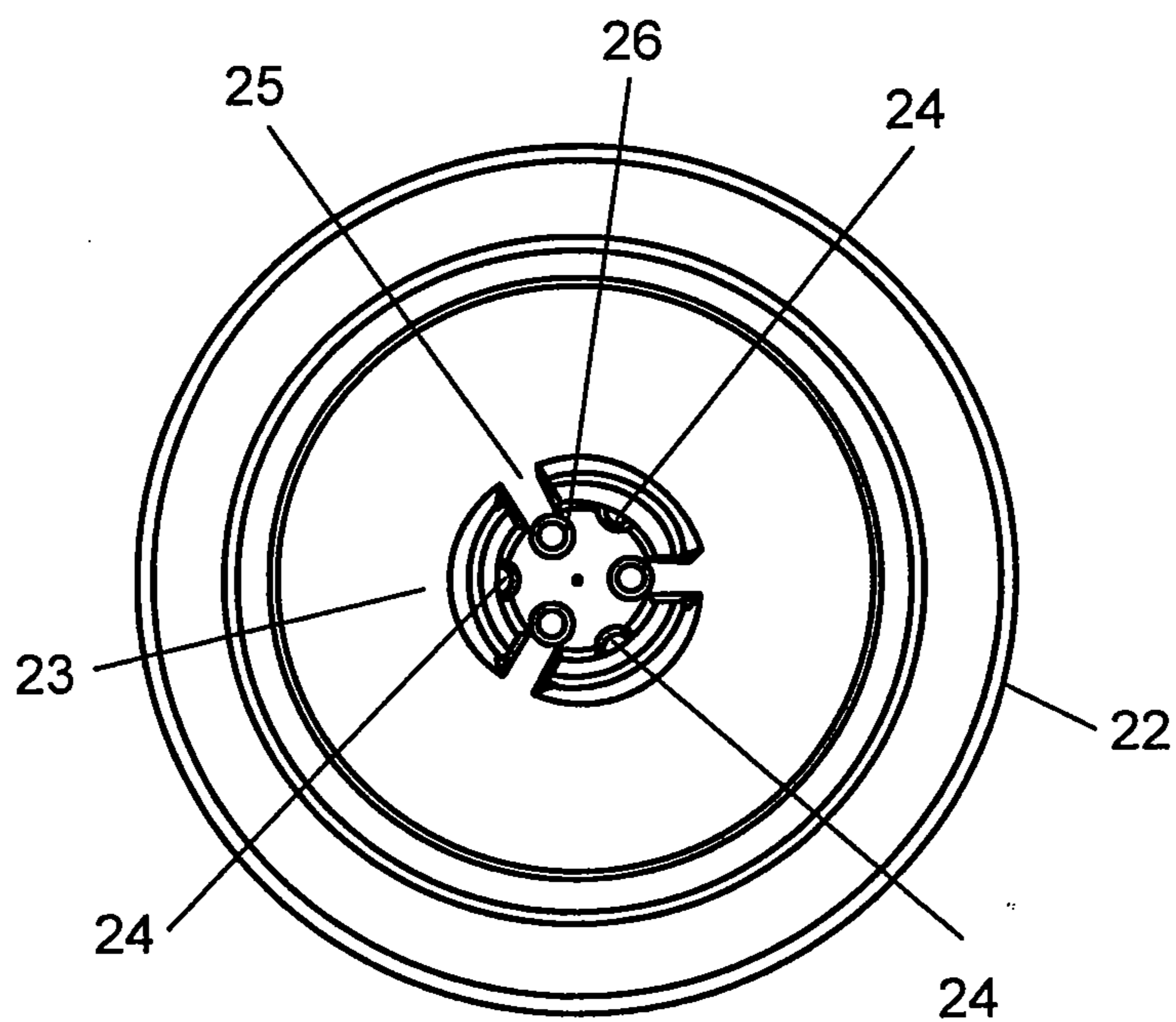
FIG. 21B
