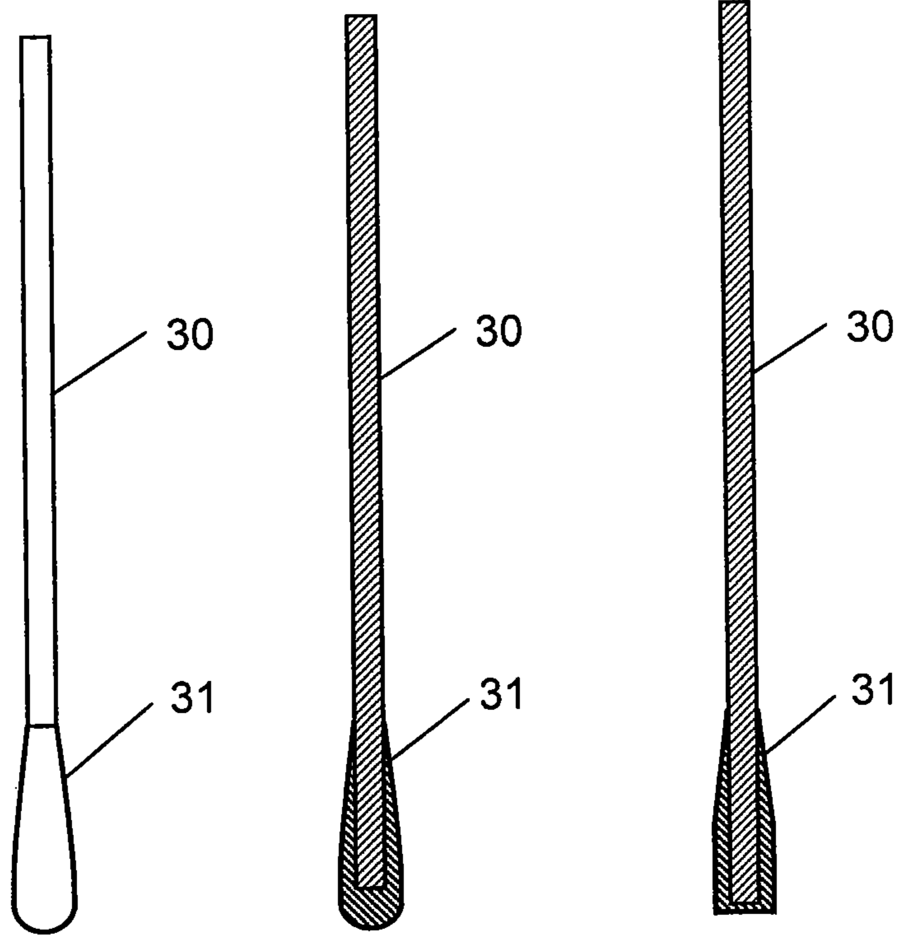
FIG. 20A
