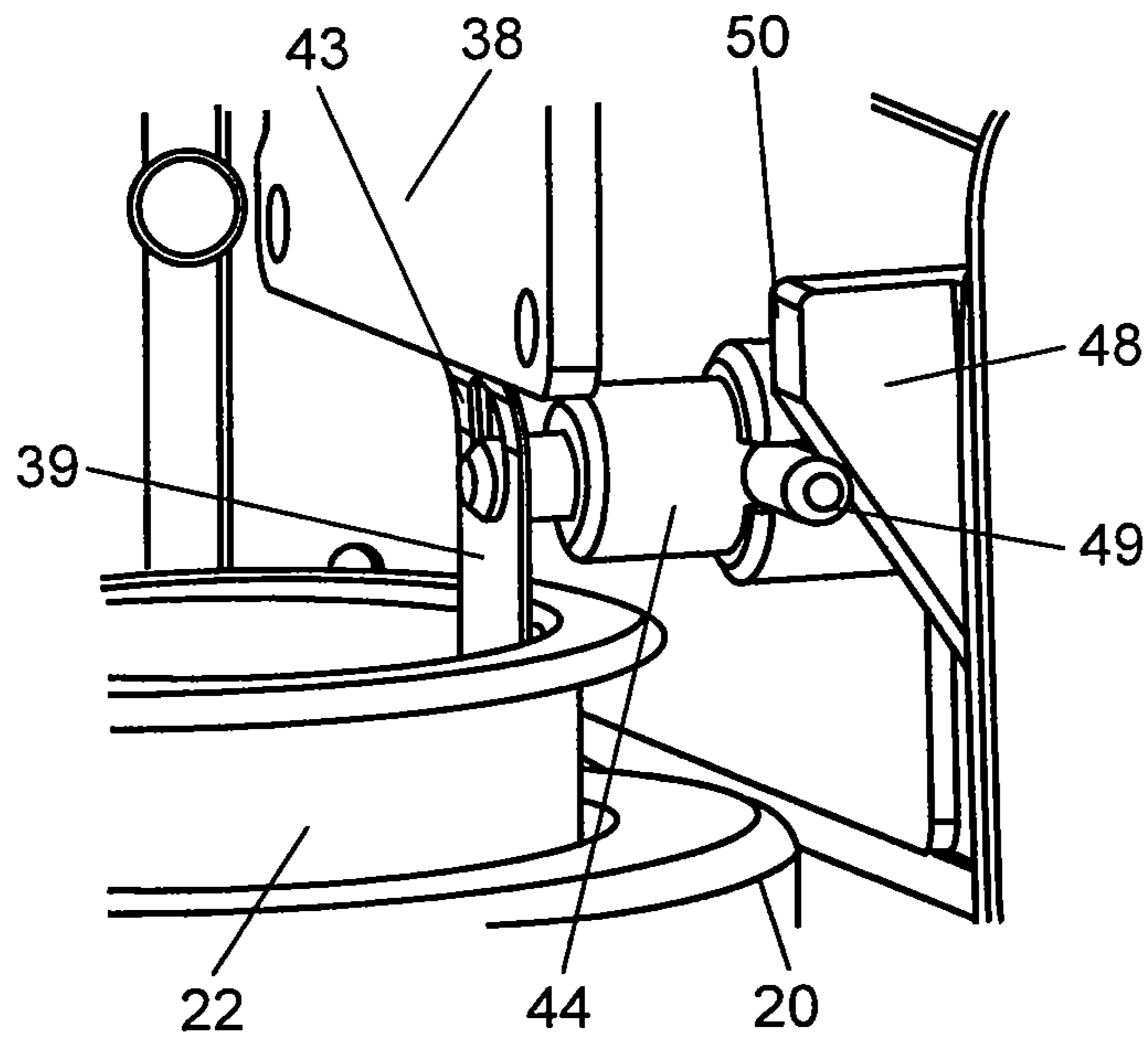
FIG. 36A
