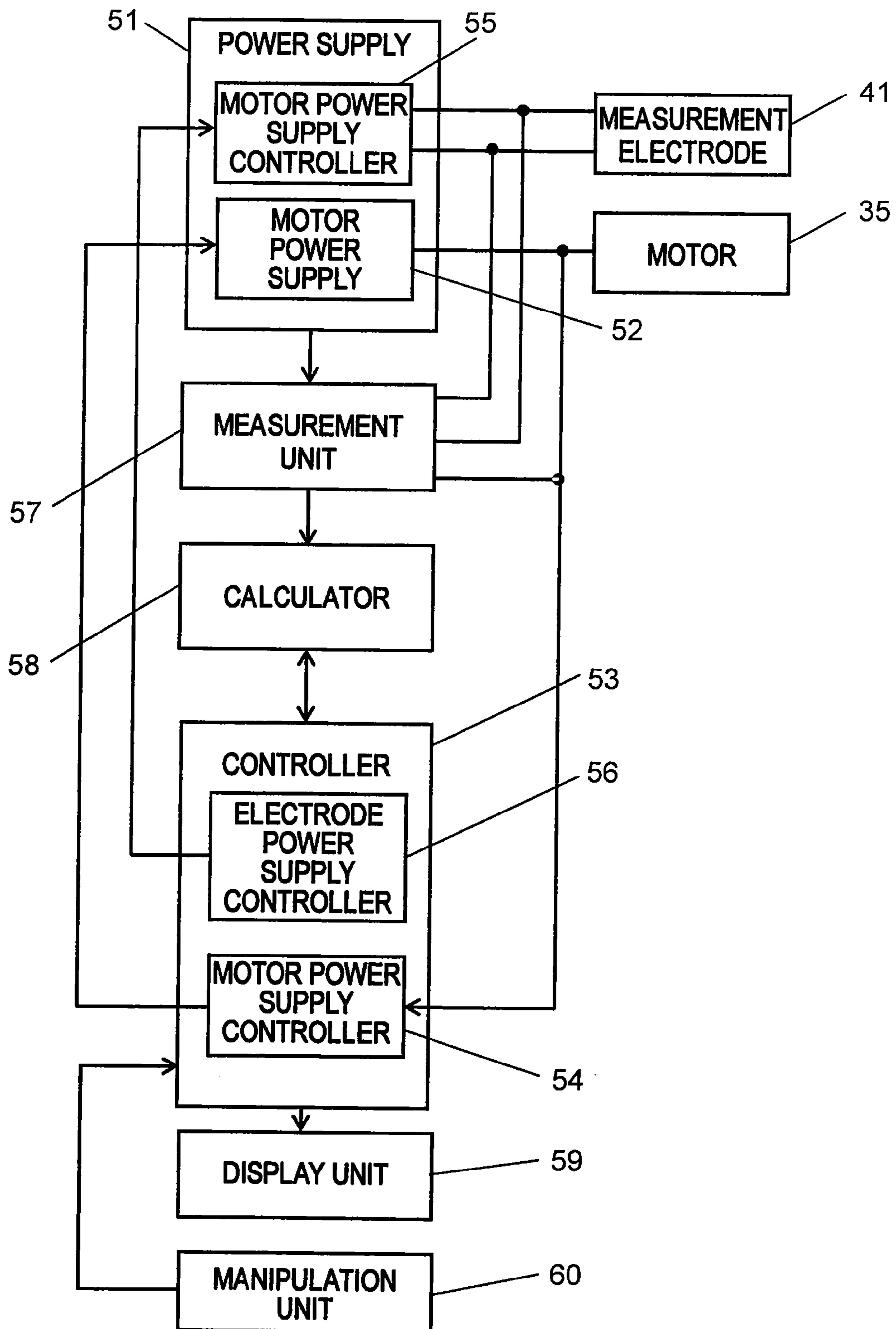
FIG. 34
