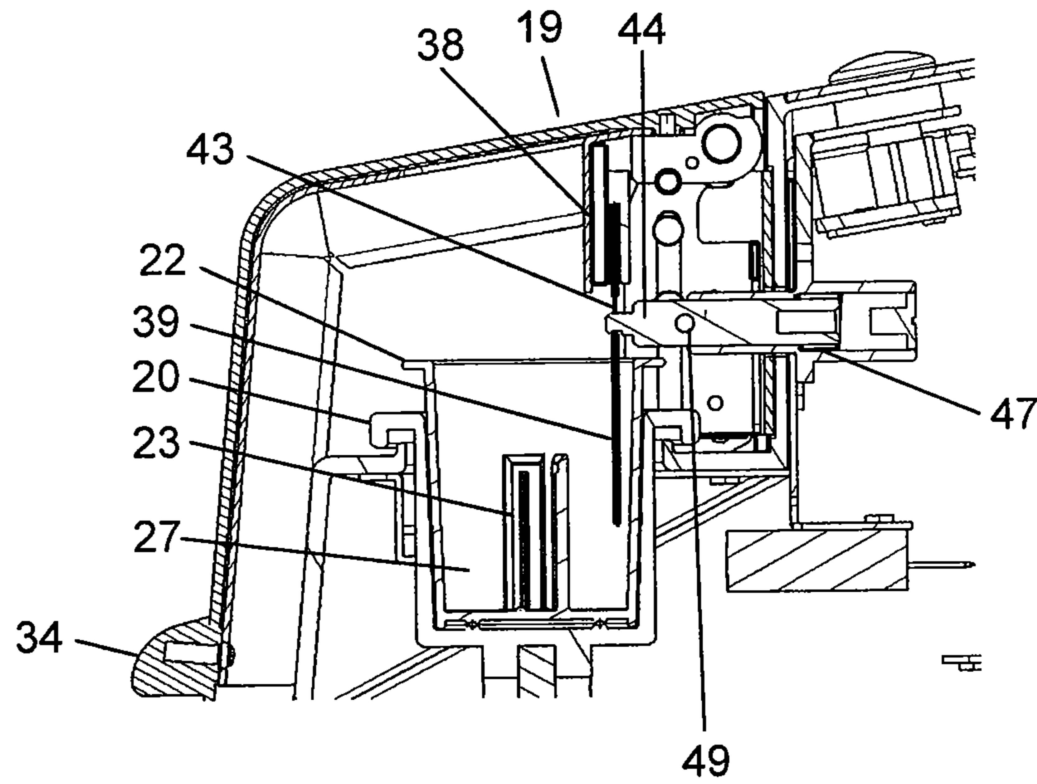
FIG. 35A
