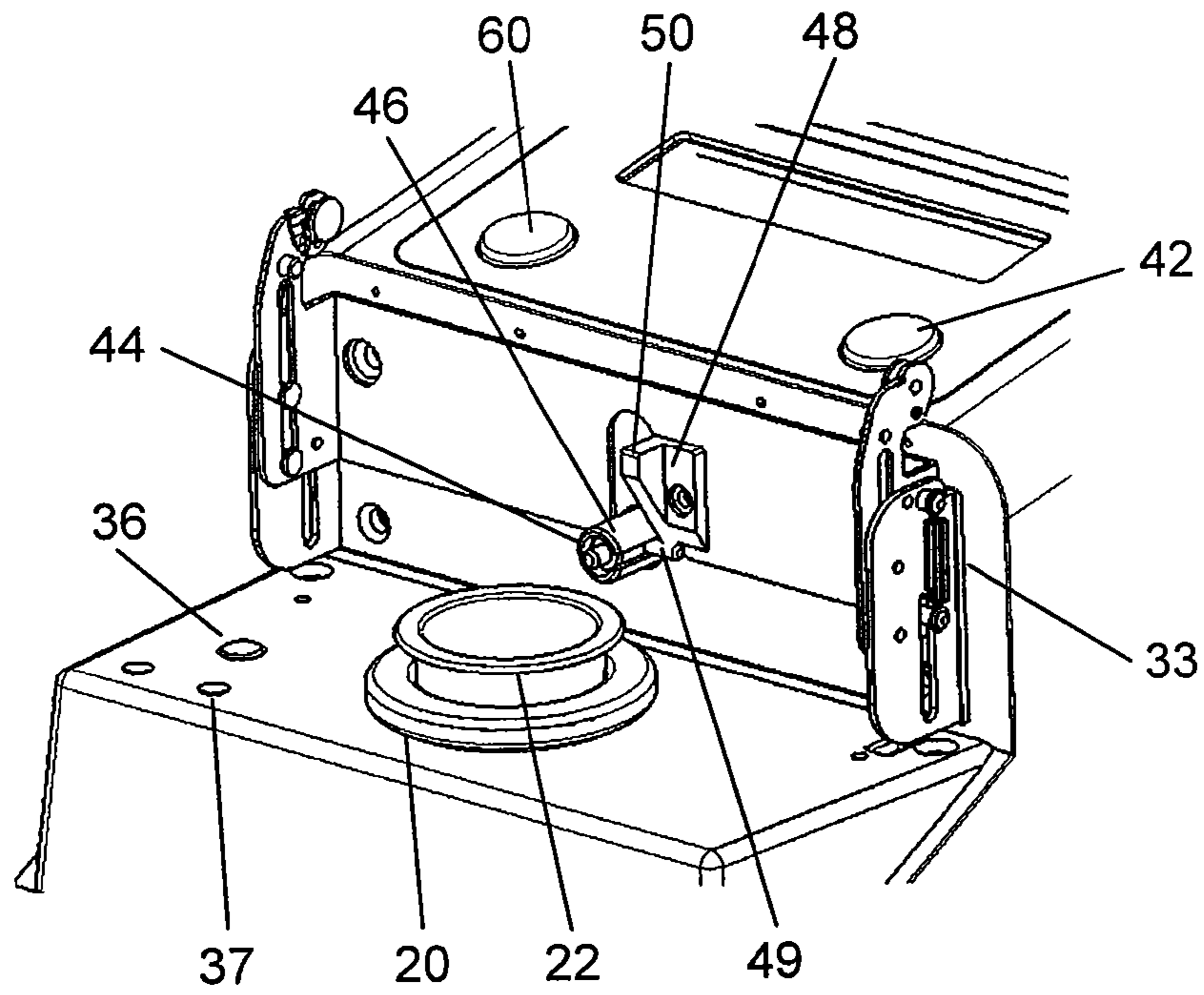
FIG. 31
