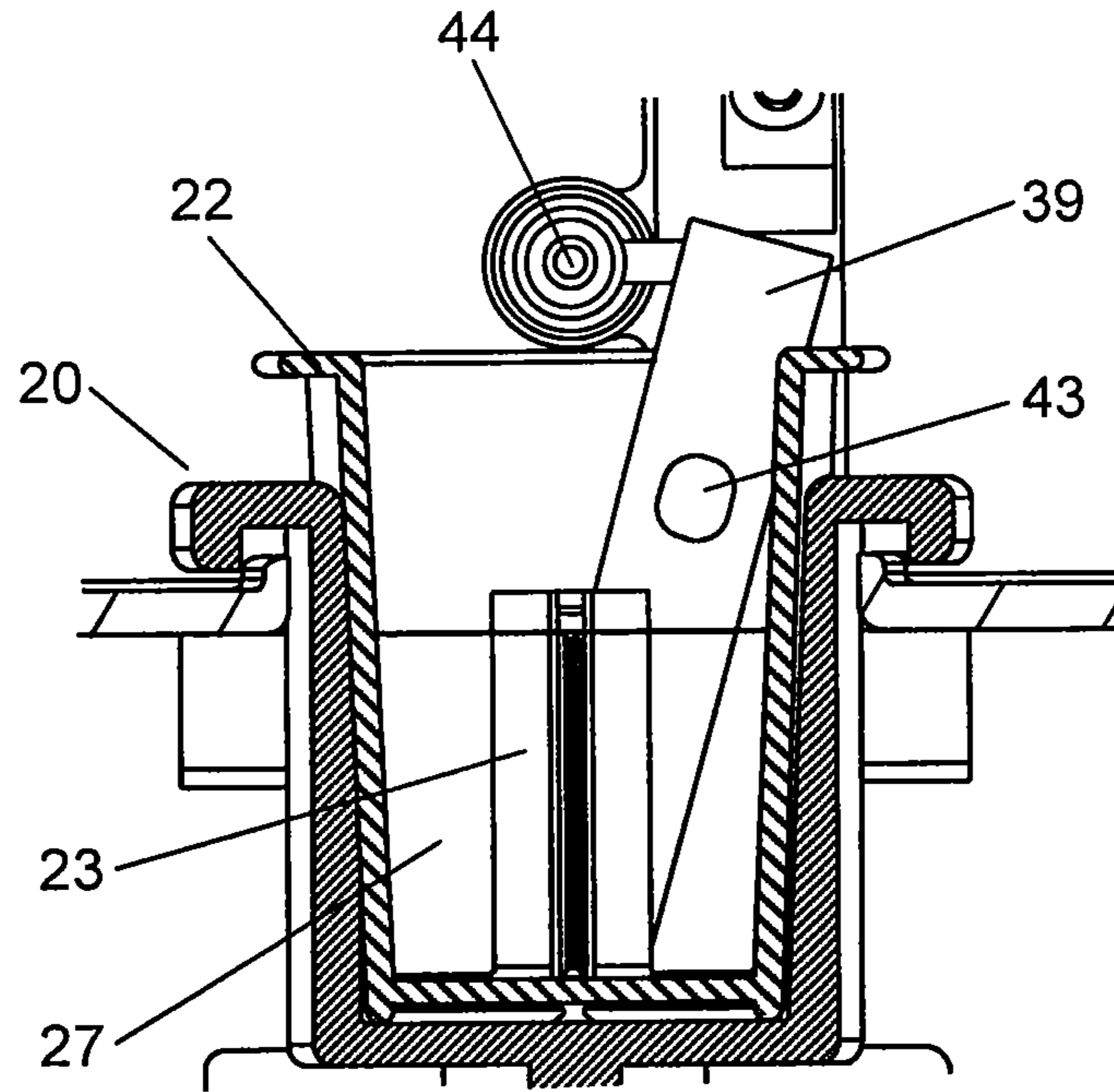
FIG. 38A
