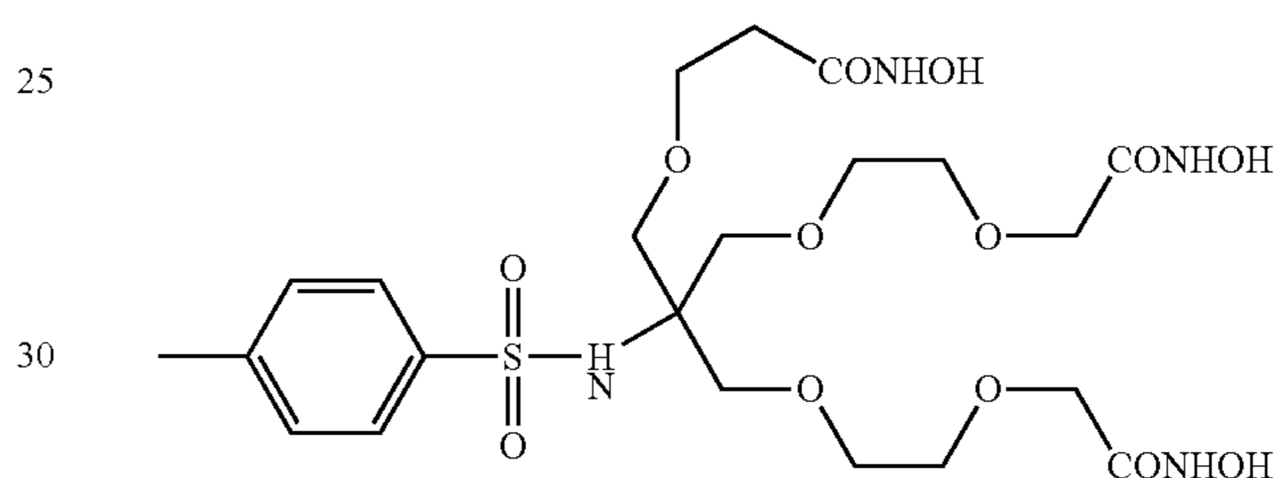
Ligand 6
