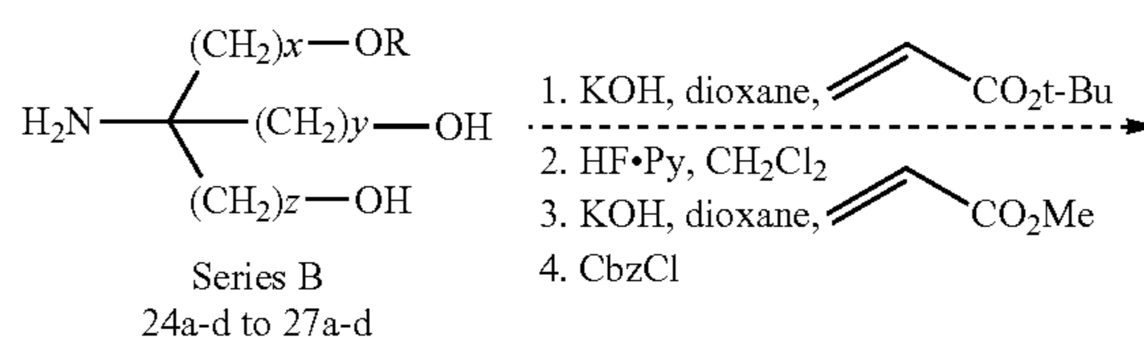
Scheme 29.
