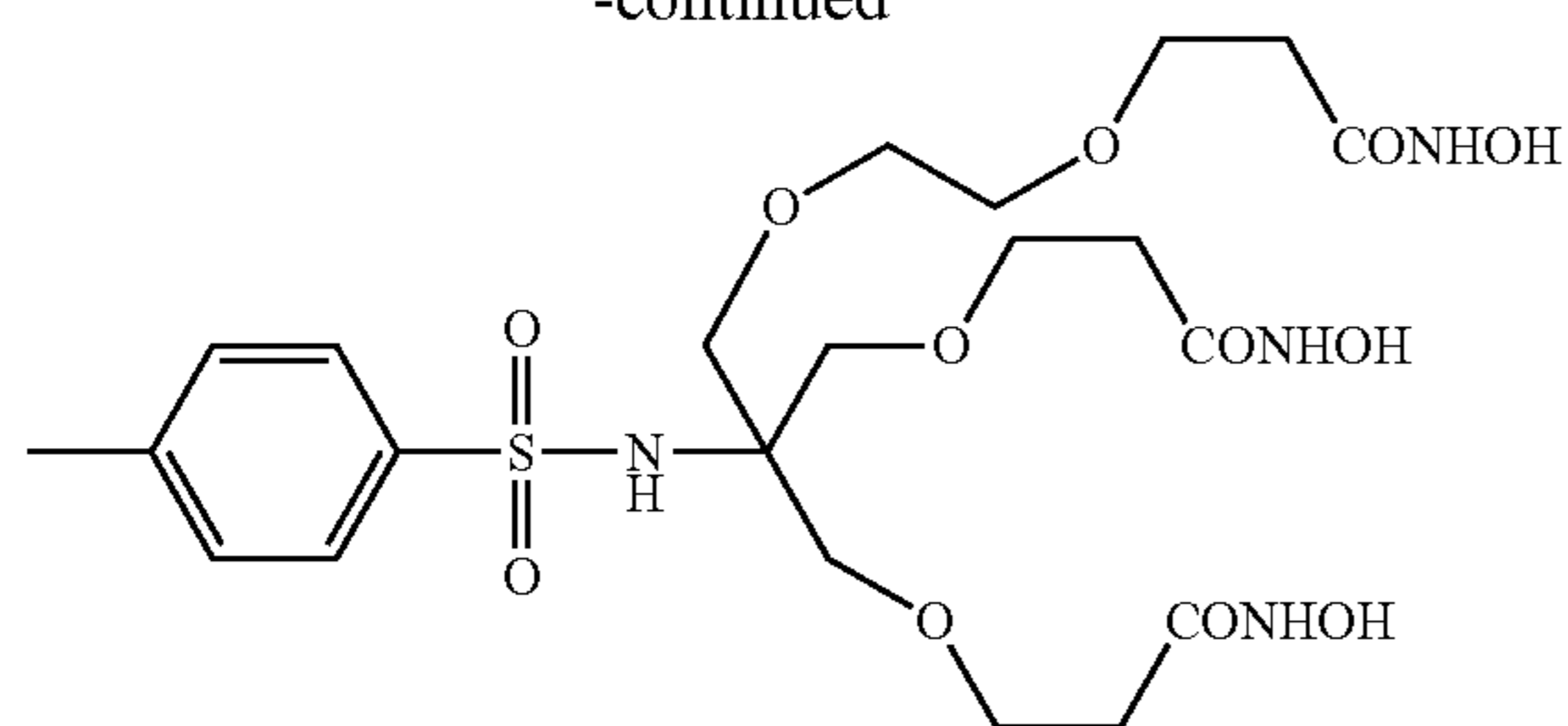
Ligand 5
