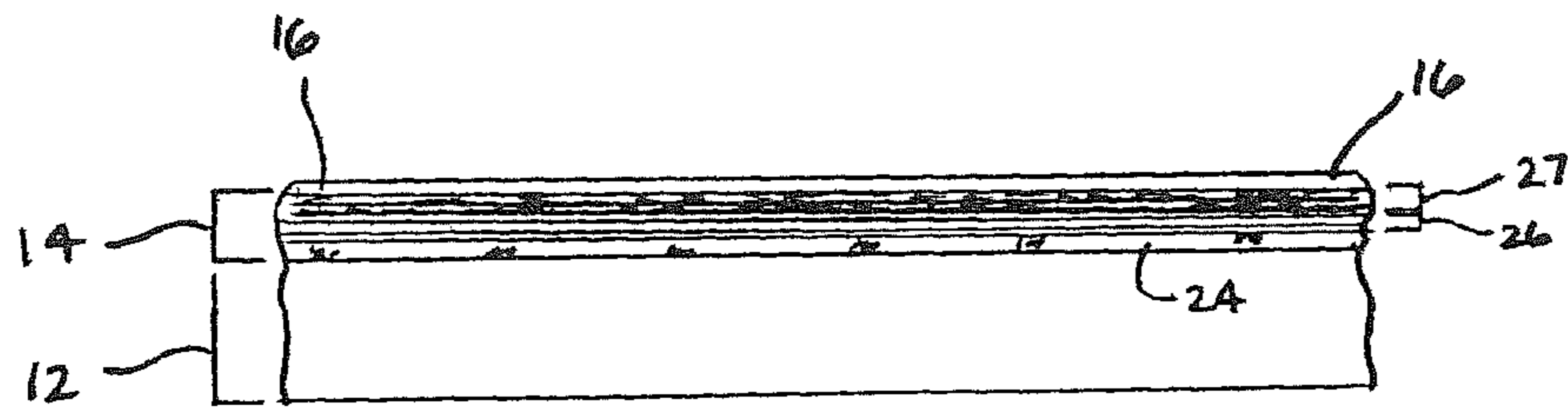
FIG. 6
