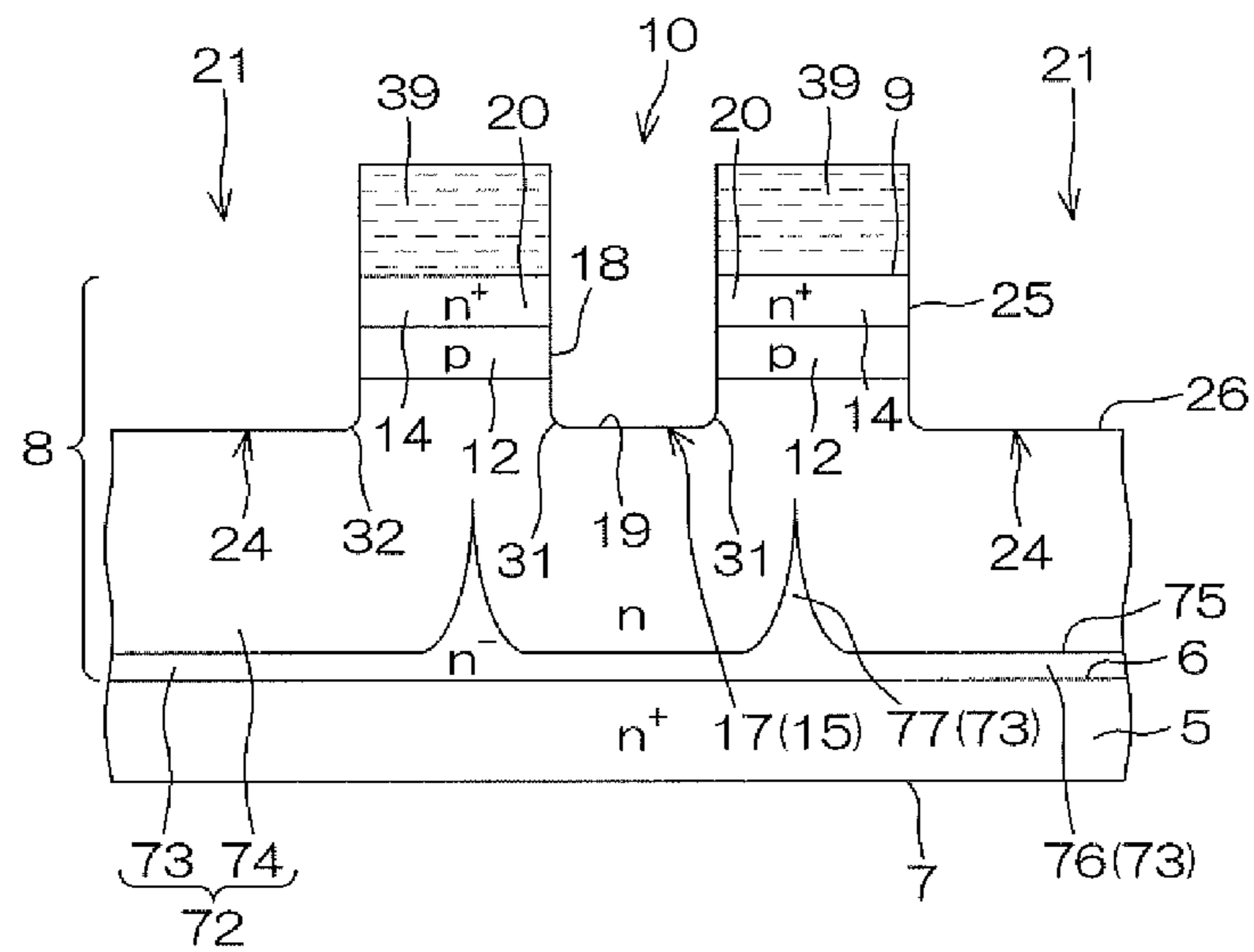
FIG. 8D A-A SECTION
