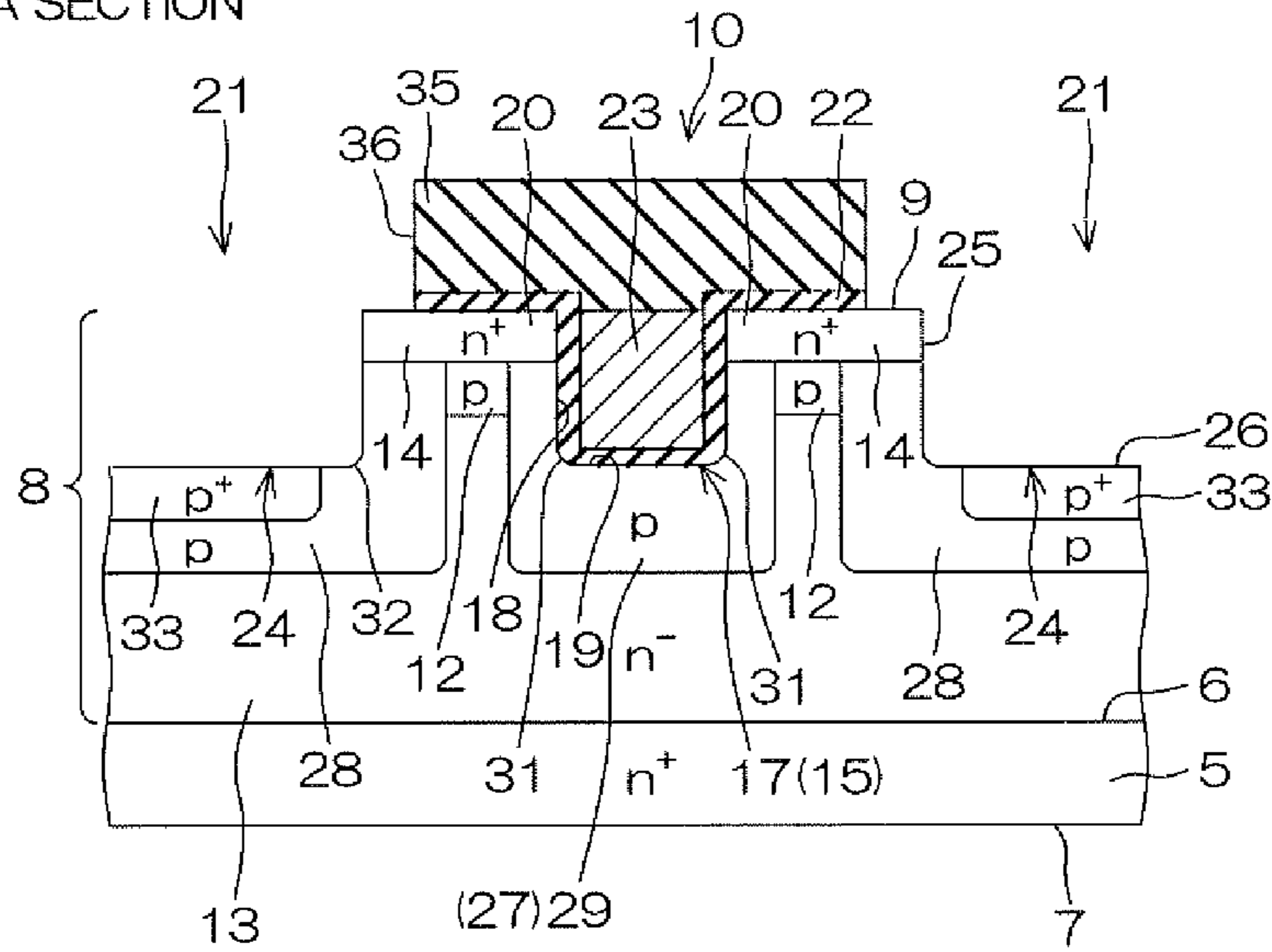
FIG. 3H A-A SECTION
