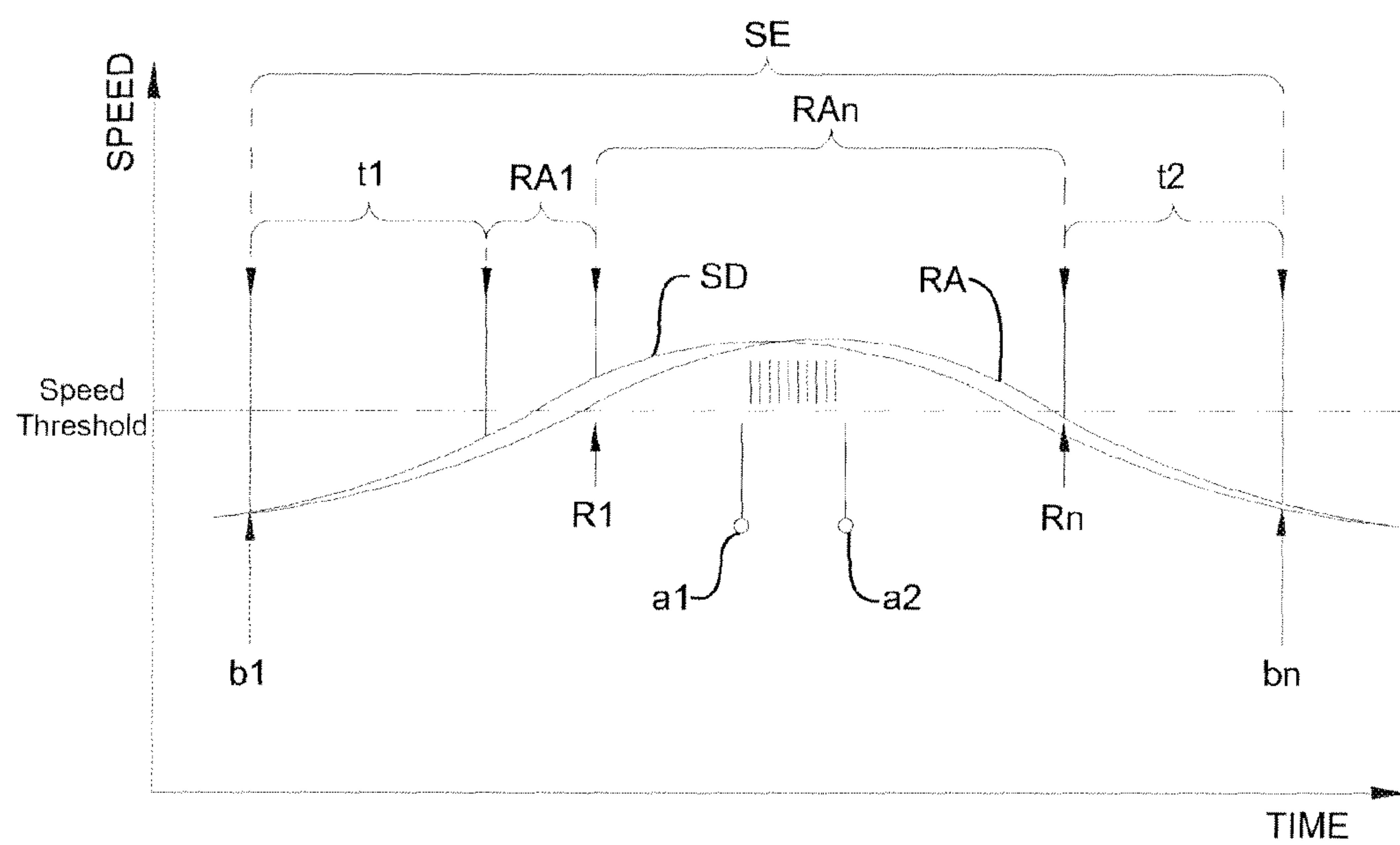
FIG. 8
