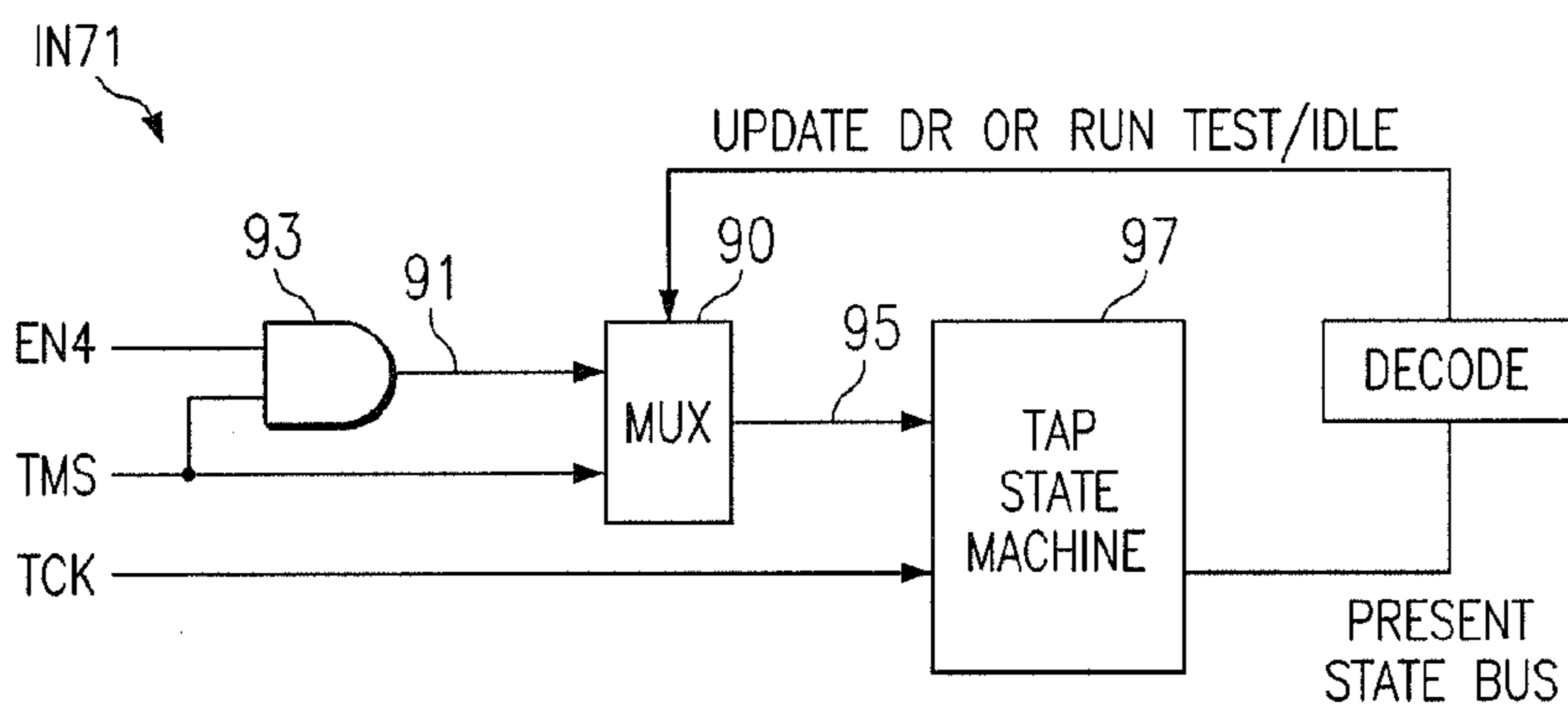
FIG. 9A
