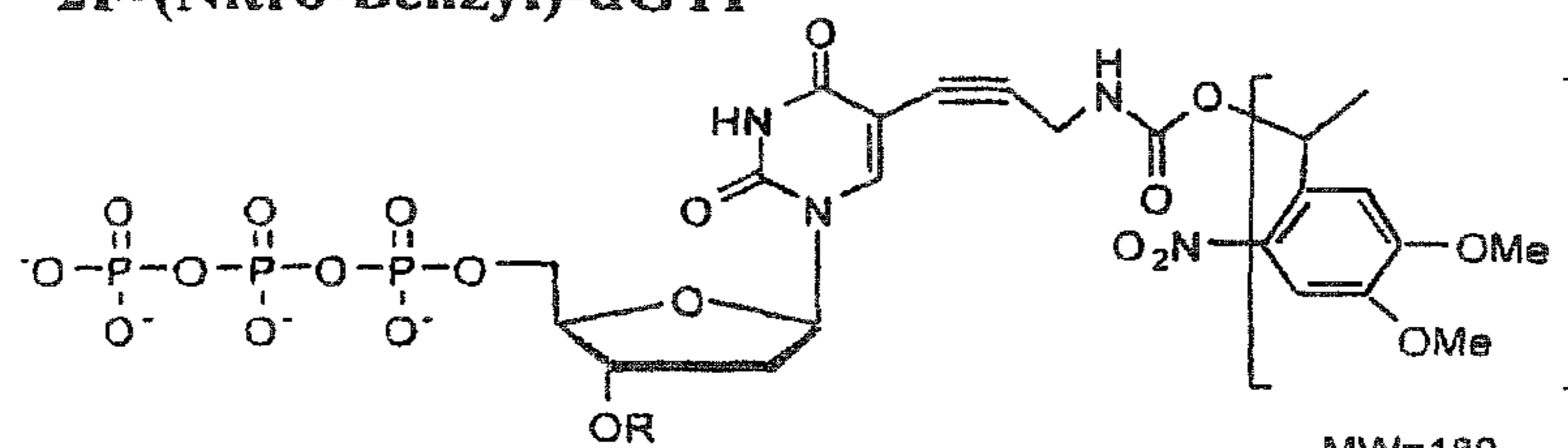
2(Meo)-(Nitro-Benzyl)-dTTP
