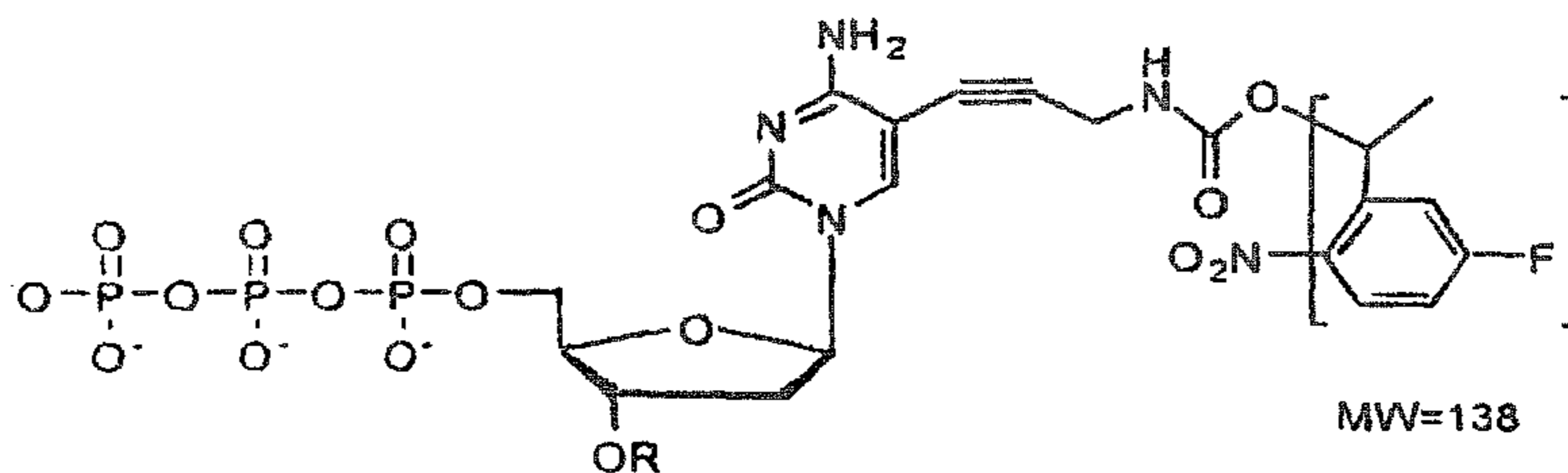
F-(Nitro-Benzyl)-dCTP
