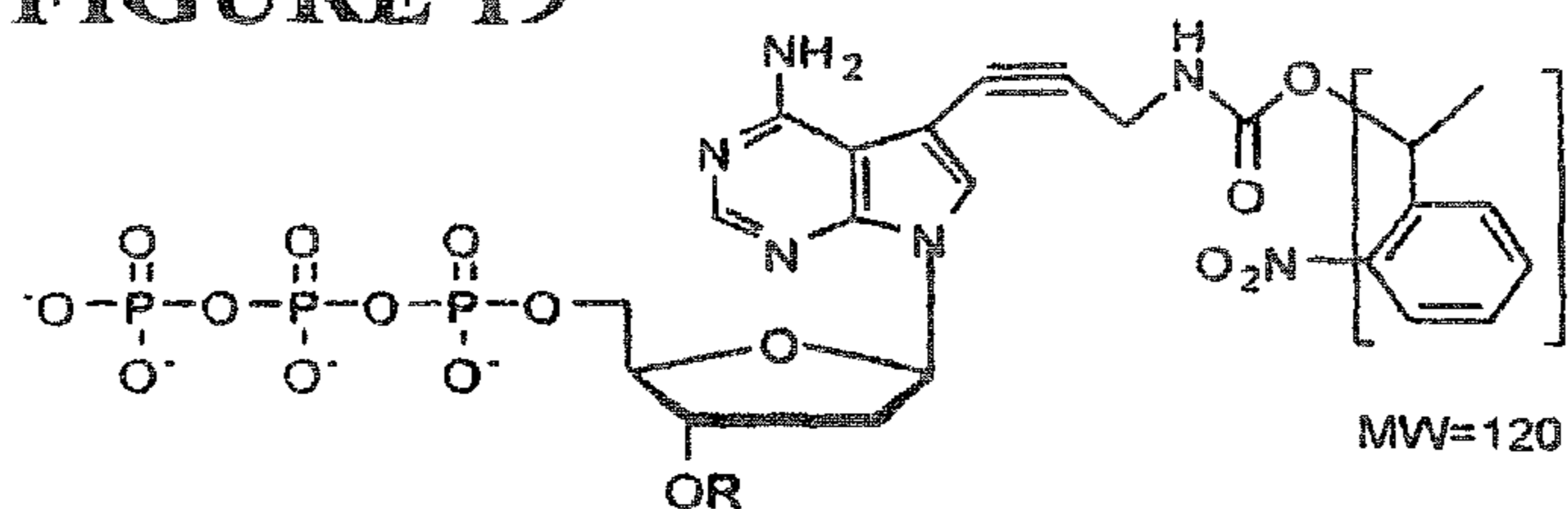
(Nitro-Benzyl)-dATP
