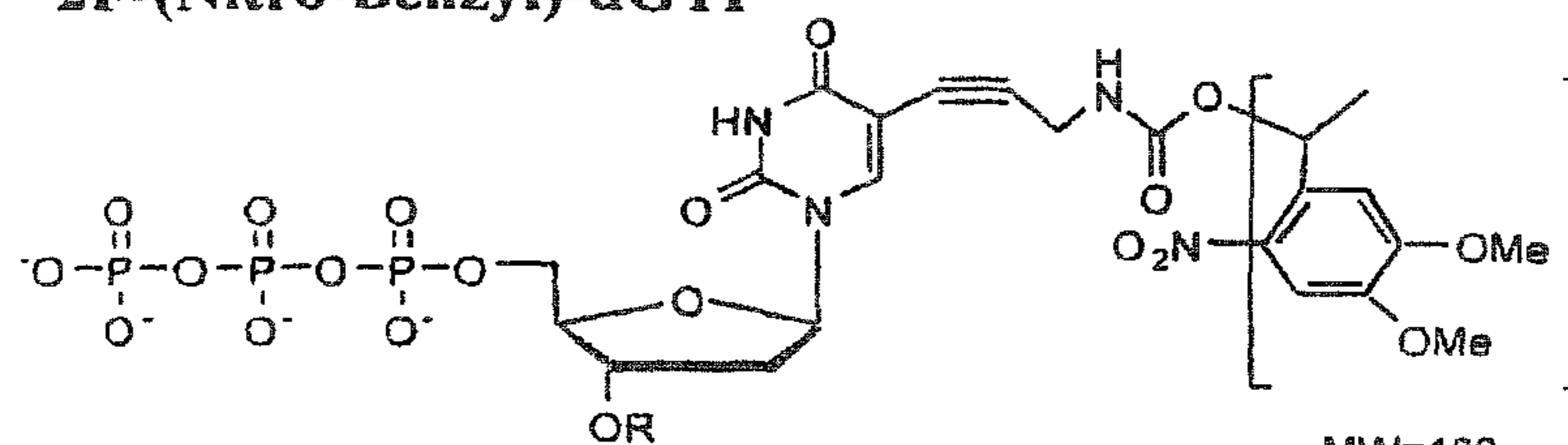
2(Meo)-(Nitro-Benzyl)-dTTP
