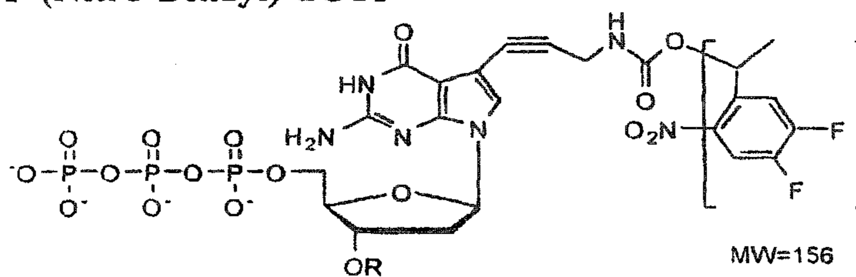
2F-(Nitro-Benzyl)-dGTP
