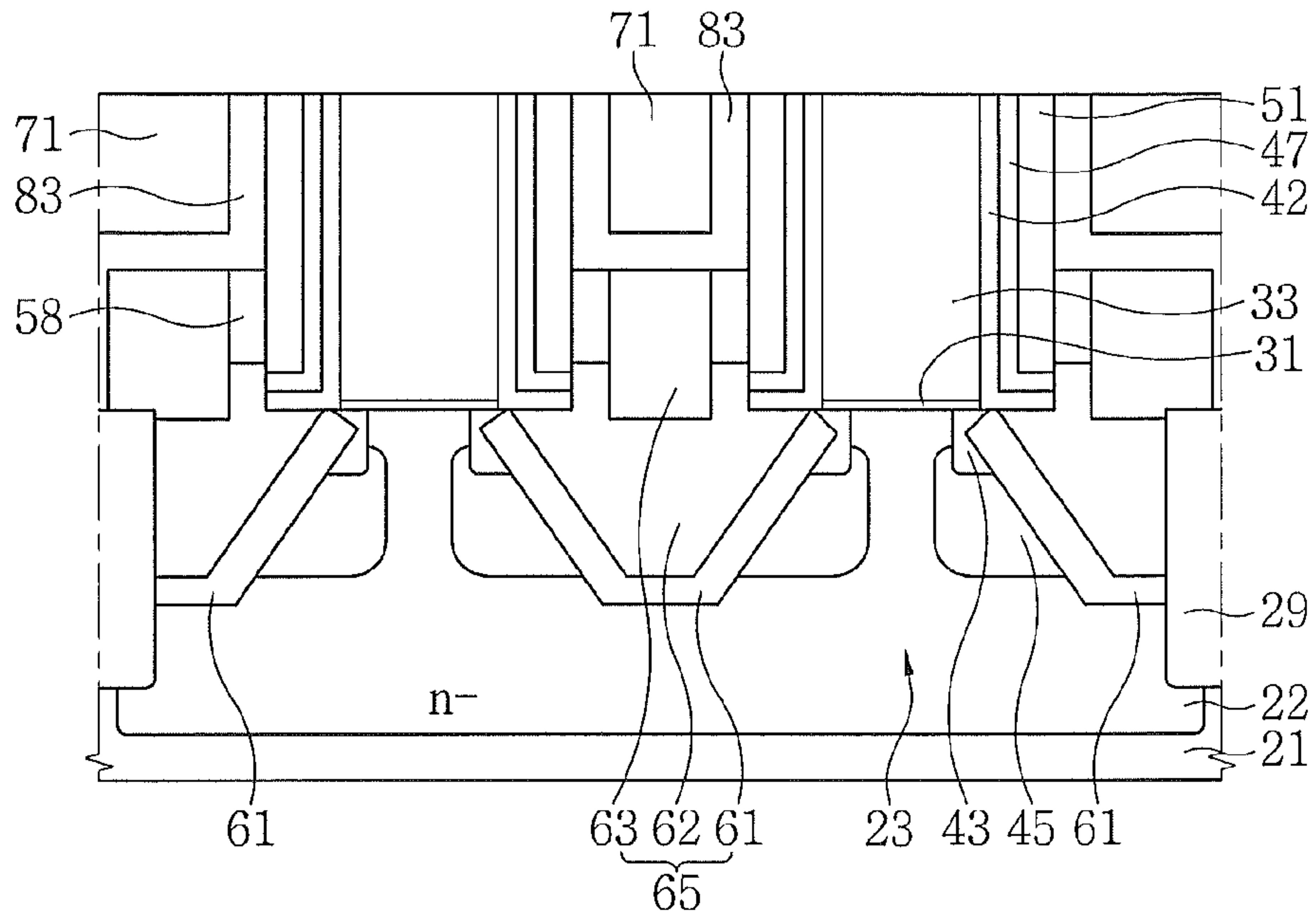
FIG. 20
