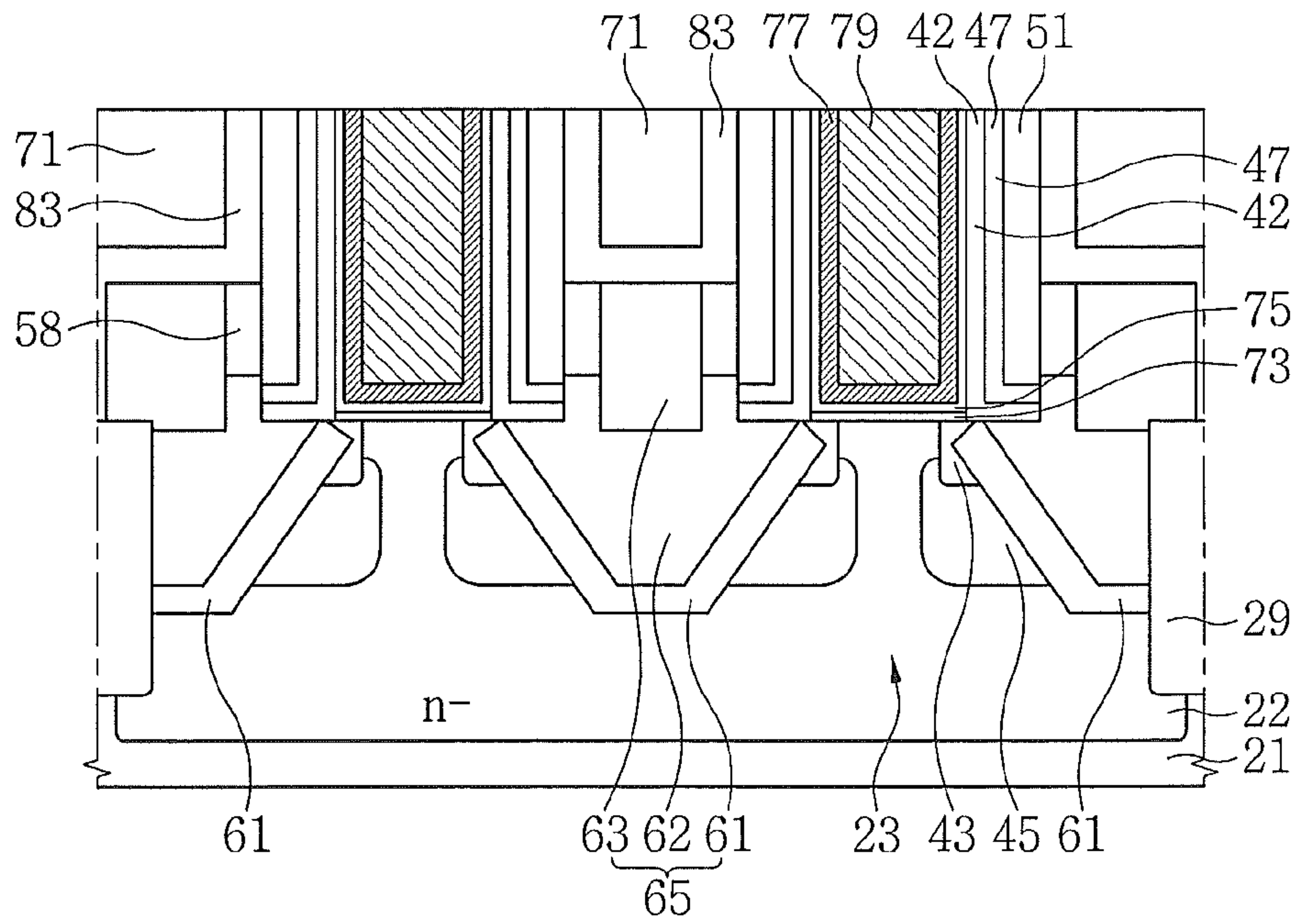
FIG. 21B
