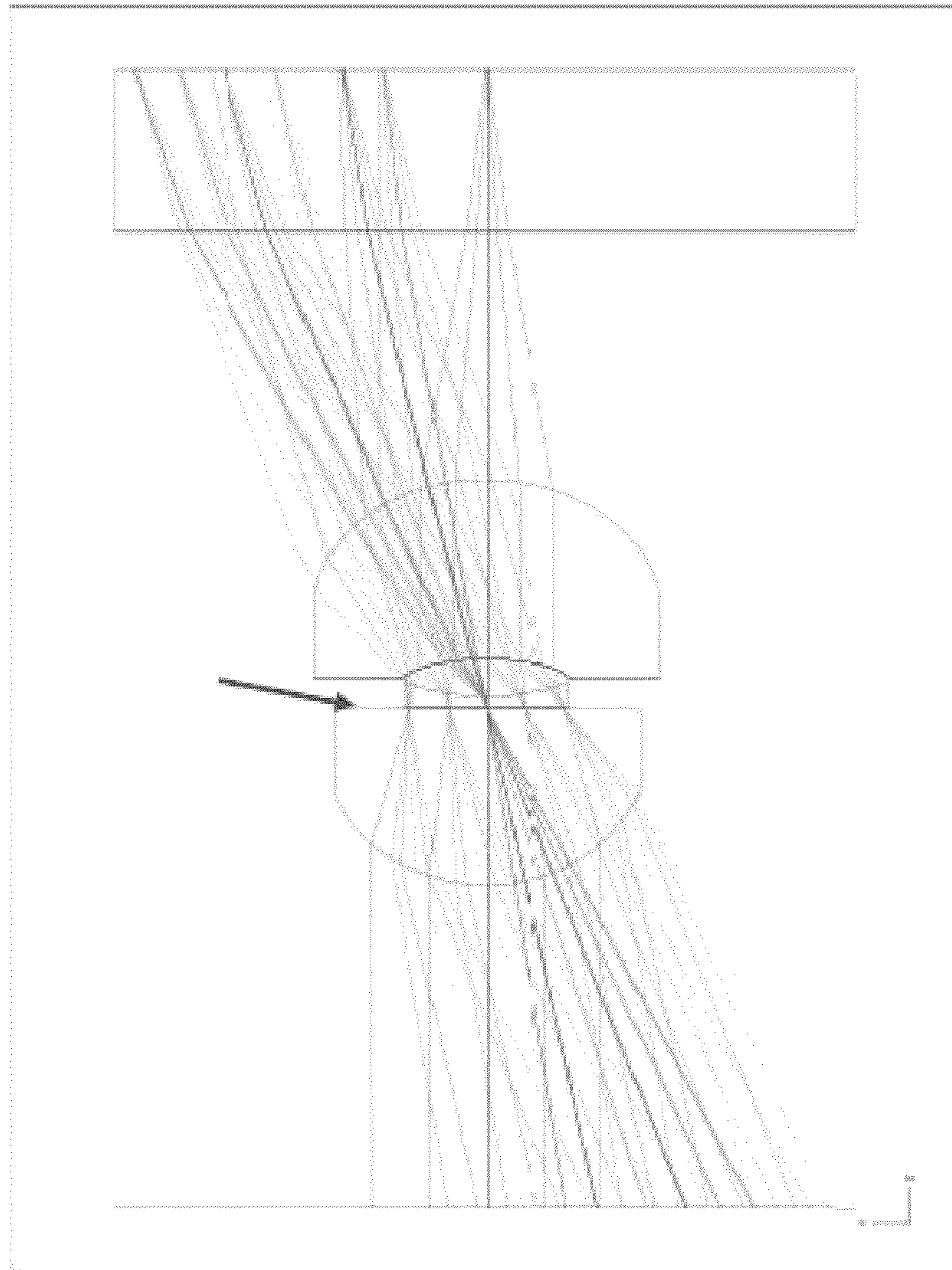
FIG. 7F
