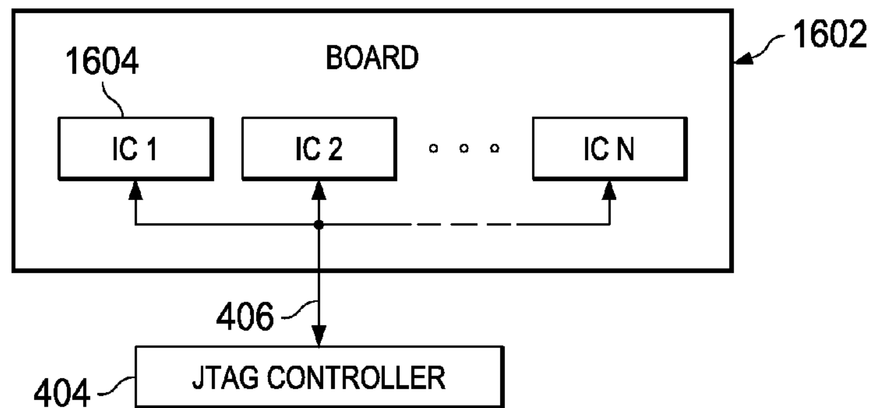
FIG. 16
