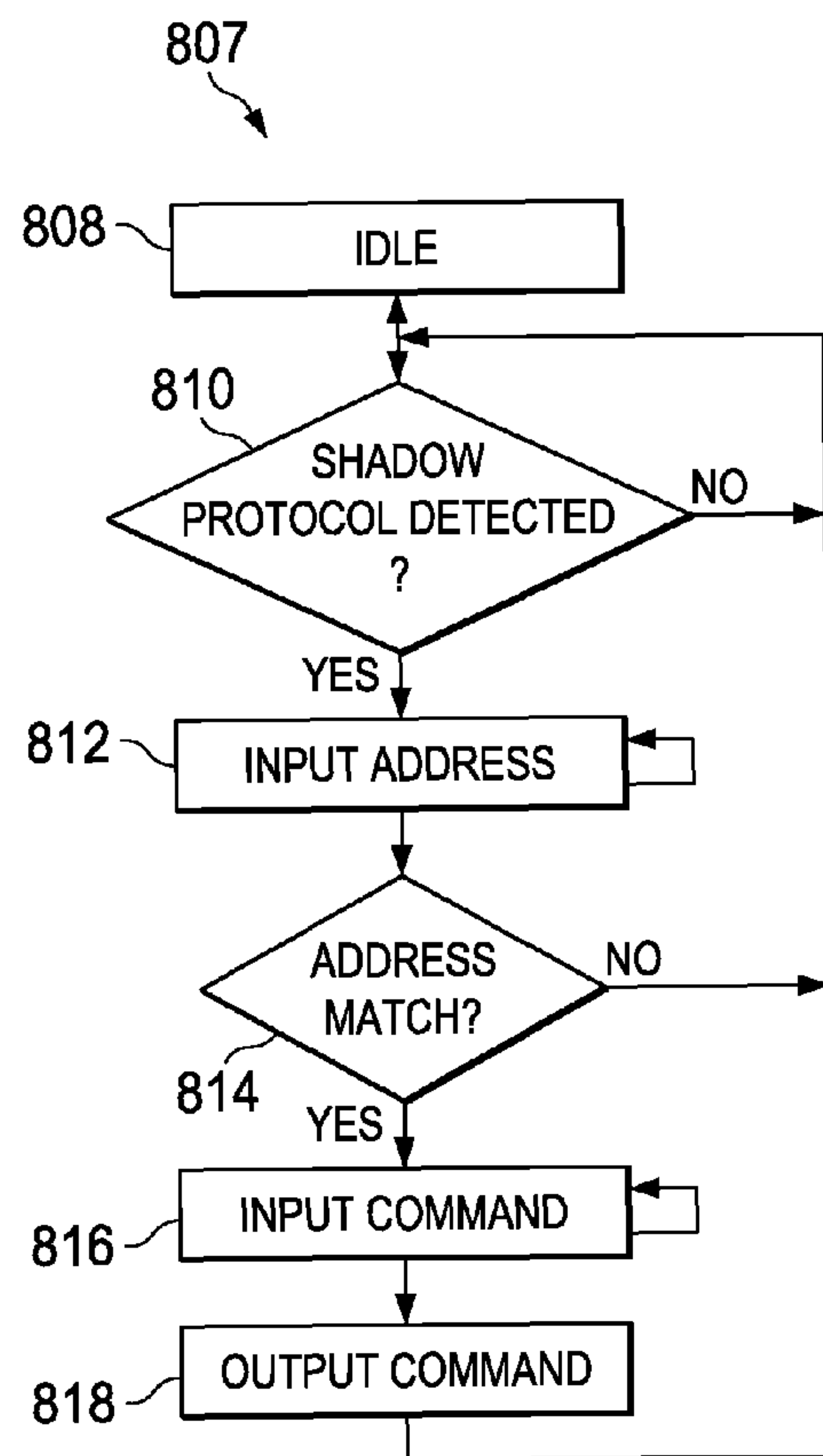
FIG. 8B
