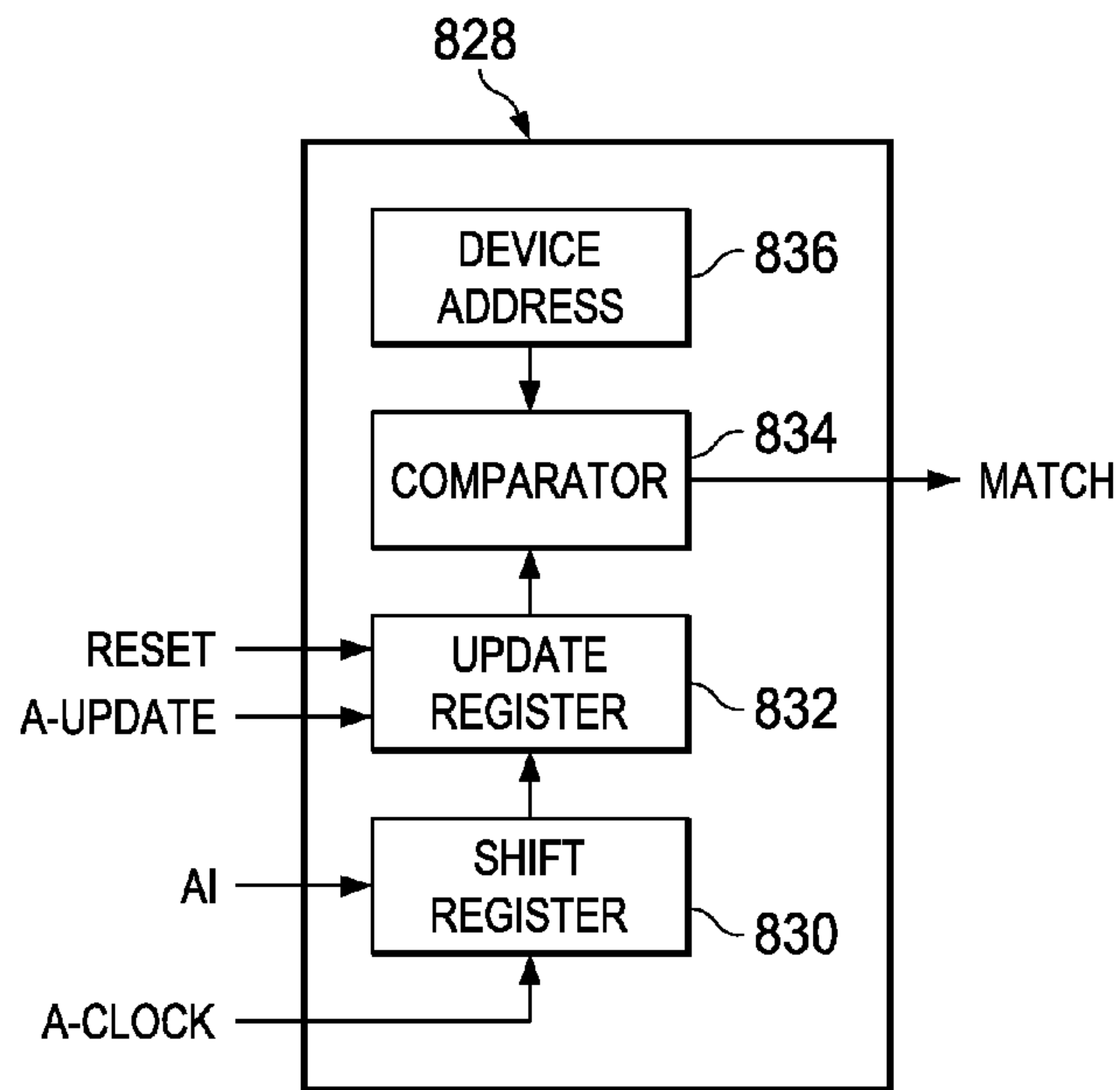
FIG. 8D
