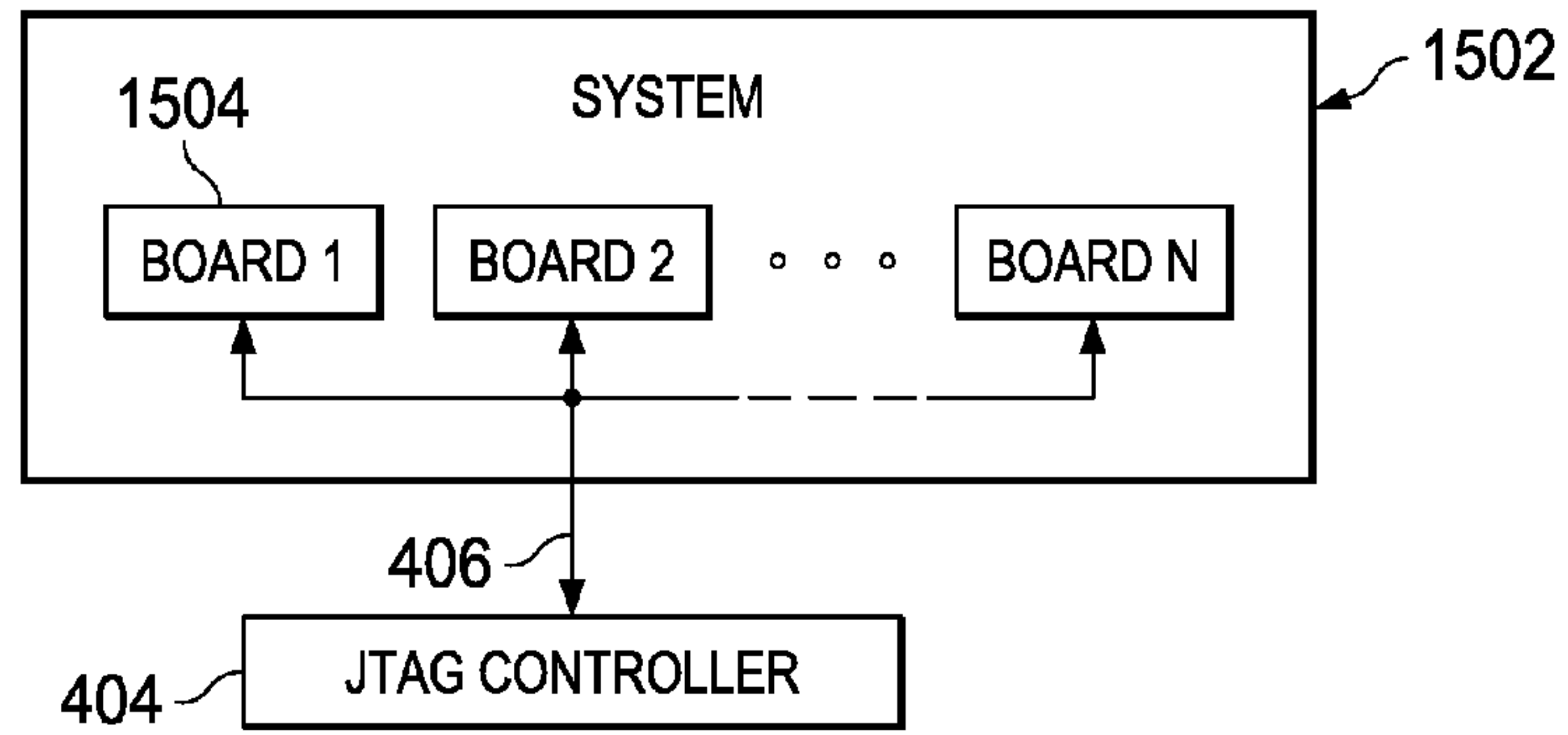
FIG. 15
