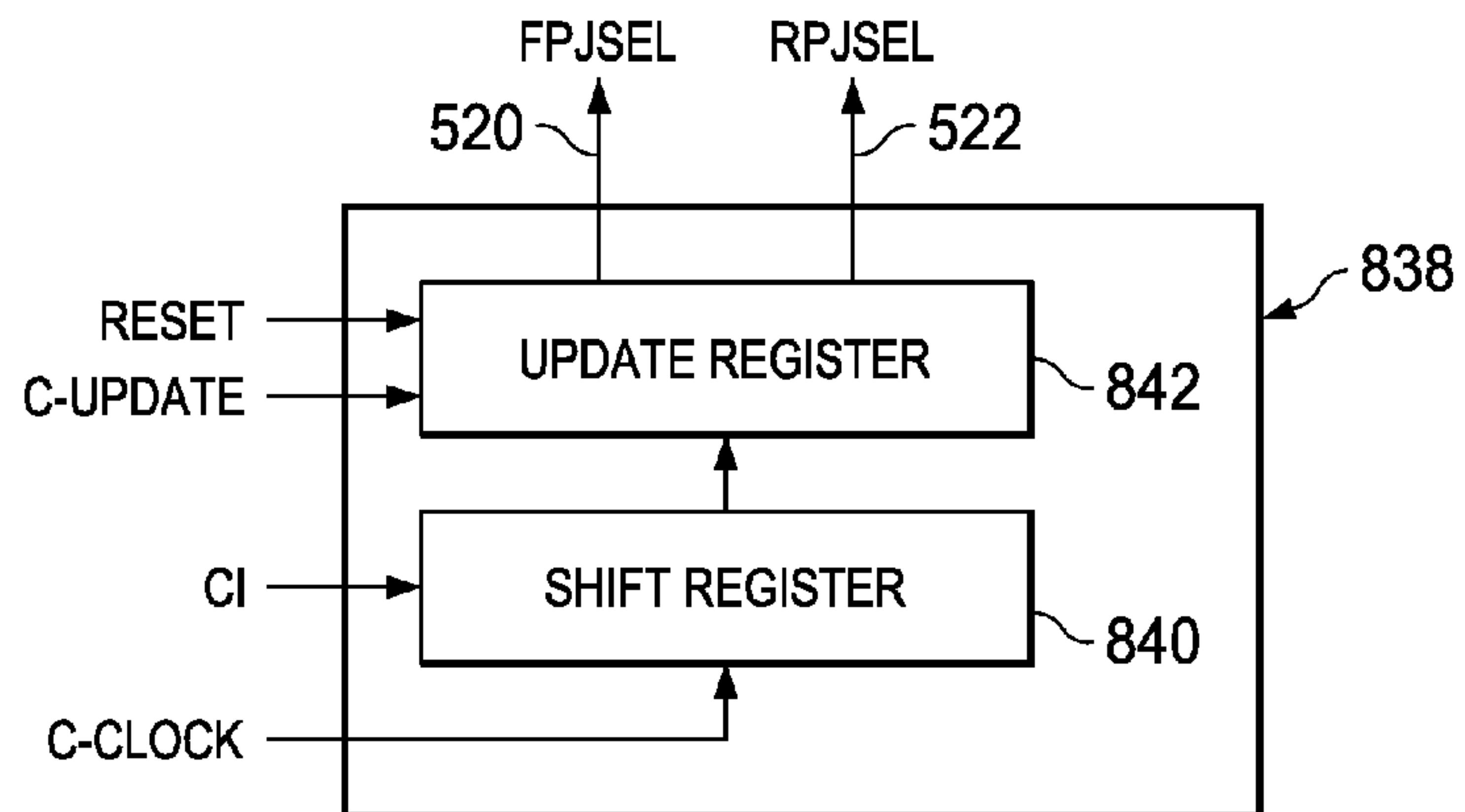
FIG. 8E
