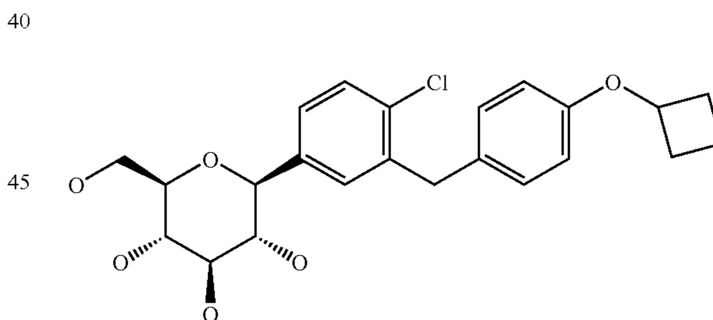
(5) 1-Chloro-4-(β-D-glucopyranos-1-yl)-2-(4-cyclobutyloxy-benzyl)-benzene
