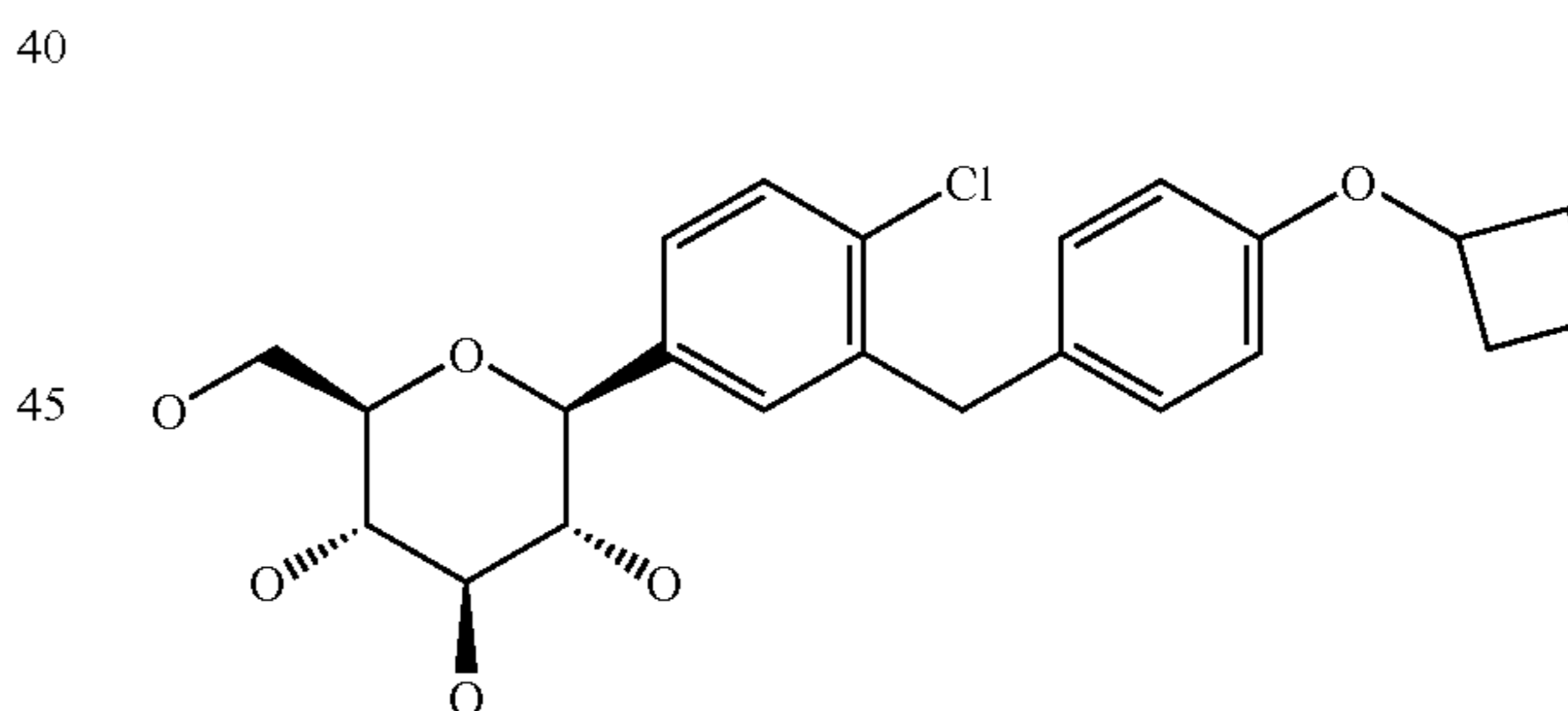
(5) 1-Chloro-4-(β-D-glucopyranos-1-yl)-2-(4-cyclobutyloxy-benzyl)-benzene
